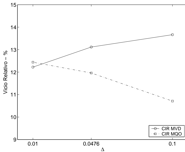
Figura 4.12: Variação do vício relativo em função do \Delta para o modelo CIR, com T = 120 e \kappa = 0,3 .
