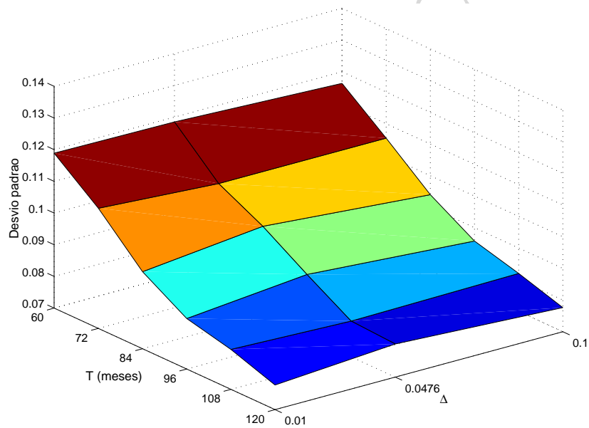
Figura 4.19: Variação do desvio padrão de \hat{\kappa}_{mvd} para o modelo de Vasicek e \kappa = 0,3 .
