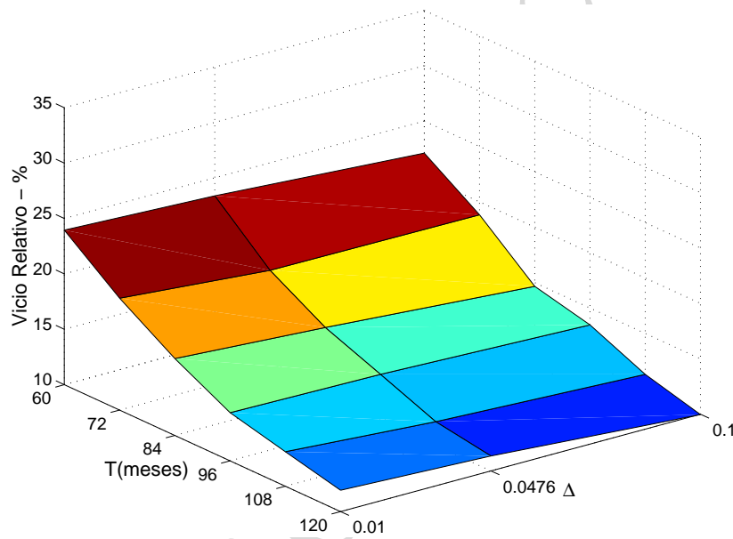
Figura 4.18: Variação do vício relativo de \hat{\kappa}_{mqo} para o modelo de CIR e \kappa = 0, 3 .
