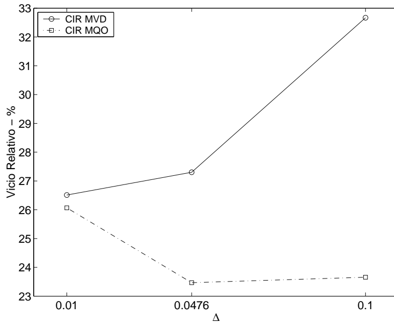
Figura 4.11: Variação do vício relativo em função do \Delta para o modelo CIR, com T = 60 e \kappa = 0,3 .
