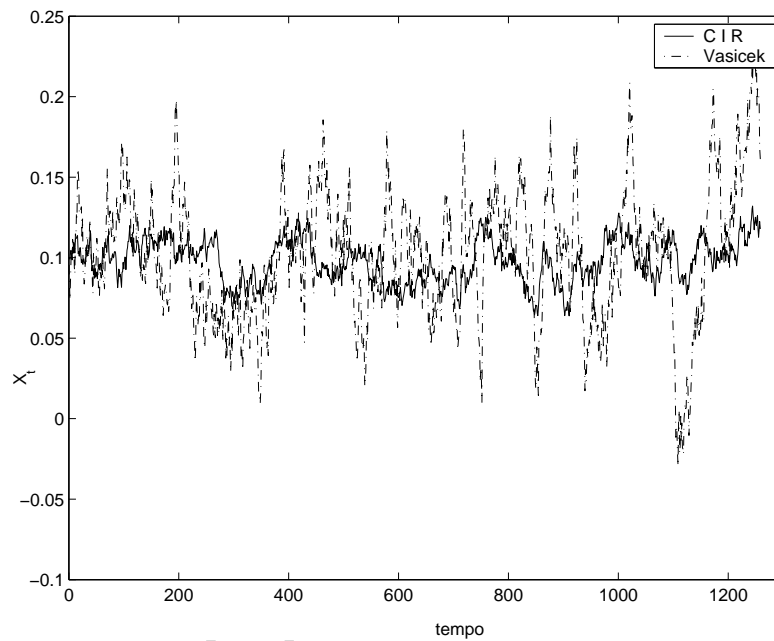
Figura 4.6: Trajetórias simuladas dos modelos CIR e Vasicek \kappa = 0,8 , \nu = 0,1 , \sigma = 0,06 , T = 60 e \Delta = 0,04761 .
