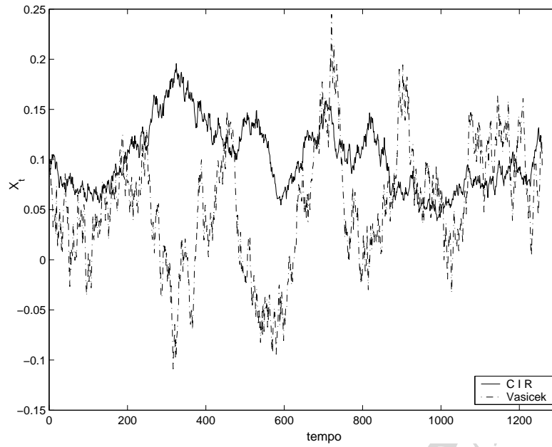
Figura 4.5: Trajetórias simuladas dos modelos CIR e Vasicek \kappa = 0,3 , \nu = 0,1 , \sigma = 0,06 , T = 60 e \Delta = 0,04761 .
