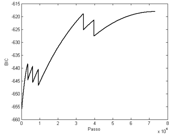
Figura 5.6: Método LASSO - BIC
