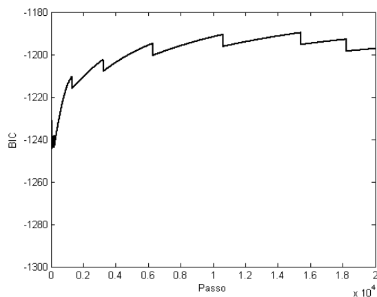
Figura 5.1: Método LASSO - BIC
