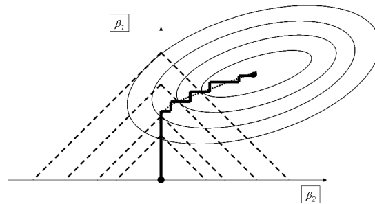
Figura 3.2: Avaliação visual do Método LASSO.
