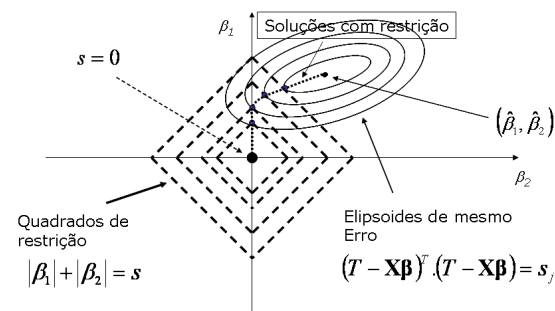
Figura 3.1: Avaliação visual do Método LASSO.
