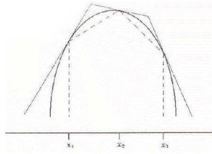
Figura 2.1: Função de Taxa de Falha.
