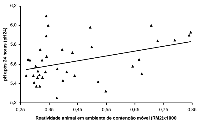
FIGURA 2: Relação funcional entre reatividade animal em ambiente de contenção móvel medida no 84º dia experimental (RM2) e o pH 24 horas post mortem (pH24) em carne de zebuínos (Tabapuã e Nelore) confinados. Linha pontilhada representa valores de pH24 gerados pela equação \text{pH24} = 5,37297 + 0,0005493(\text{RM2}) , com R^2 de 0,22.
