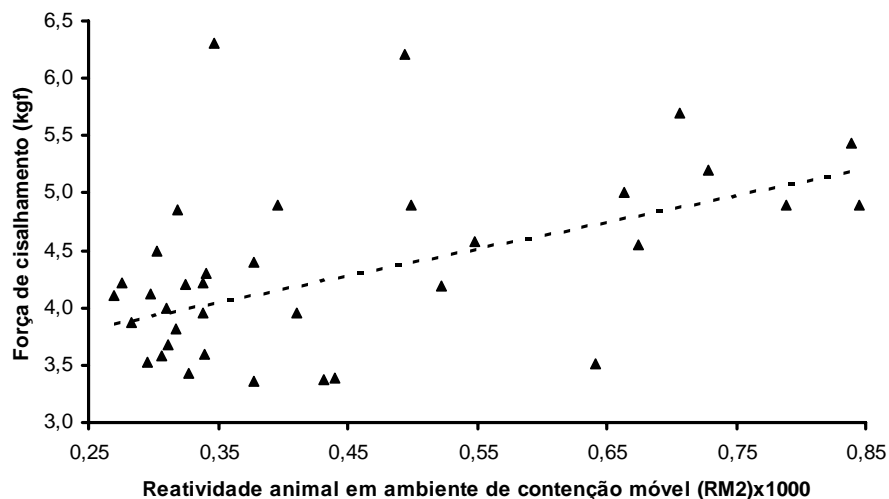
FIGURA 4: Relação funcional entre reatividade animal em ambiente de contenção móvel medida no 84º dia experimental (RM2) e a força de cisalhamento (FC) em carne de zebuínos (Tabapuã e Nelore) confinados. Linha pontilhada representa valores de FC gerados pela equação: FC = 3,2212 + 0,00235(RM2) , com R^2 de 0,22.
