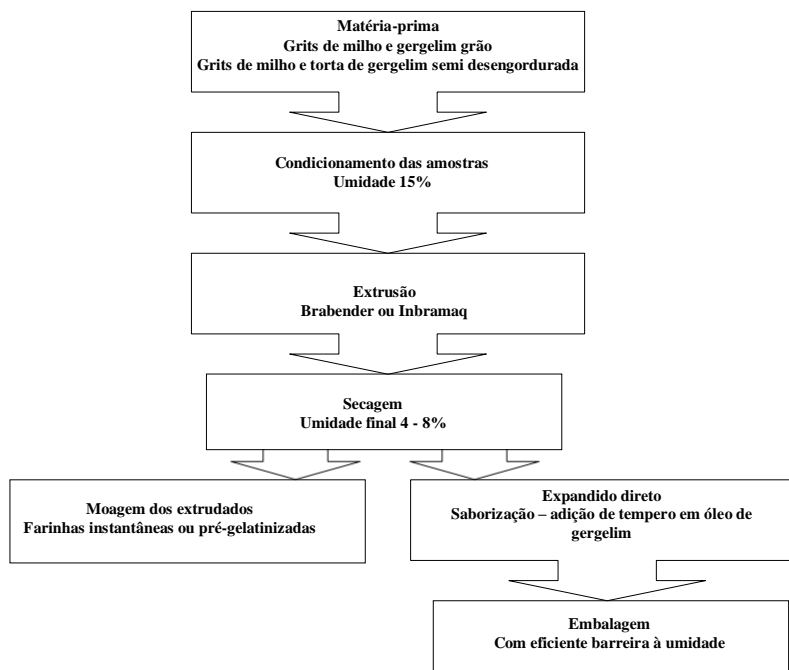
Figura 5 Fluxograma de produção de snacks de expansão direta e farinha instantânea em extrusora Brabender ou Inbramaq.
