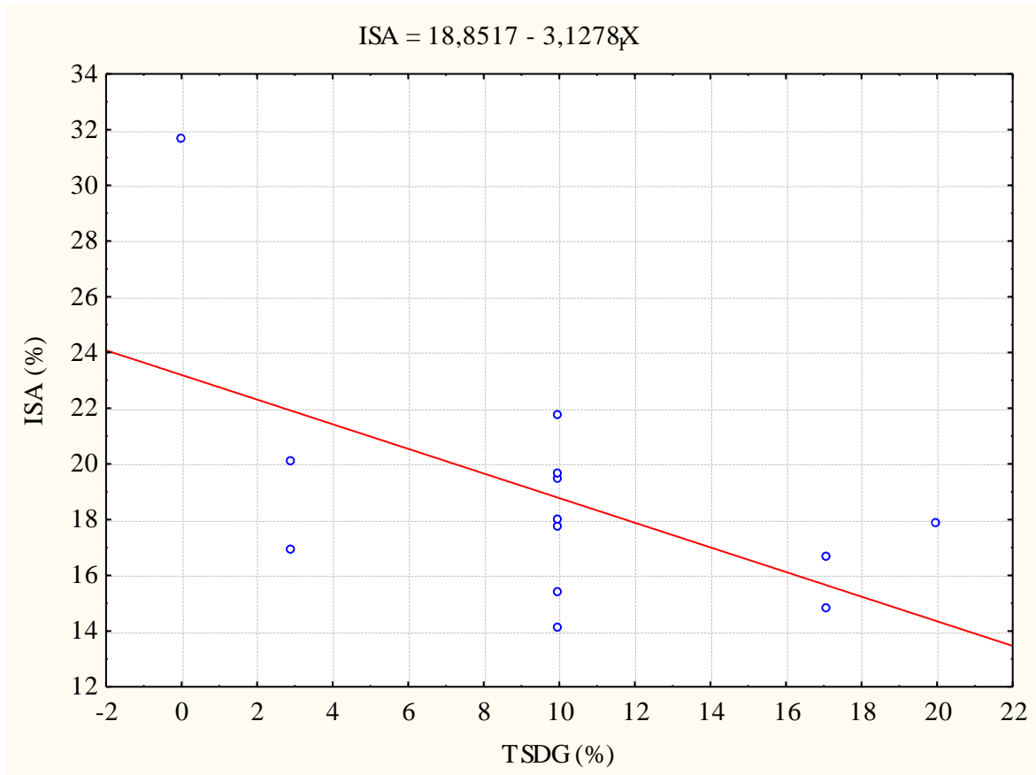
Figura 39 Efeito da adição de torta semi-desengordurada sobre o ISA das farinhas obtidas da moagem dos "snacks".
