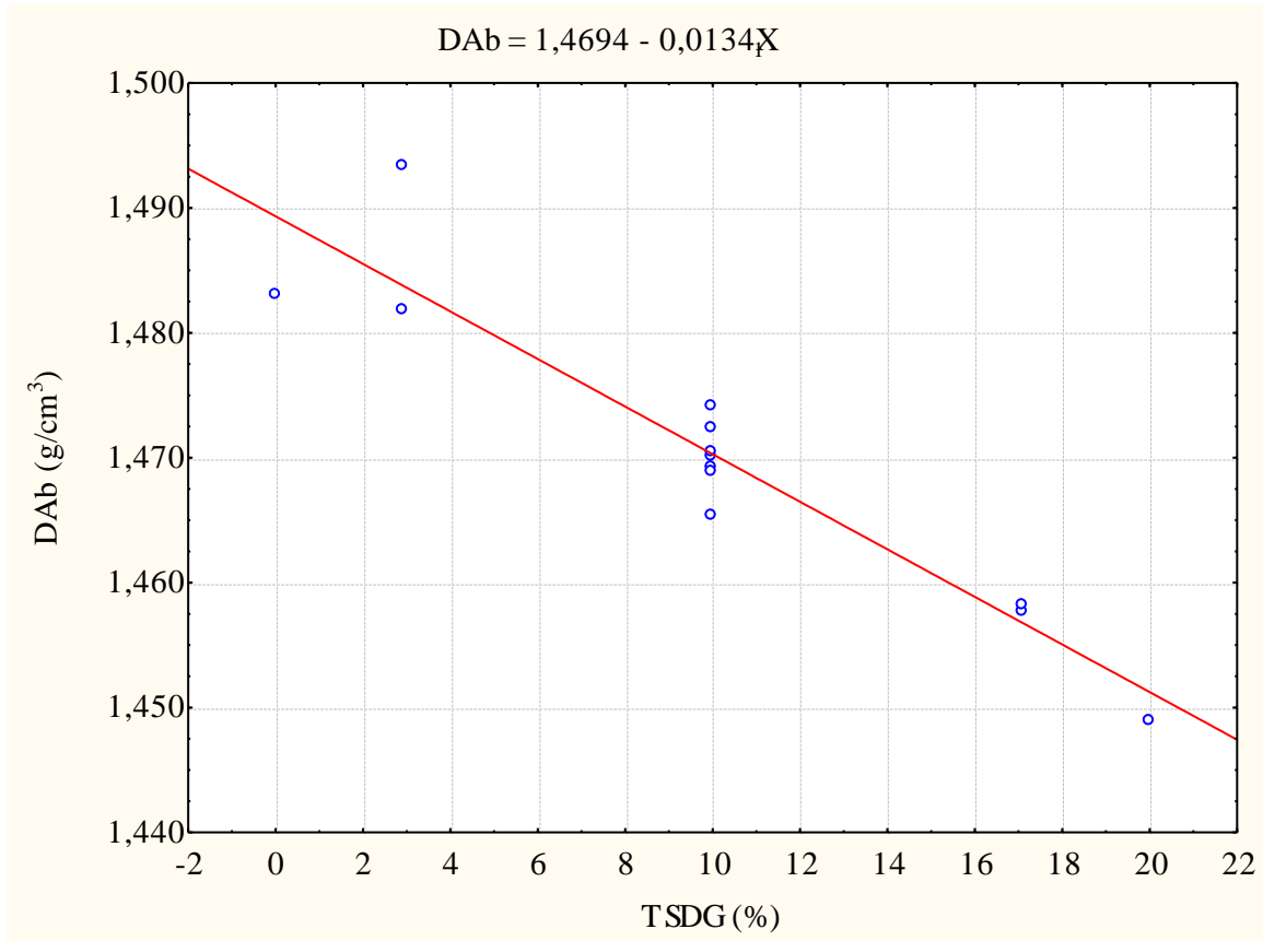
Figura 30 Influência da adição de TSDG em farinha de milho obtido da moagem de extrudados expandidos produzidos em extrusora comercial Inbramaq sobre a DAb das farinhas.
