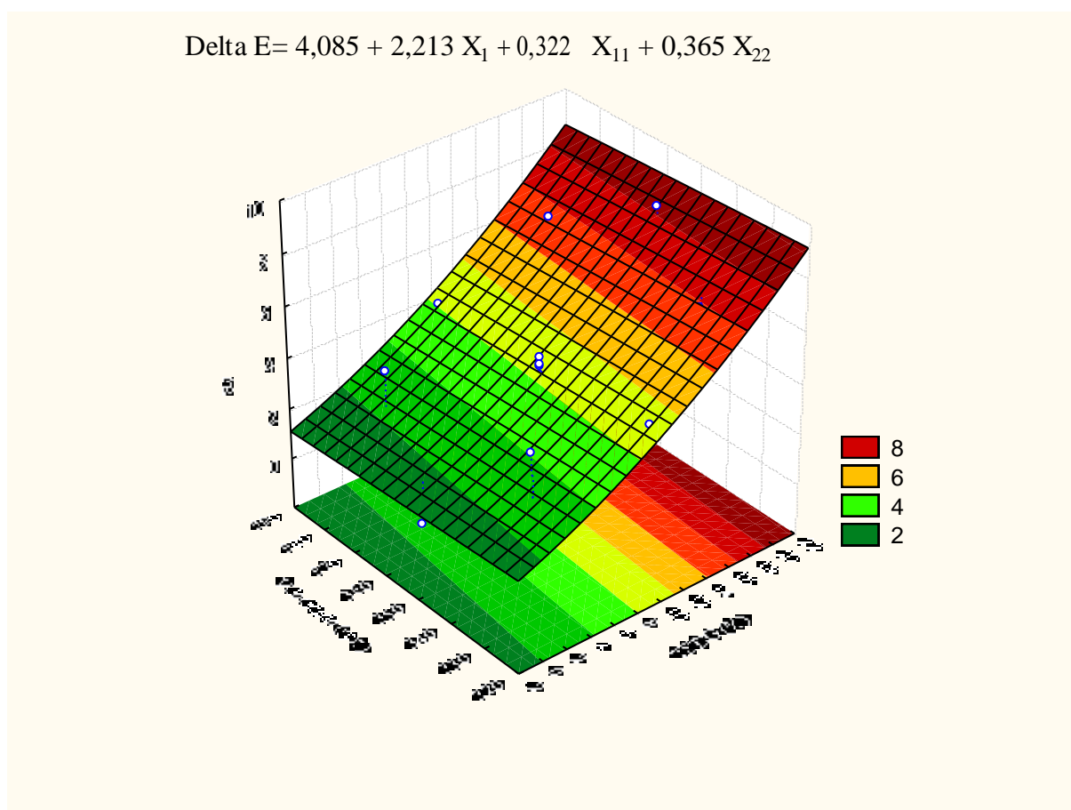
Figura 26 Superfície de resposta para \Delta E dos extrudados elaborados na extrusora comercial Inbramaq.
