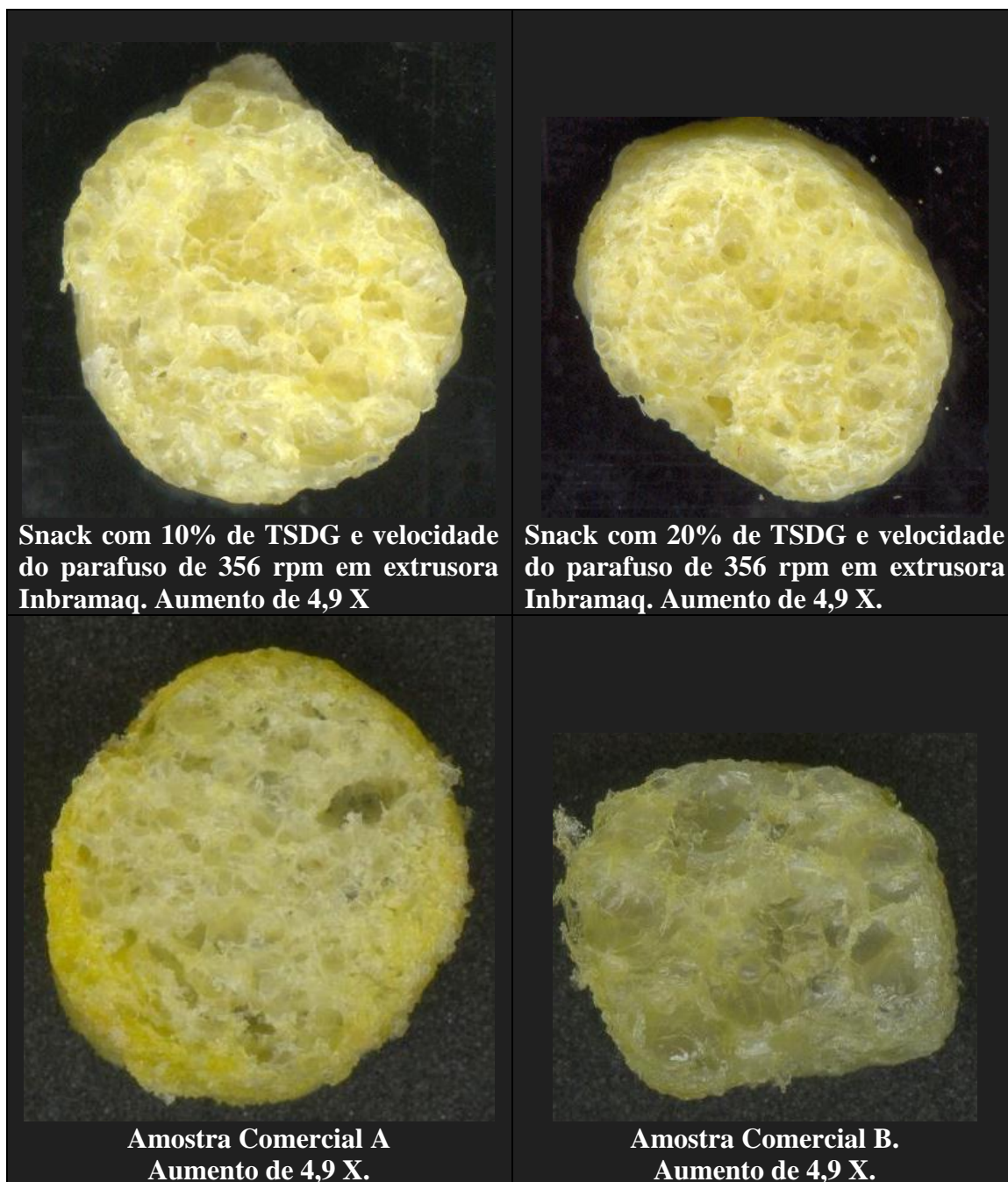
Figura 16 Imagens de expandidos feitas em scanner de escritório. Ao lado esquerdo acima um tratamento central e ao lado direito acima o tratamento axial máximo.
