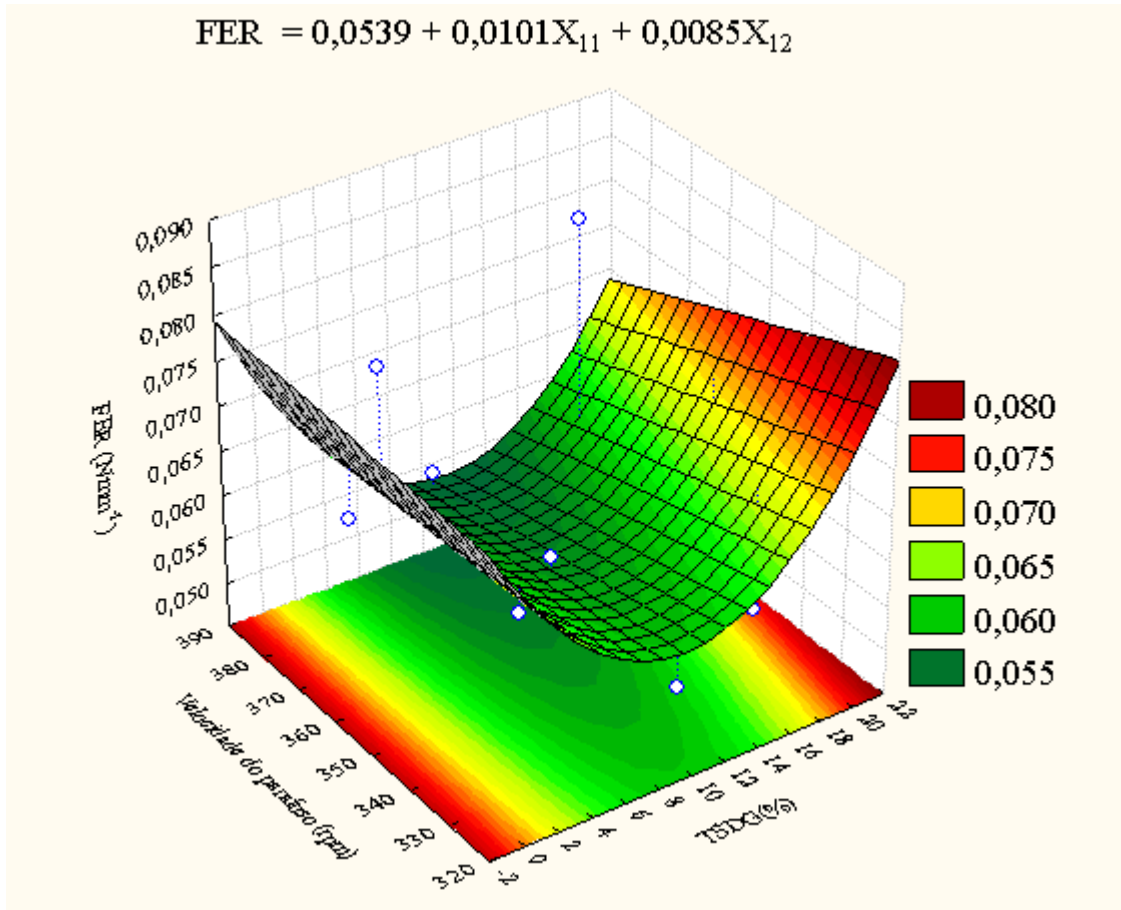
Figura 14 Efeito da velocidade do parafuso e do TSDG sobre a variável resposta Força Específica das Rupturas, FER (N) na extrusora Inbramaq.
