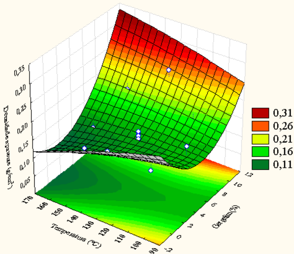
Figura 10 Efeito da temperatura e do teor de gergelim sobre a densidade aparente dos extrudados produzidos na extrusora de laboratório (Brabender).
