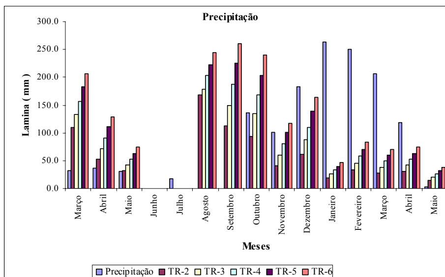
FIGURA 15 Precipitação e lâminas de irrigação aplicadas na área experimental, nos períodos A ( 01/01/08 a 30/03/08), B (01/04 a 15/05 dos anos 07 e 08 ), C ( 01/08/07 a 31/10/07) e D (01/11/07 a 31/12/07).
