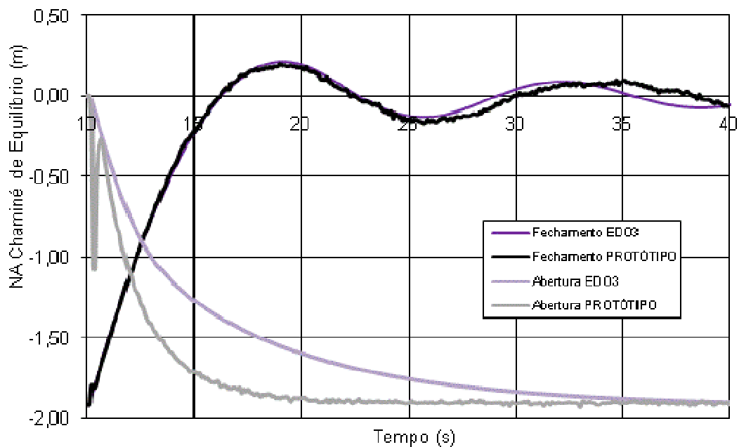
FIGURA 6.5 – Comparação DF-EDOXPROTÓTIPO – Caso Fechamento e Abertura
