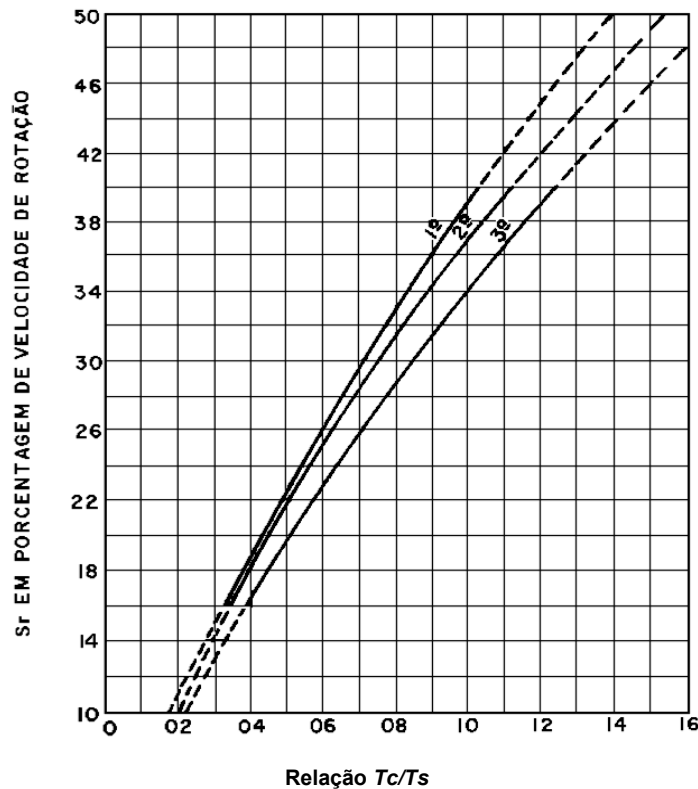
FIGURA 3.5 – Gráfico do Efeito da Sobrepressão do Golpe de Aríete (ELETROBRÁS, 2000).
