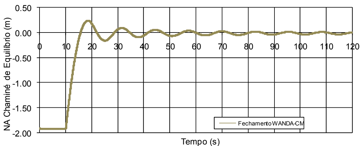
FIGURA 5.9 – Resultado da Simulação WMC-01-CM – Caso Fechamento
