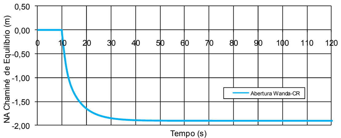
FIGURA 5.8 – Resultado da Simulação WMC-01-CR – Caso Abertura
