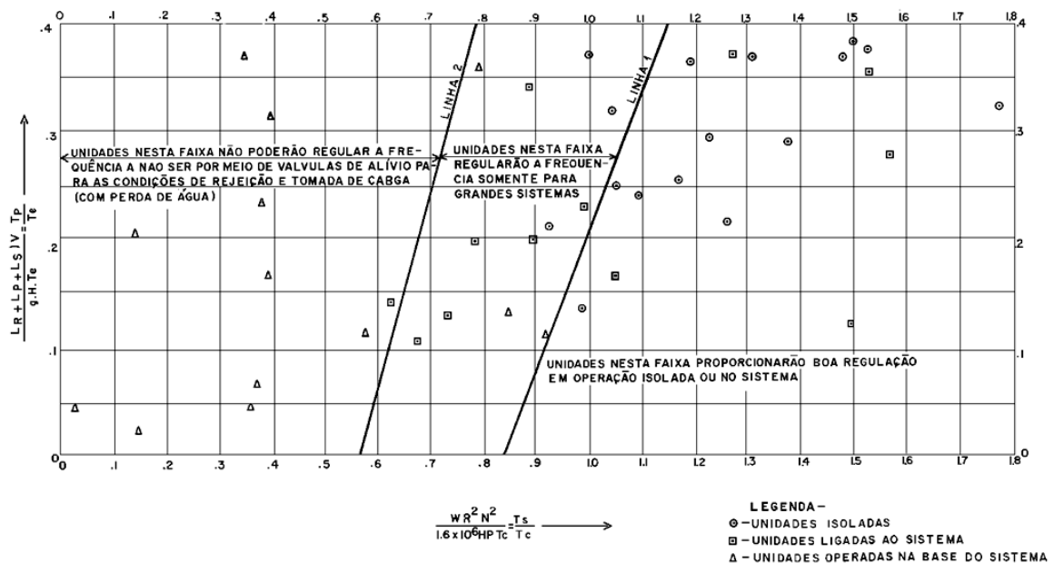
FIGURA 3.6 – Gráfico do Tempo Transitório x Tempo Regulado (ELETROBRÁS, 2000).
