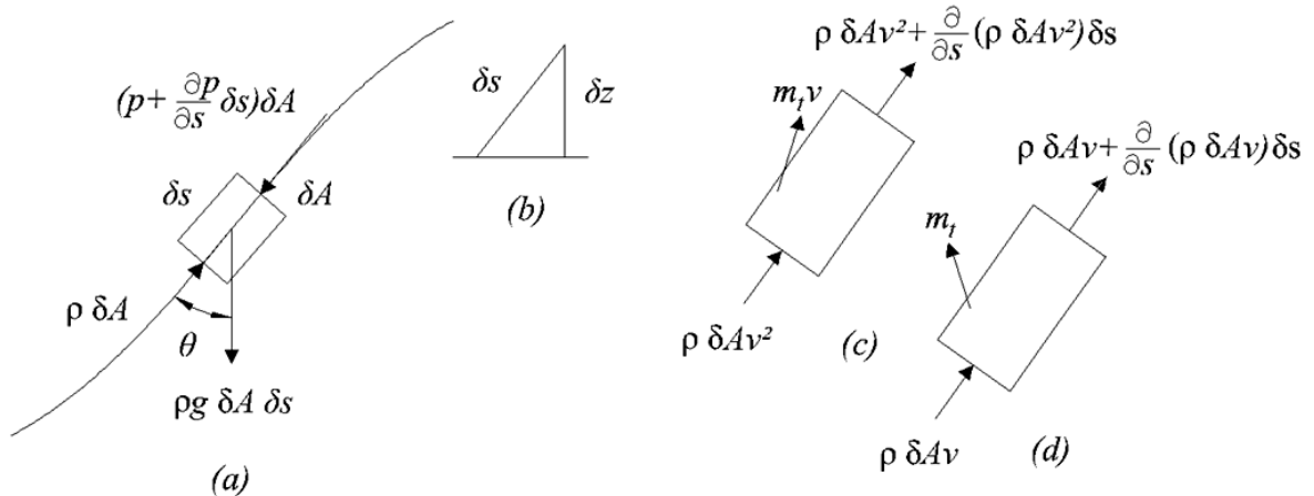
FIGURA 2.10 – Aplicação da Conservação da Quantidade de Movimento para um Escoamento na Direção s Através de um Volume de Controle, (STREETER e WYLIE, 1982).
