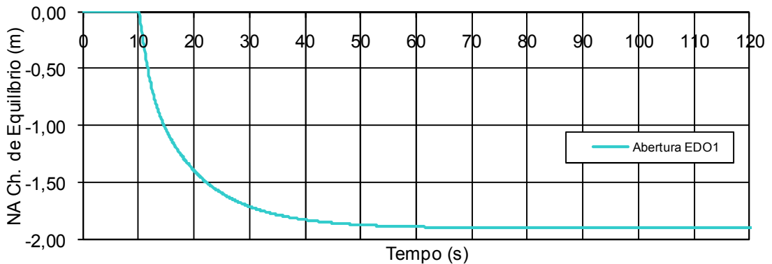
FIGURA 5.3 – Resultado da Simulação EDO1 – Caso Abertura
