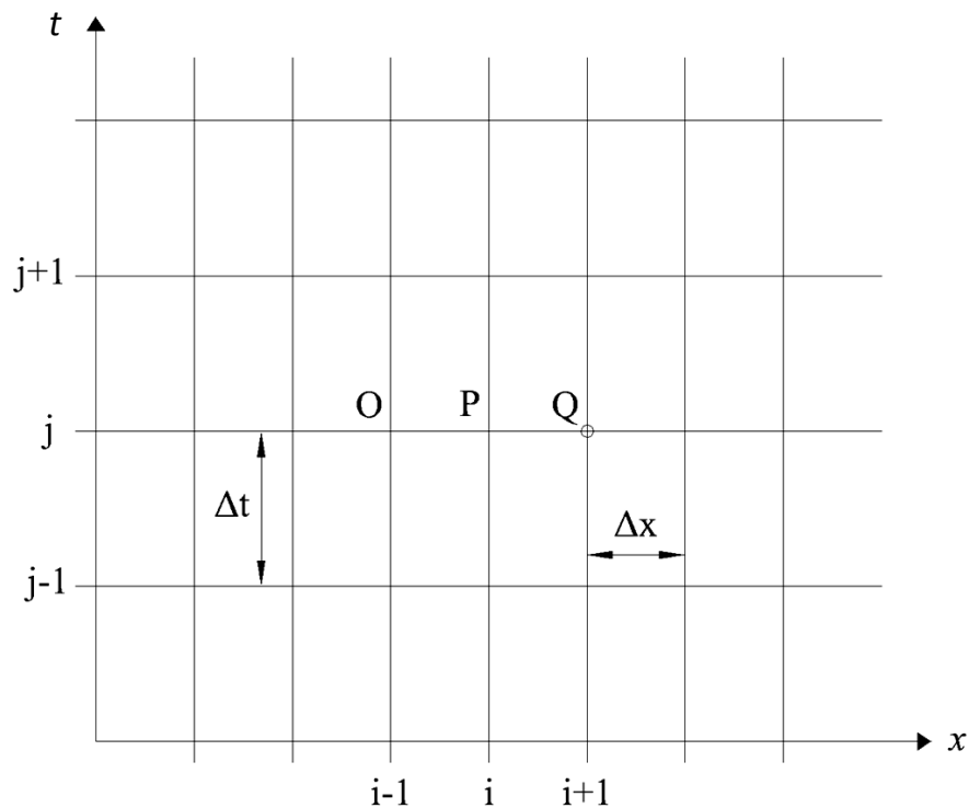
FIGURA 3.3 – Plano de Discretização Explícito (STEINSTRASSER, 2005).
