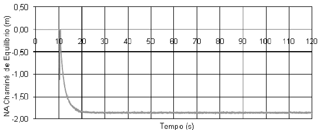
FIGURA 5.15 – Resultado dos Ensaio no Protótipo – Caso Abertura
