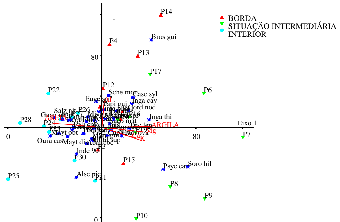
Figura 2 – Expressão gráfica da análise de correspondência canônica (CCA), baseadas na distribuição do número de indivíduos de 22 espécies em 30 parcelas de 10 × 10 m para o dossel (A) e de 39 espécies em 30 parcelas de 5 × 5 m para o sub-bosque (B) na Mata de Zambana em Igarassu, PE, e sua correlação com as variáveis ambientais utilizadas, nos dois primeiros eixos de ordenação.
