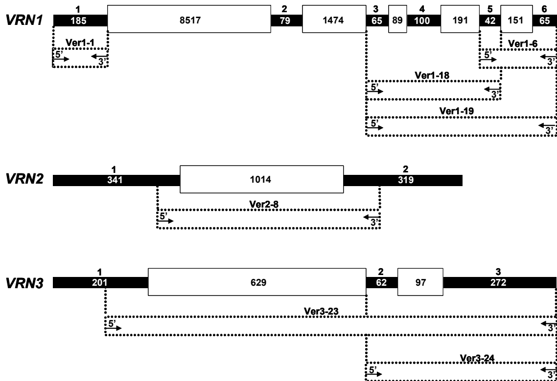
FIGURA 11. Diagrama da sequência consenso para os genes VRN1 , VRN2 e VRN3 . Barras pretas representam éxons e caixas brancas representam íntrons. O número de nucleotídeos (pares de bases) de cada éxon e íntron é apresentado dentro de barras e caixas. A localização de ancoragem dos pares de primers que geraram sequências de aveia associadas aos genes de vernalização está apresentada abaixo da sequência consenso de cada gene em caixas pontilhadas. AAFC-CEF, Ottawa. 2007.
