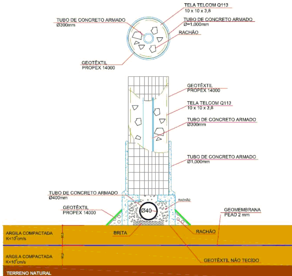
FIGURA 3.3 – SEÇÃO TÍPICA DOS DRENOS VERTICAIS E HORIZONTAIS DE LIXIVIADO FONTE: CONSILIU, 2007
