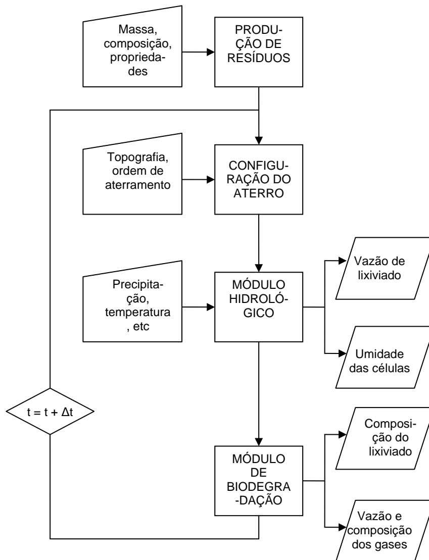
FIGURA 4.1 – ALGORITMO GERAL DO MODELO COMPUTACIONAL MODUELO 2 FONTE: LOBO, 2003a
