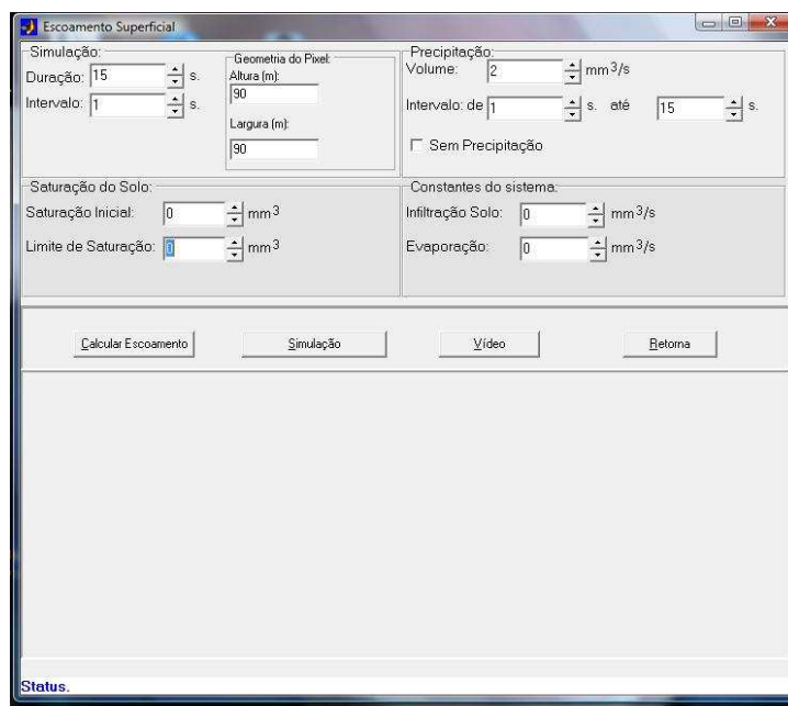
Figura 19: Módulo de controle do sistema.
