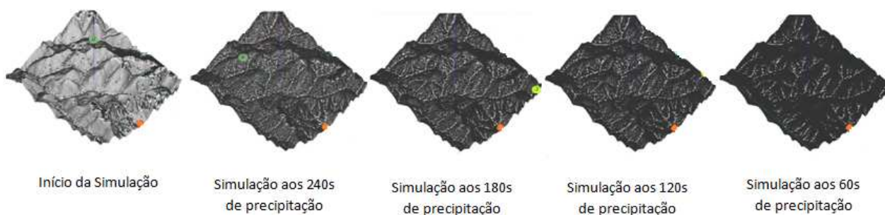
Figura 21: Evolução do Escoamento Superficial: Testes realizados sem considerar as variáveis ambientais
