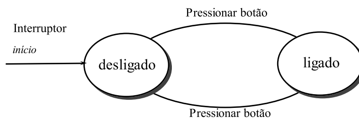
Figura 12: Exemplo de aplicação de um autômato finito.
