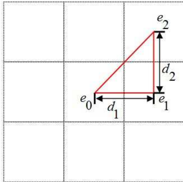
Figura 8: Cálculo da declividade do método Dinfito.
