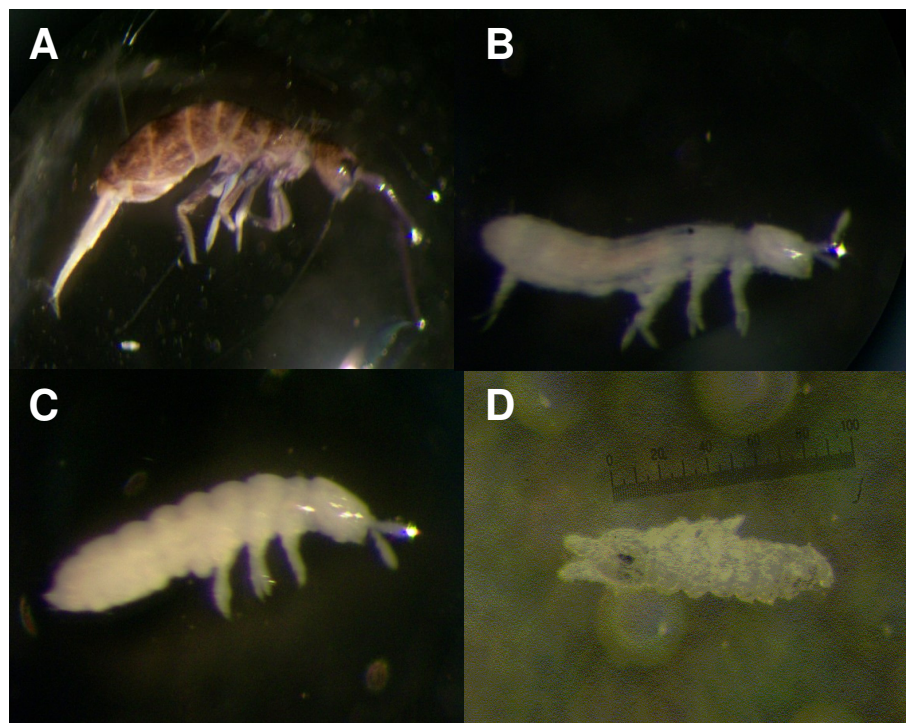
Figura 11: Exemplos de Colembolos (A-D) pertencente às famílias (A) Entomobridae (Agudo- set/2008); (B) Hipogastruridae (Agudo-mar/2008); (C) Onychiuridae (Santa Cruz do Sul - fev/2008) e (D) Poduridae (Agudo - mar/2008).
