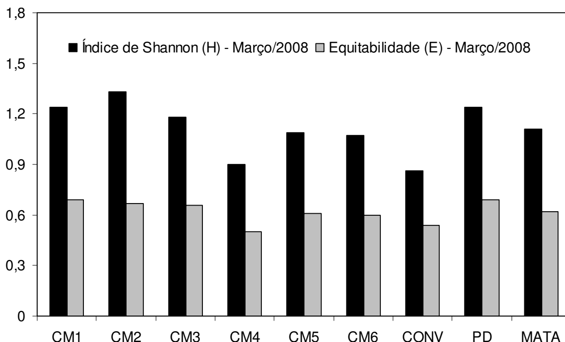
Figura 14: Índices de Shannon (H) e de Equitabilidade (E) em sistemas de manejo do solo e de culturas em Arvorezinha na presença das culturas de verão (março/2008).
