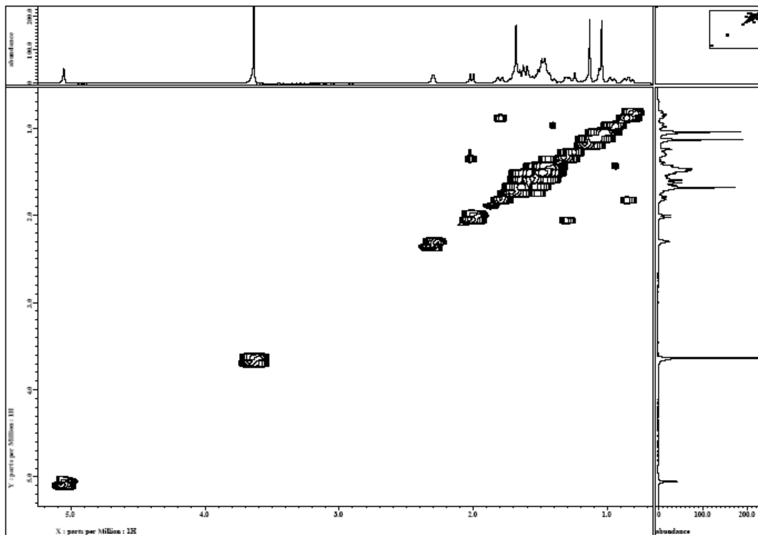
FIGURA 45A – Espectro de COSY (400 MHz, CDCl 3 ) do caur-15-en-18-ato de metila ( 38 ).
