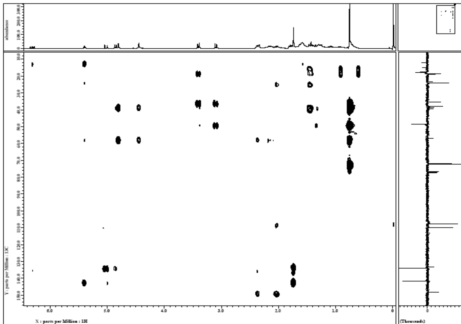
FIGURA 59A – Espectro de HMBC ( ^1\text{H} -400 MHz, ^{13}\text{C} -100 MHz, \text{CDCl}_3 ) do álcool do ozato de metila ( 40 ).
