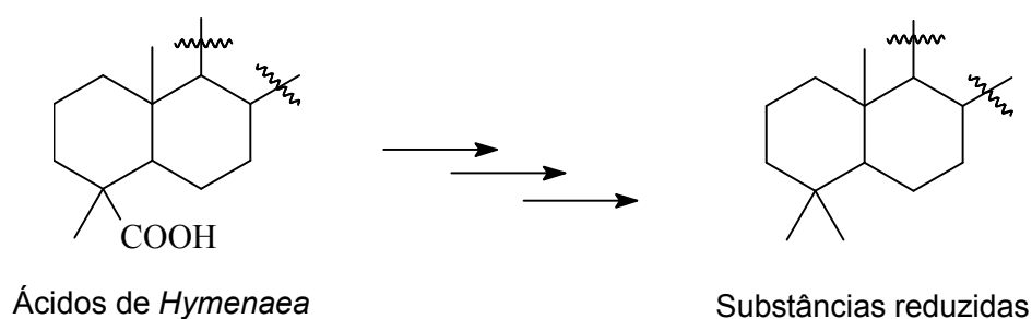
Figura 17 - Redução da posição neo -pentílica.
