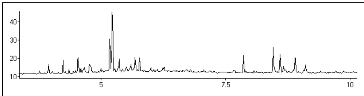
Figura 10 - Cromatograma da fração de neutros do extrato hexânico do epicarpo de H. stigonocarpa .
