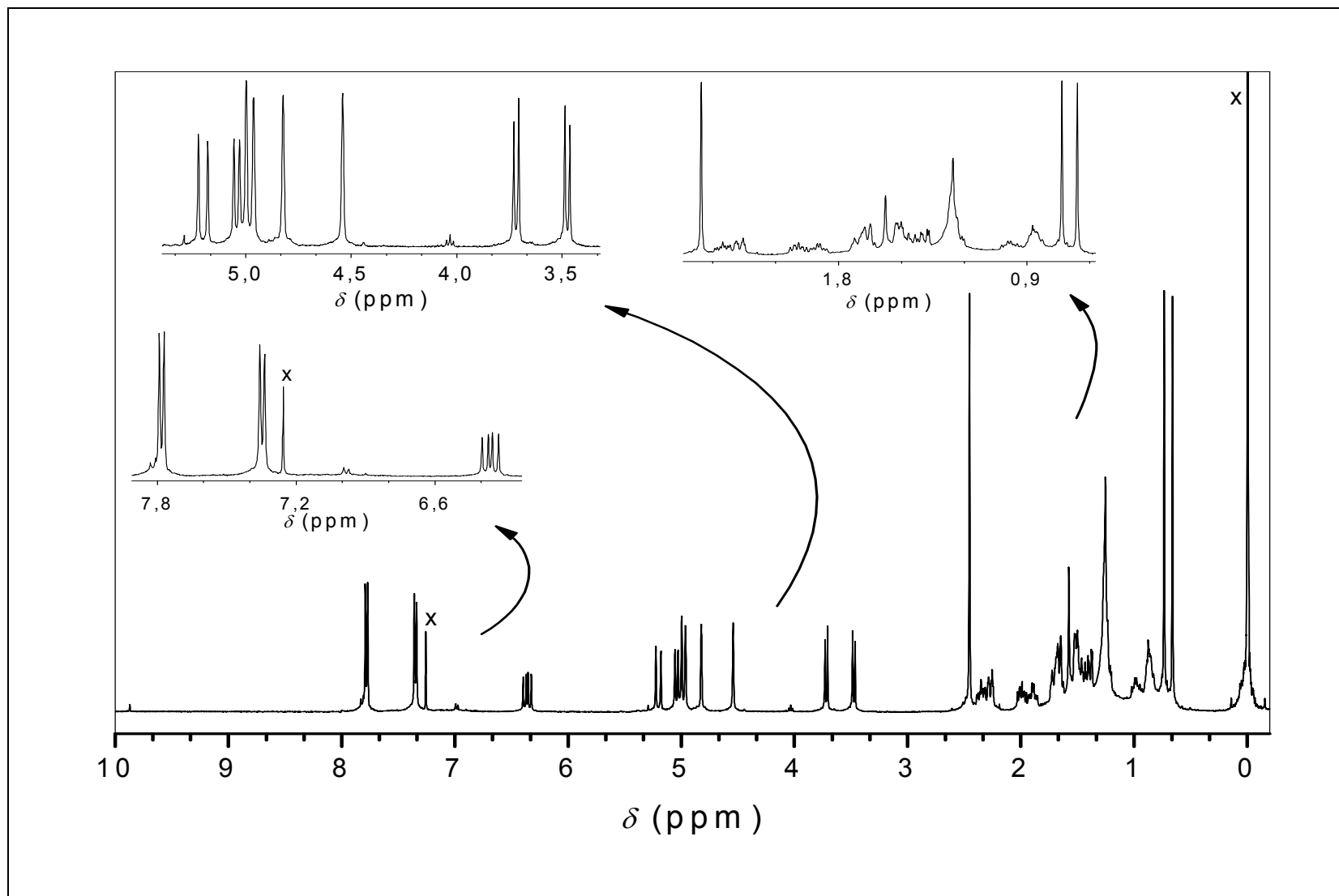
FIGURA 68A – Espectro de RMN de ^1\text{H} (400 MHz, \text{CDCl}_3 ) do tosilato do isoozato de metila (43).
