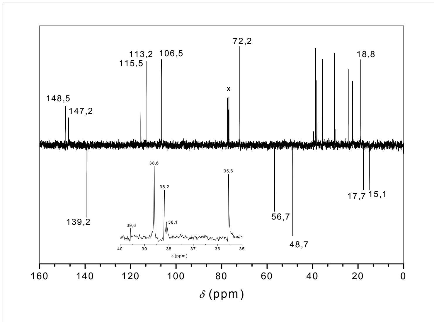
FIGURA 62A - Espectro de RMN de ^{13}\text{C} obtido pela técnica APT (100 MHz, \text{CDCl}_3 ) do álcool do isoozato de metila ( 41 ).
