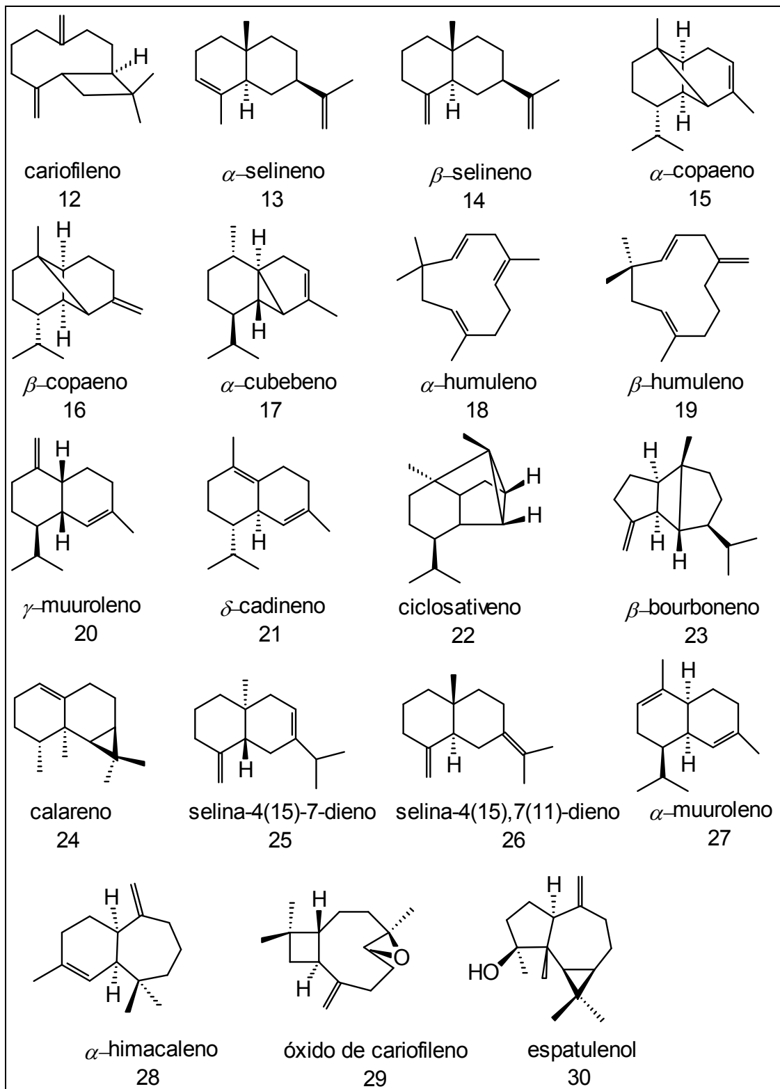
Figura 8 – Sesquiterpenos isolados de Hymenaea .
