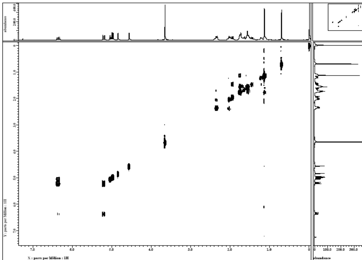
FIGURA 51A – Espectro de COSY (400 MHz, CDCl 3 ) do isoozato de metila ( 39 ).
