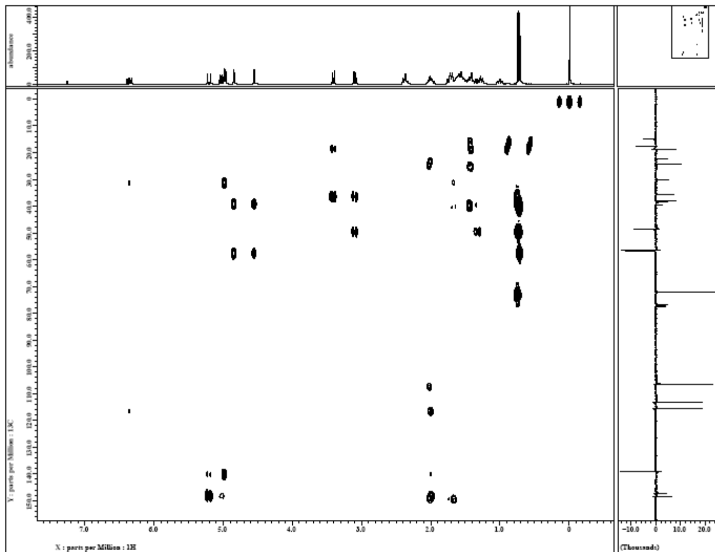
FIGURA 65A – Espectro de HMBC ( ^1\text{H} -400 MHz, ^{13}\text{C} -100 MHz, \text{CDCl}_3 ) do álcool do isooxato de metila ( 41 ).
