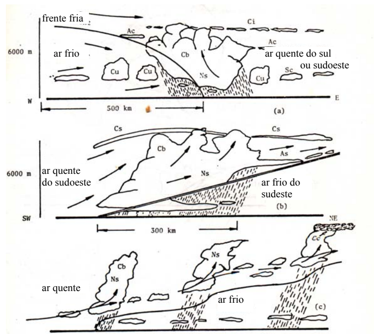
FIGURA 22 – SEÇÕES ESQUEMÁTICAS DE FRENTE DE PRECIPITAÇÃO NO HEMISFÉRIO NORTE, EVIDENCIANDO A GRANDEZA DAS ÁREAS ABRANGIDAS, DA ORDEM DE CENTENAS DE QUILOMETROS (FONTE: RAUDIQUIVI, 1979)
