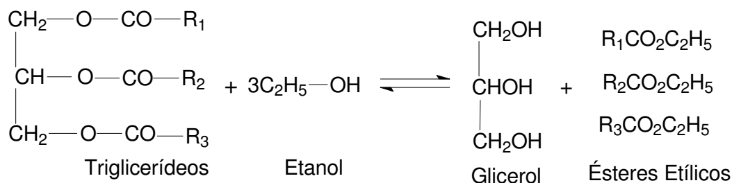
Figura 13 – Reação de transesterificação de triglicerídeos com etanol.
