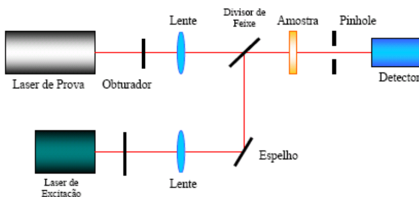
Figura 17 – Configuração para ELT no modo descasado
