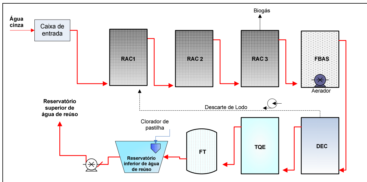
Figura 16: Fluxograma da ETAC
