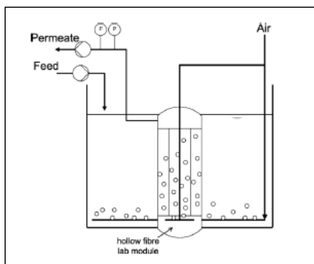
Figura 10: Desenho esquemático do reator MBR Fonte: Merz et al. 2007.
