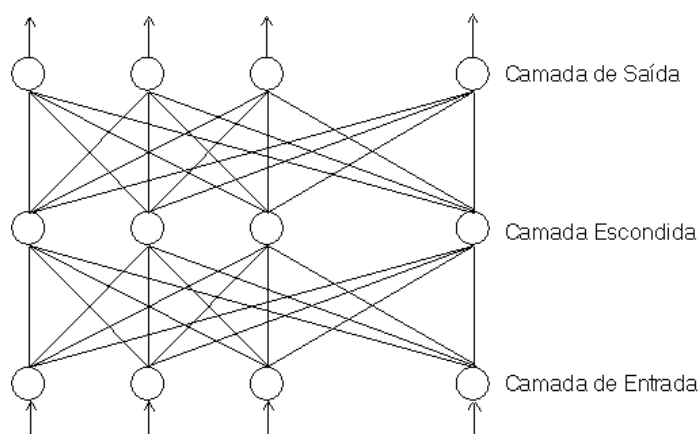
Figura 5 - Estrutura do método Backpropagation Fonte: Tatibana e Kaetsu (2006).
