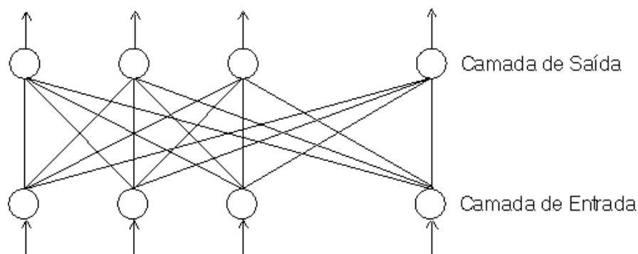
Figura 3 - Rede de Perceptrons proposta por Rosenblatt Fonte: Tatibana e Kaetsu (2006)
