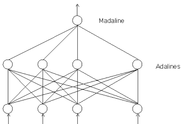
Figura 4 - Redes ADALINE e MADALINE Fonte: Tatibana e Kaetsu (2006)
