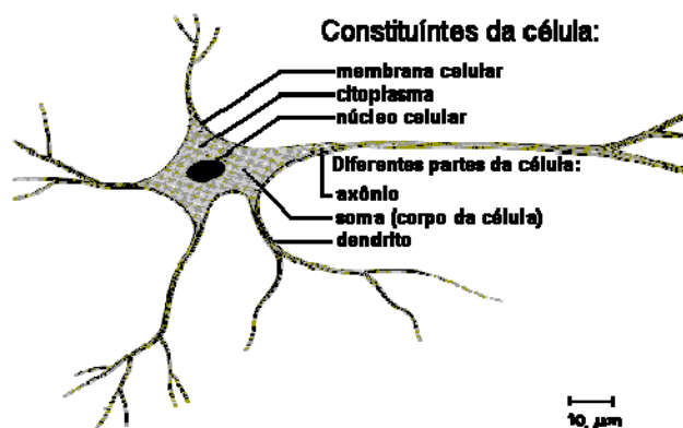
Figura 1 - Esquema dos constituintes da célula neural Fonte: Tatibana e Kaetsu (2006)
