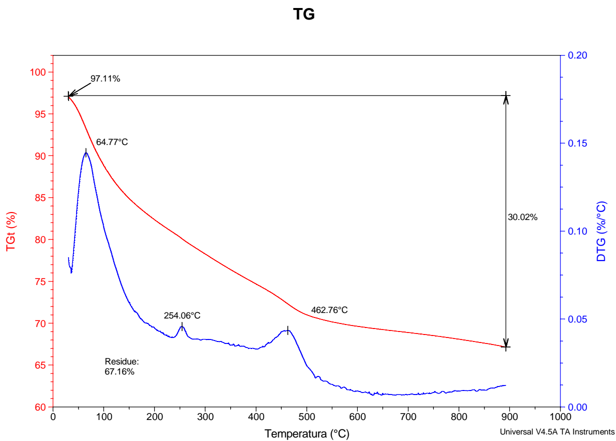
Figura 5.22- Gráfico da 2ª corrida da análise de TG- Lodo 3.
