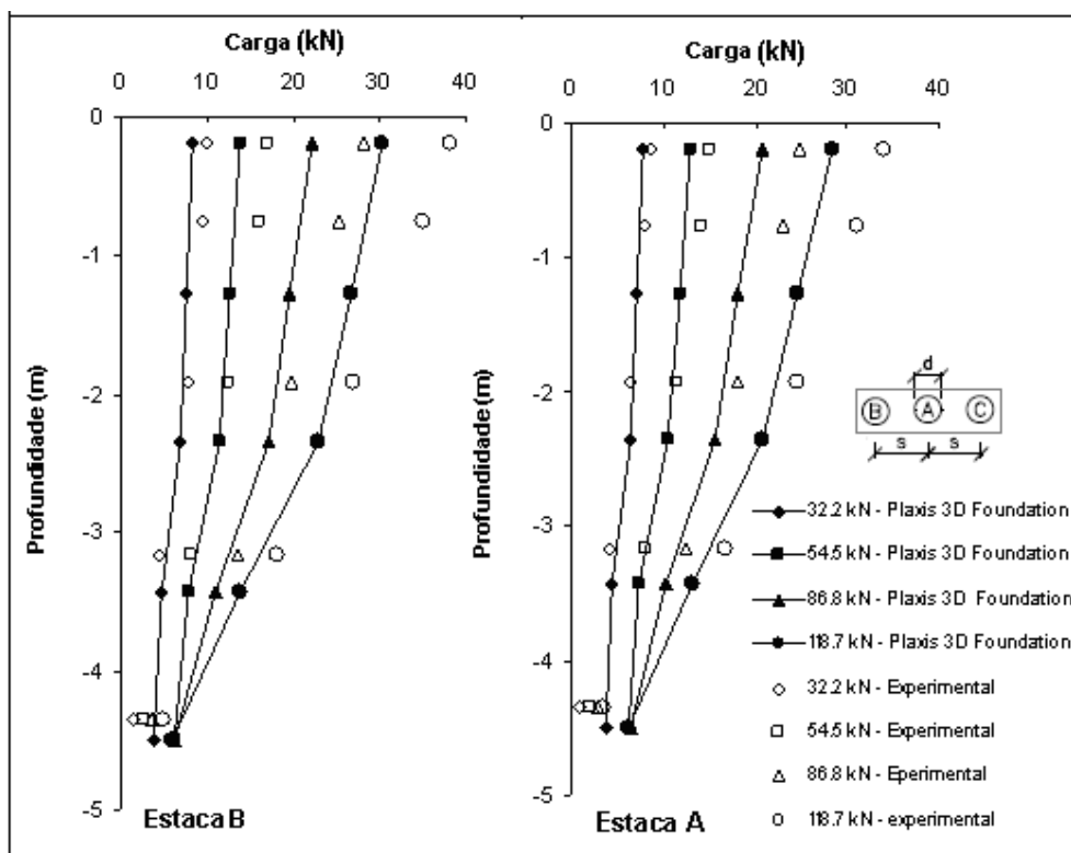
Figura 2.45- Resultados do ensaio 7 – Transferência de carga nas estacas B e A.
