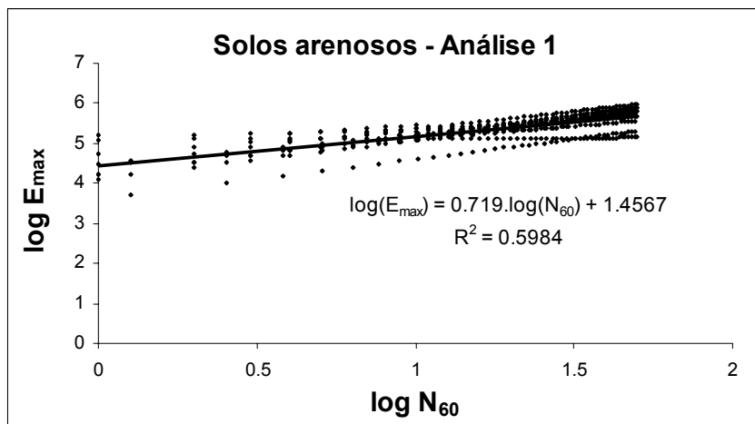
Figura 3.3- Solos arenosos ( \log N_{60} \times \log E_{max} ) - banco de dados completo – análise 1.
