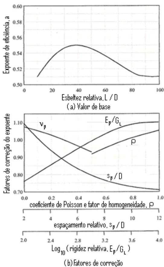
Figura 1.9- Estimativa do fator de eficiência da rigidez para um grupo de estacas carregado verticalmente (adaptado de Fleming et al, 1992).
