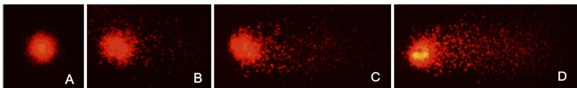
Figura 7: Classes de danos observadas no ensaio do cometa com Oreochromis niloticus expostos a diversas amostras de água coletadas. A. Classe 0: célula sem dano; B. Classe 1: célula com pouco dano; C. Classe 2: célula com médio dano; D. Classe 3: célula com grande dano.
