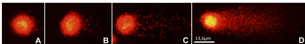
Figura 5: Danos no DNA observados em células de brânquias de Oreochromis niloticus , após a exposição a um biosurfactante ramnolipídico. A. Classe 0; B. Classe 1; C. Classe 2; D. Classe 3 [159].
