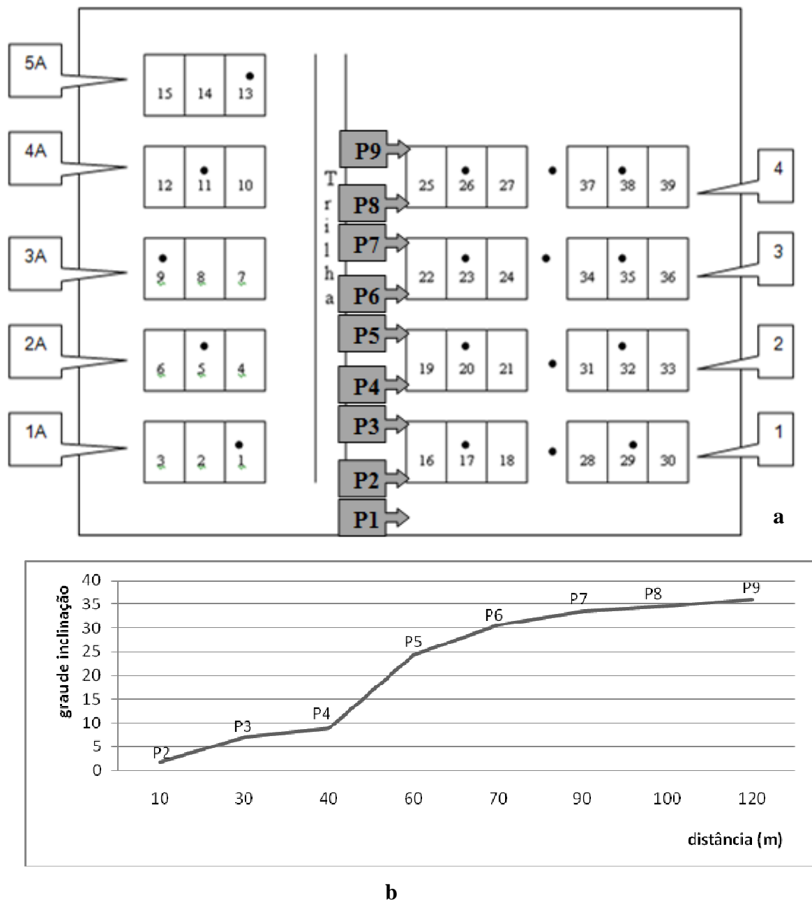
Figura 12. Localização dos pontos de georreferenciamento na área das parcelas (a) e gráfico da Declividade do terreno na mesma área no Parque Prainha, município de Caconde, SP (b). Para os pontos marcados, consultar Tabela 3, a seguir.
