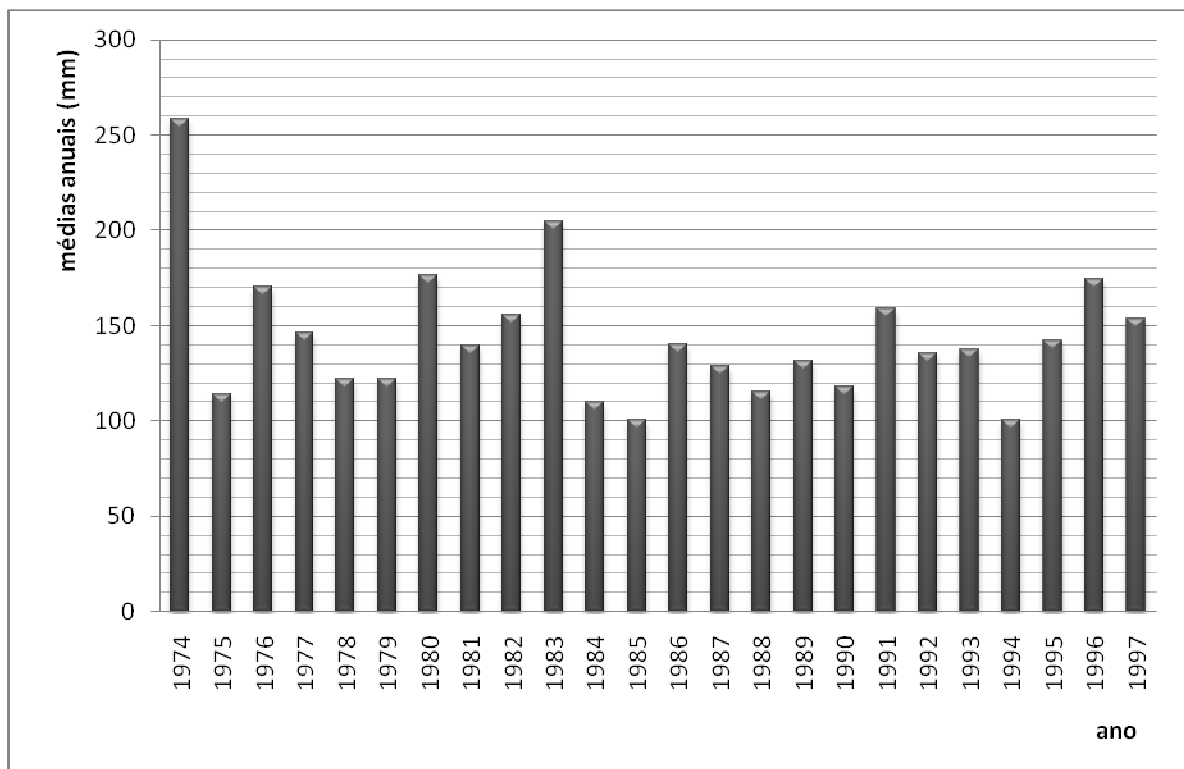
Figura 9. Chuvas anuais num período de 24 anos no município de Caconde, SP (dados: SIGRH, 2008).
