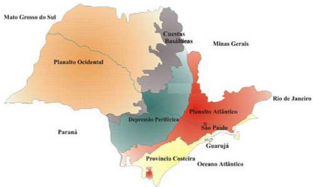
Figura 4. Mapa da divisão geomorfológica do Estado de São Paulo (fonte: SÃO PAULO, 2009, modificado)
