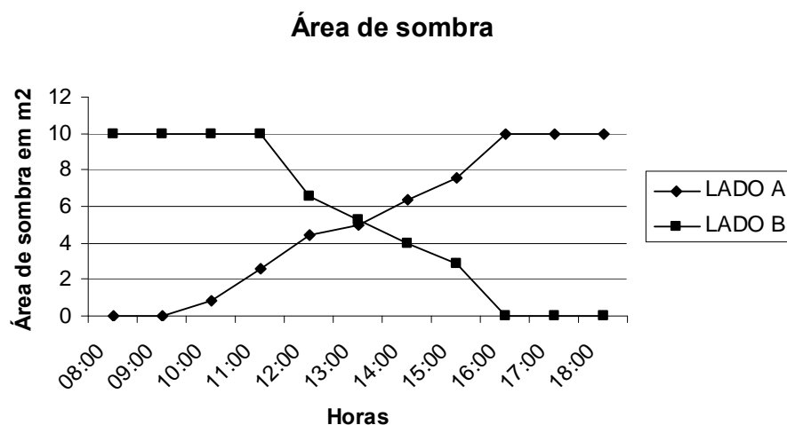
Figura 3 – Representação gráfica da área de sombra ao longo do dia nos diferentes lados do confinamento.
