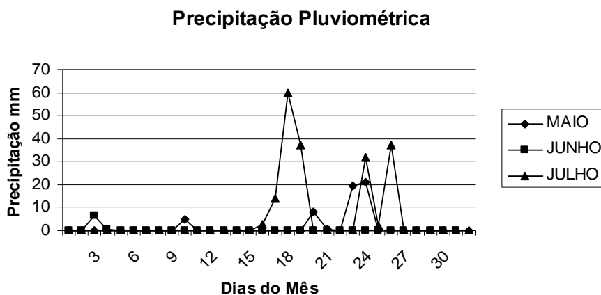
Figura 2 – Representação gráfica da precipitação pluviométrica nos dias de coletas de dados.
