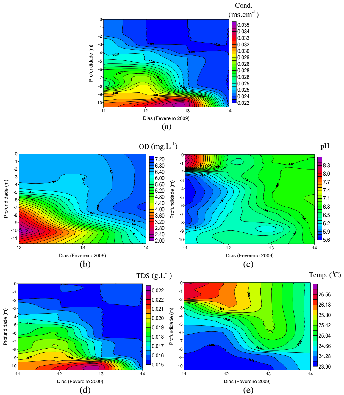
Figura 11: Perfil vertical da coluna de água de variáveis física e químicas nos dias 11, 12, 13 e 14/02/09. (a) Condutividade ( \text{ms.cm}^{-1} ); (b) oxigênio dissolvido ( \text{mg.L}^{-1} ); (c) pH; (d) sólidos totais dissolvidos ( \text{g.L}^{-1} ) e (e) temperatura ( ^{\circ}\text{C} ).
