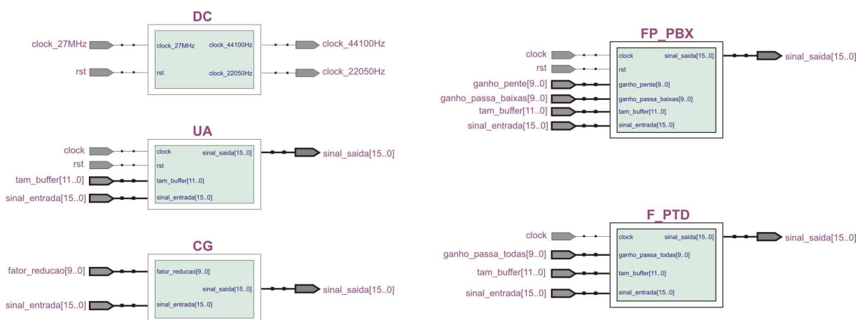
Figura 4.1 - Diagrama de blocos do conjunto de módulos básicos.
