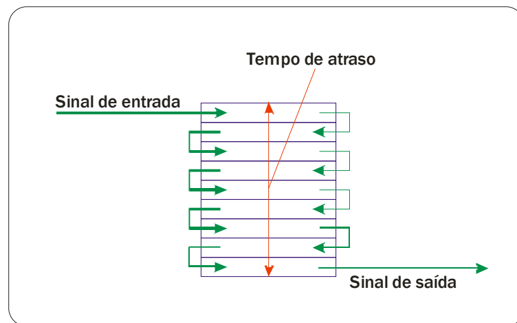
Figura 4.3 – Unidade de atraso implementada através de uma FIFO.
