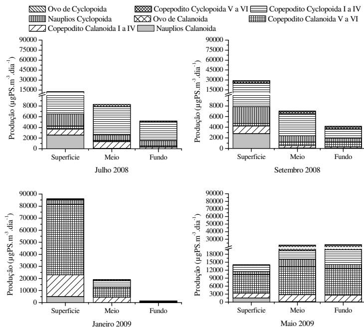
Figura 84. Valores de produção ( \mu\text{g PS} \cdot \text{m}^{-3} \cdot \text{dia}^{-1} ) dos Copepoda no reservatório no reservatório de Nova Avanhandava nas camadas de superfície, meio e fundo da coluna d'água nos meses de julho e setembro de 2008 e janeiro e maio de 2009.
