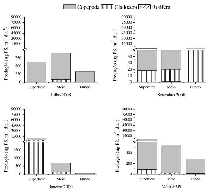
Figura 91. Valores de produção ( \mu\text{g PS. m}^{-3} \cdot \text{dia}^{-1} ) da comunidade zooplancônica no reservatório de Três Irmãos nas camadas de superfície, meio e fundo da coluna d'água nos meses de julho e setembro de 2008 e janeiro e maio de 2009.
