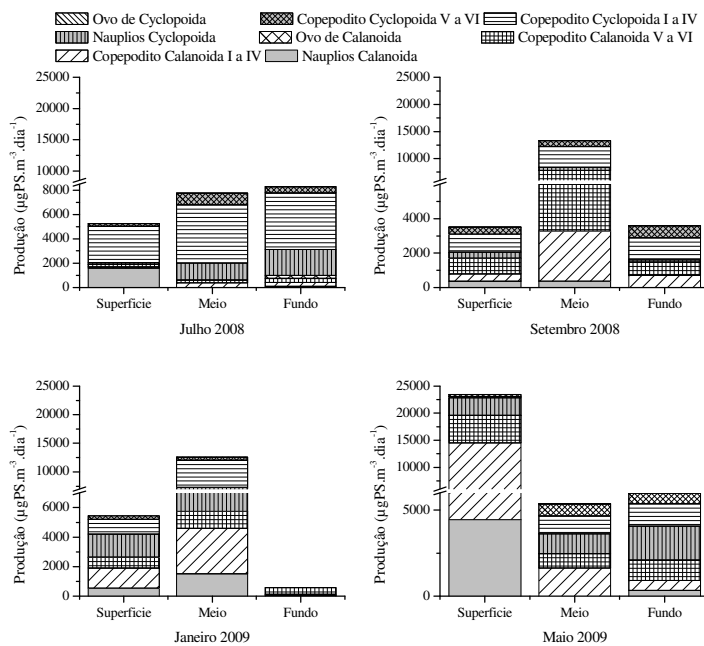
Figura 83. Valores de produção ( \mu\text{g PS} \cdot \text{m}^{-3} \cdot \text{dia}^{-1} ) dos Copepoda no reservatório no reservatório de Promissão nas camadas de superfície, meio e fundo da coluna d'água nos meses de julho e setembro de 2008 e janeiro e maio de 2009.
