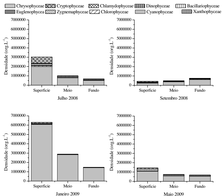
Figura 48. Densidade (org.L -1 ) das classes fitoplânctônicas no reservatório de Nova Avanhandava nas camadas de superfície, meio e fundo da coluna d'água nos meses de julho e setembro de 2008 e janeiro e maio de 2009.
