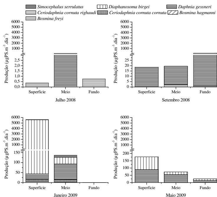
Figura 82. Valores da produção ( \mu\text{gPS}\cdot\text{m}^{-3}\cdot\text{dia}^{-1} ) dos Cladocera no reservatório no reservatório de Três Irmãos nas camadas de superfície, meio e fundo da coluna d'água nos meses de julho e setembro de 2008 e janeiro e maio de 2009.
