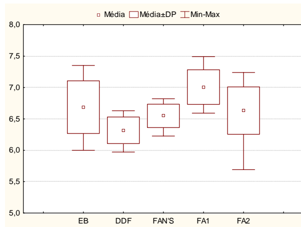
Figura 4.2: Box Plot de pH – FASE 01.
