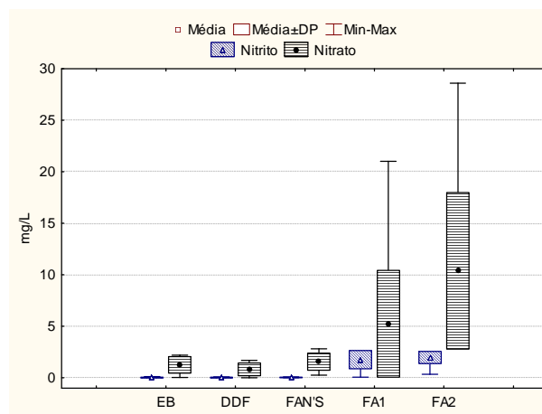
Figura 4.8: Box Plot de nitrito e nitrato geral – FASE 01
