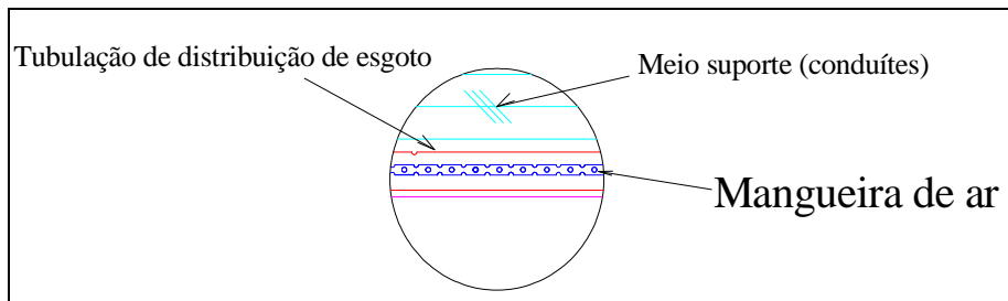
Figura 3.14: Detalhe B (coleta inferior de esgoto)
