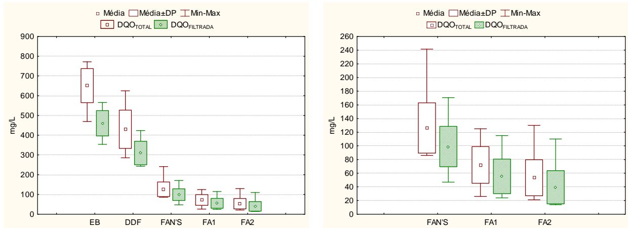
Figura 4.4: Boxs Plots de DQO total e DQO filtrada geral e ampliado – FASE 01.
