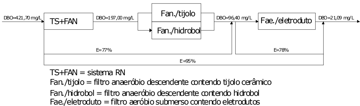
Figura 3.6: Esquema de eficiências esperadas para reator
