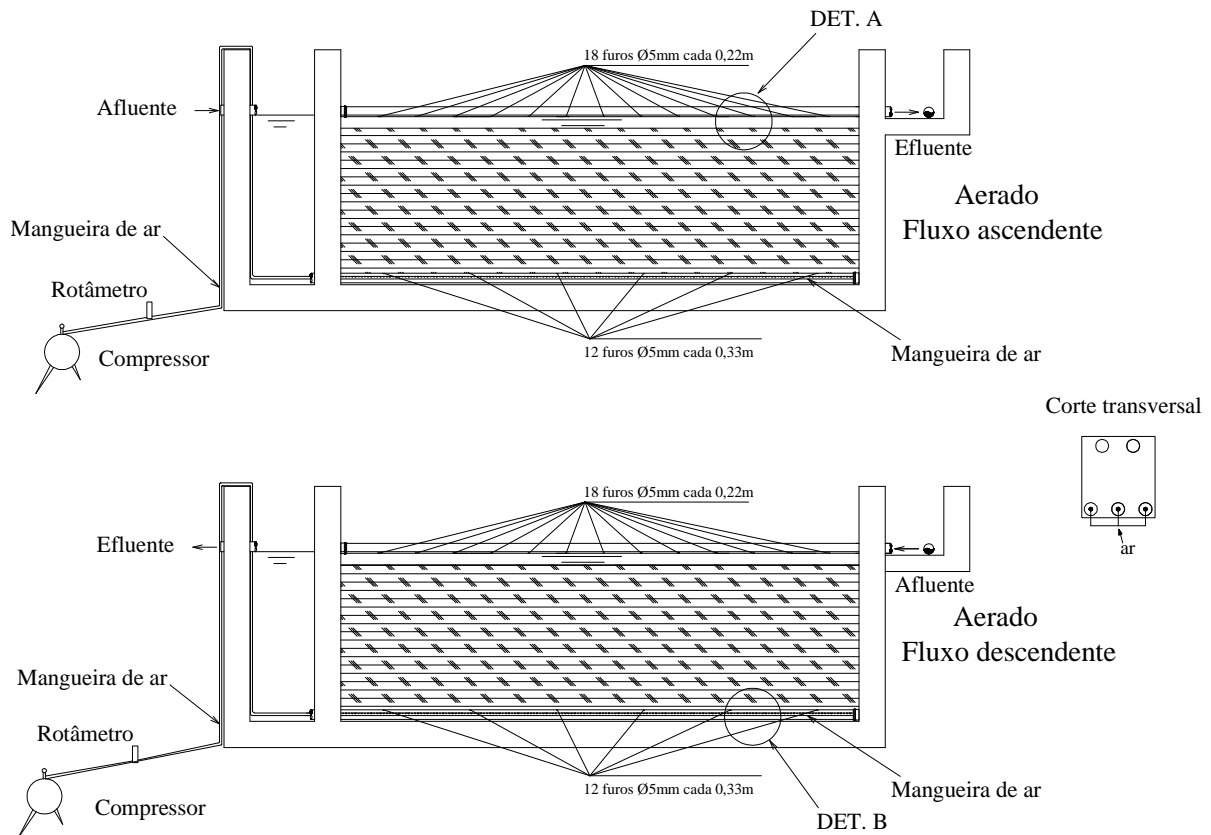
Figura 3.11: Detalhamento da furação. Tubulações de coleta no FA1 e de distribuição no FA2.
