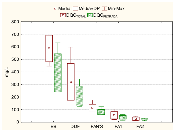
Figura 4.10: Boxs Plots de DQO total e DQO filtrada geral e ampliado – FASE 02.
