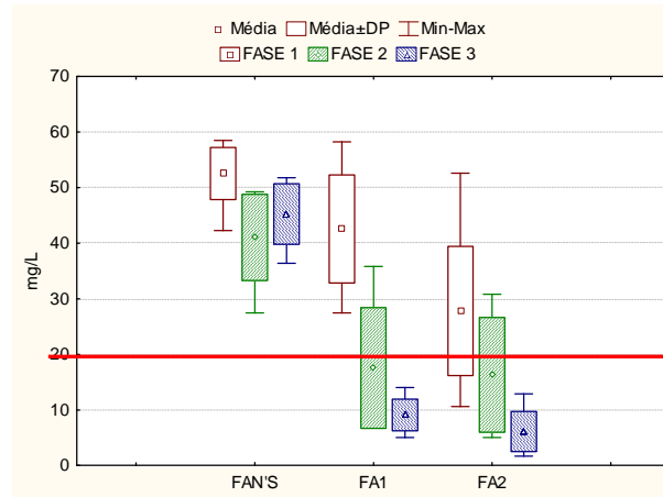
Figura 4.27: Nitrogênio amoniacal nas três fases ampliado.
