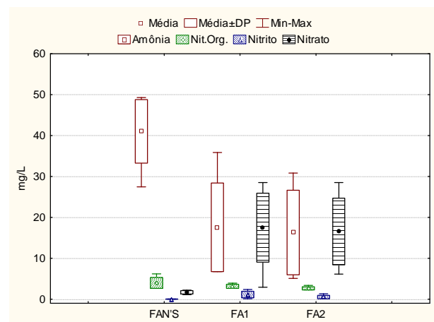
Figura 4.11: Boxs Plots de Amônia, Nitrogênio orgânico, nitrito e nitrato geral e ampliado – FASE 02.
