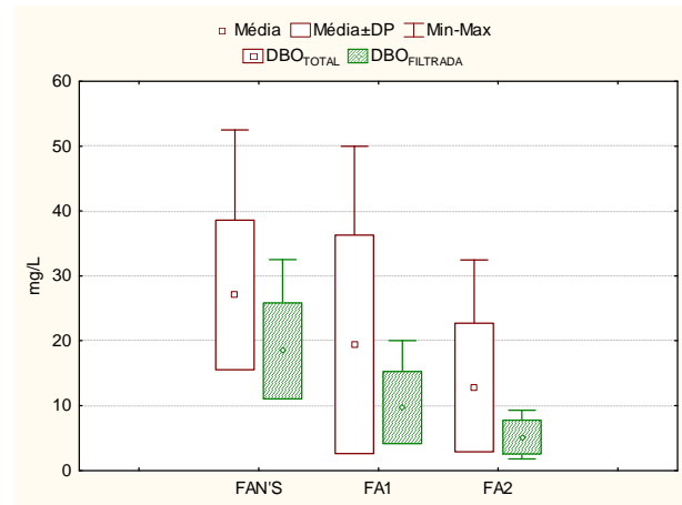
Figura 4.9: Boxs Plots de DBO total e DBO filtrada geral e ampliado – FASE 02.
