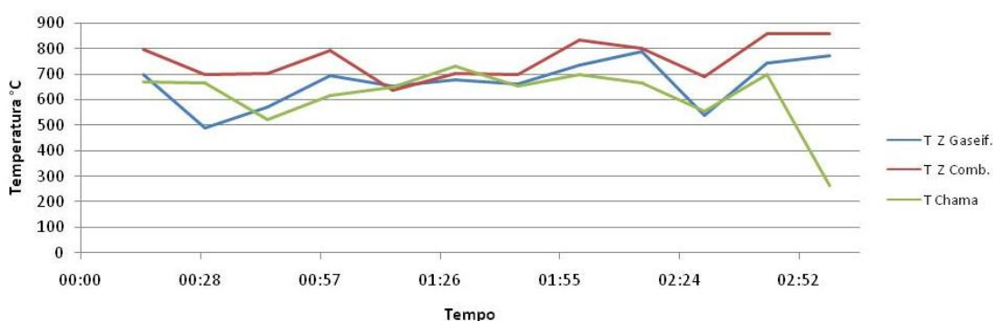
Figura 3.21 - Temperatura da zona de combustão, zona de gaseificação e da chama durante a gaseificação da palha de café.
