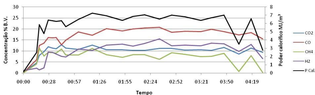
Figura 3.15 - Comportamento da composição do gás e poder calorífico em função do tempo de gaseificação durante o teste 1 com eucalipto.
