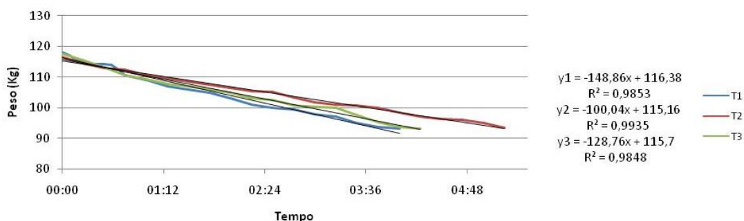
Figura 3.14 - Representação do consumo de cavaco de eucalipto em função do tempo de gaseificação nos testes T1, T2 e T3.
