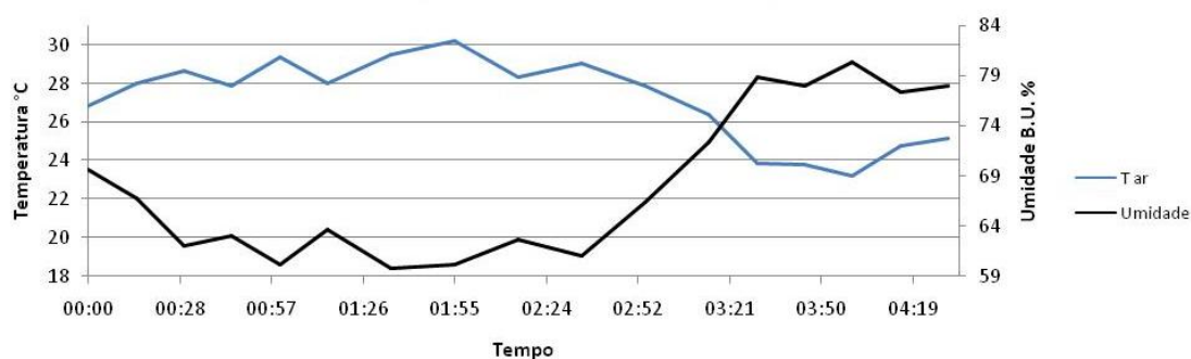
Figura 3.7 - Temperatura e umidade do agente gaseificante durante o teste 3 com cavacos de eucalipto.
