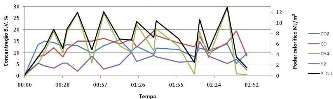
Figura 3.23 - Comportamento da composição do gás e poder calorífico em função do tempo de gaseificação durante o teste com palha de café.
