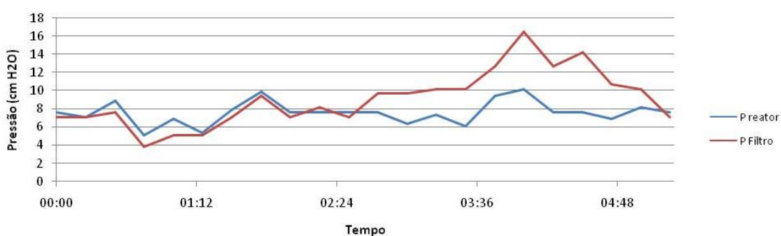
Figura 3.9 - Pressão negativa no reator e no filtro durante o tempo do teste 2 com cavacos de eucalipto.
