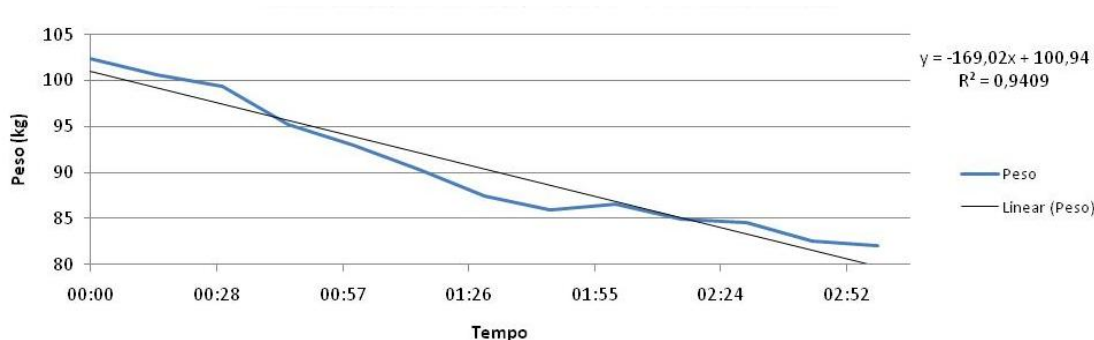
Figura 3.22 - Representação do consumo de palha de café em função do tempo de gaseificação.
