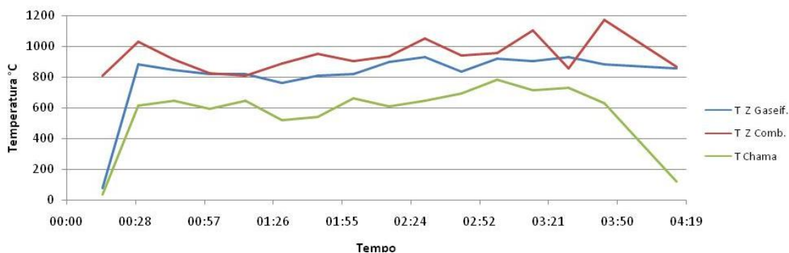
Figura 3.27 - Temperatura da zona de combustão, zona de gaseificação e da chama durante a gaseificação da lenha do cafeeiro.
