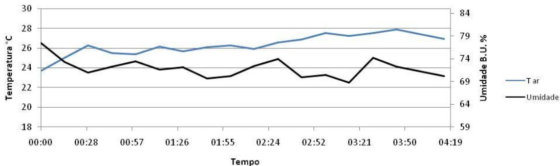
Figura 3.25 - Temperatura e umidade do ar (agente gaseificante) durante o tempo de gaseificação da lenha oriundo de cafeeiro.
