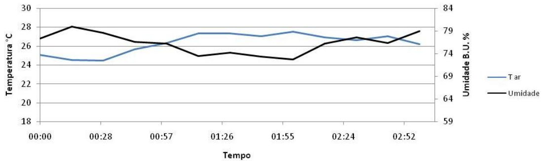
Figura 3.19 - Temperatura e umidade do agente gaseificante (ar) durante gaseificação da palha do café.
