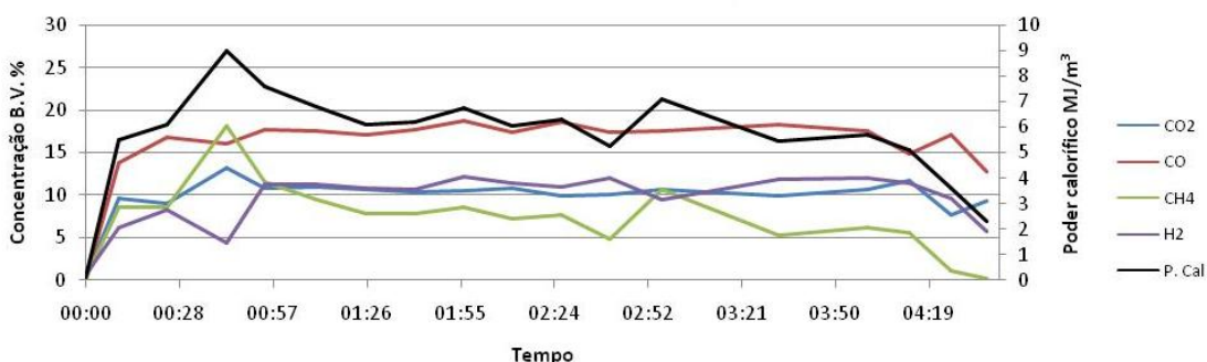
Figura 3.17 - Comportamento da composição do gás e poder calorífico em função do tempo de gaseificação durante o teste 3 com eucalipto.
