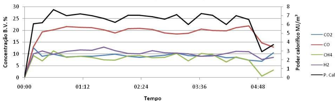
Figura 3.16 - Comportamento da composição do gás e poder calorífico em função do tempo de gaseificação durante o teste 2 com eucalipto.
