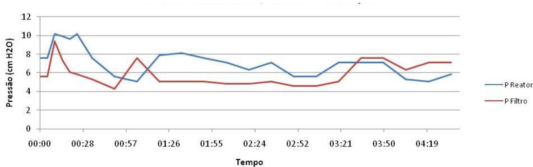
Figura 3.8 - Pressão negativa no reator e no filtro durante o tempo do teste 1 com cavacos de eucalipto.
