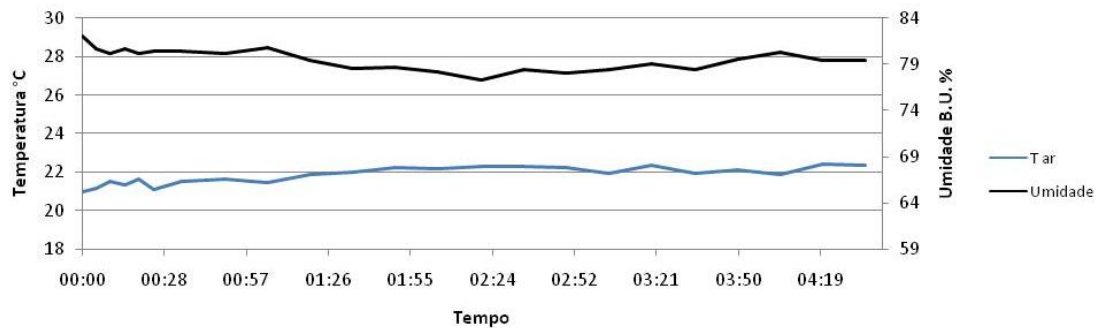
Figura 3.5 - Temperatura e umidade do agente gaseificante durante o teste 1 com cavacos de eucalipto.
