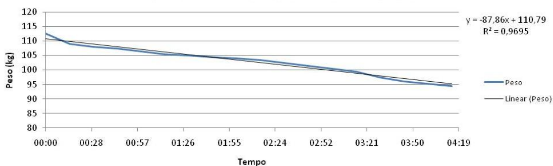
Figura 3.28 - Representação do consumo de biomassa em função do tempo de gaseificação.
