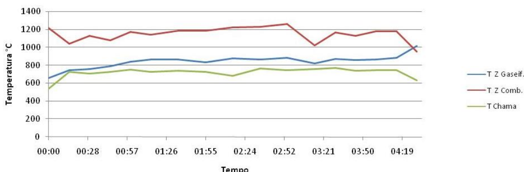
Figura 3.13 - Temperatura da zona de combustão, zona de gaseificação e da chama durante o teste 3 com cavacos de eucalipto.
