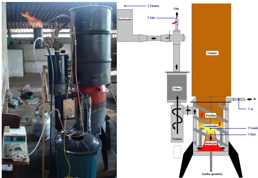
Figura 3.1 - Sistema de gaseificação - gaseificador com os componentes secundários e esquematização do processo.
