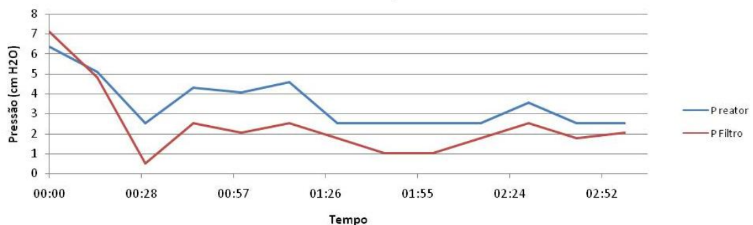
Figura 3.20 - Pressão negativa no reator e no filtro durante a gaseificação da palha de café.
