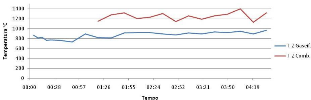
Figura 3.11 - Temperatura da zona de combustão e da zona de gaseificação durante o teste 1 com cavacos de eucalipto.
