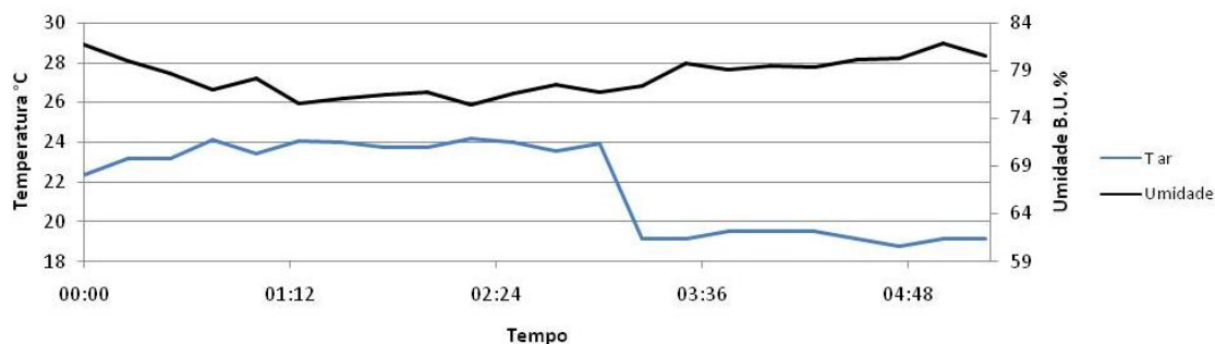
Figura 3.6 - Temperatura e umidade do agente gaseificante durante o teste 2 com cavacos de eucalipto.
