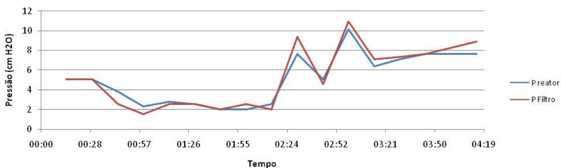
Figura 3.26 - Pressão negativa no reator e no filtro durante a gaseificação da lenha do cafeeiro.
