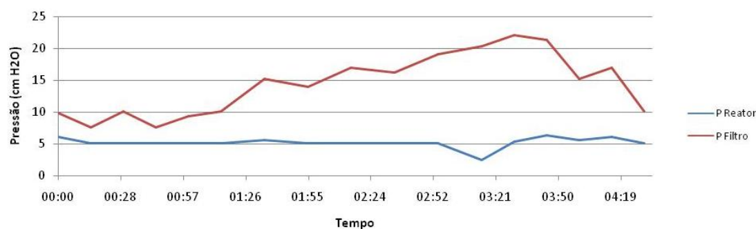
Figura 3.10 - Pressão negativa no reator e no filtro durante o tempo do teste 3 com cavacos de eucalipto.
