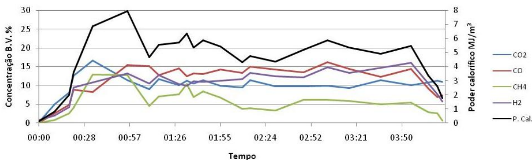
Figura 3.29 - Comportamento da composição do gás e poder calorífico em função do tempo de gaseificação durante o teste com lenha de cafeeiro.
