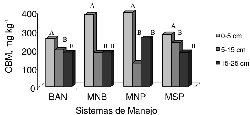
Figura 2. Teores de carbono da biomassa microbiana em amostras de solo, sob diferentes sistemas de manejo, na Chapada do Apodi - CE. Médias seguidas pela mesma letra não diferem entre si a 5%, pelo teste de Tukey: A e B comparam as áreas.
