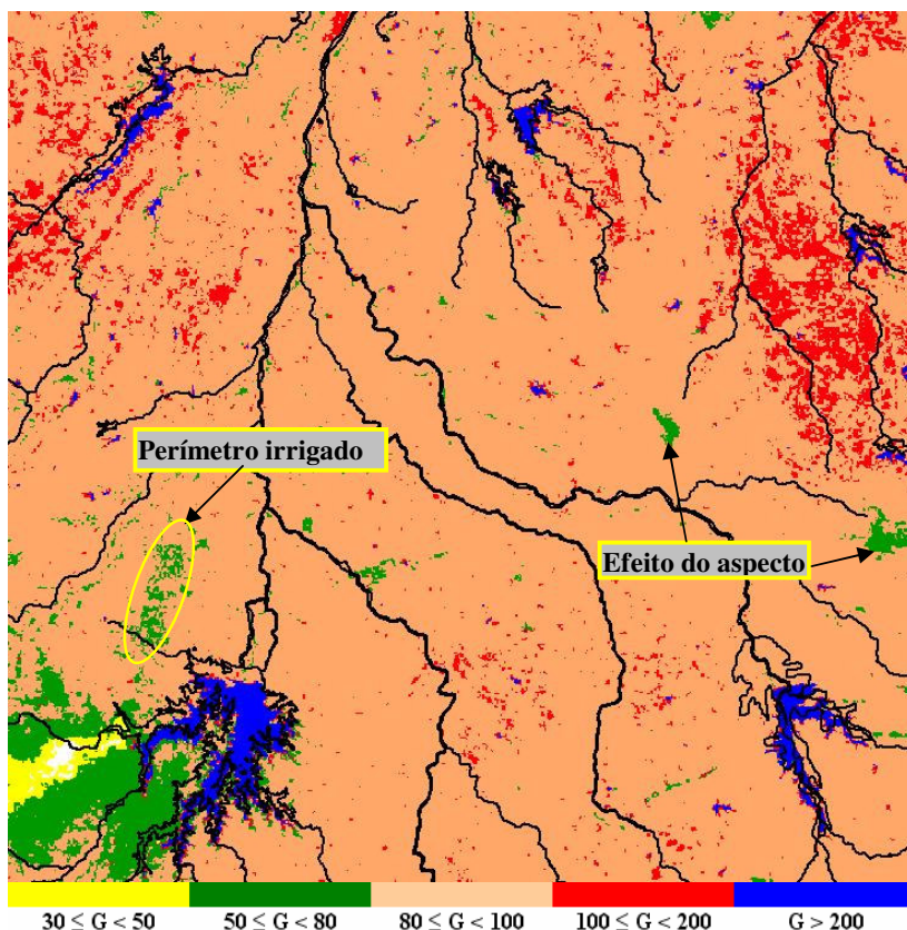
FIGURA 16: Cena do fluxo de calor do solo ( \text{W.m}^{-2} ) para o dia 01/09/2004.
