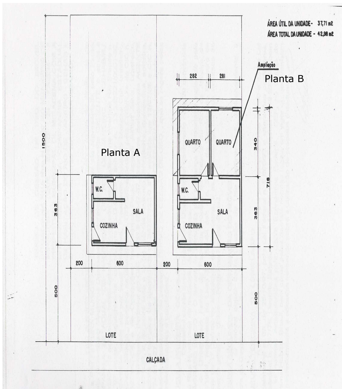
Figura 5.- Planta do embrião da moradia popular (Planta A) e planta para a ampliação da moradia, que deveria ser feita pelos moradores (Planta B). CRHL, 2007.
