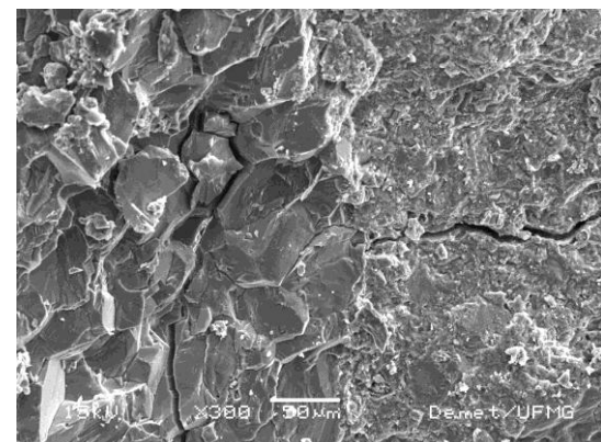
(d) Normal-weight concrete (300X)
