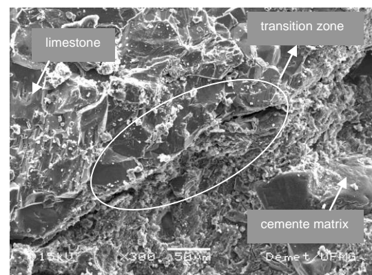
(d) normal-weight concrete - 40 MPa (300X)
