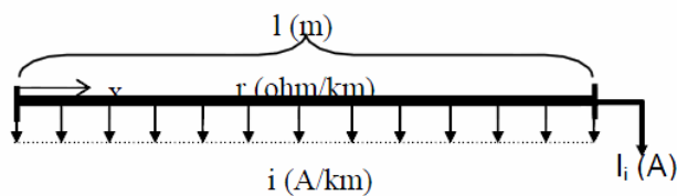
Figura 2.5 - Trecho de rede elementar
