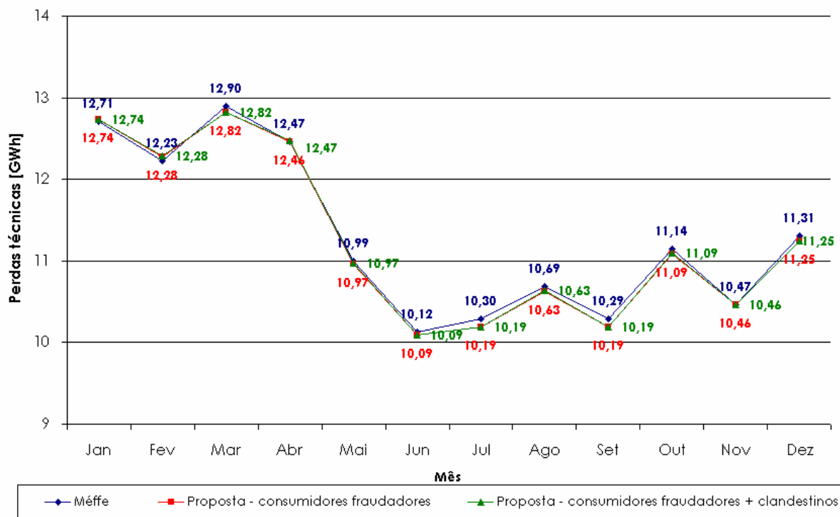
Figura 4.6 – Cálculo das perdas técnicas na área piloto: metodologia de Meffe e proposta - janeiro a dezembro/2008
