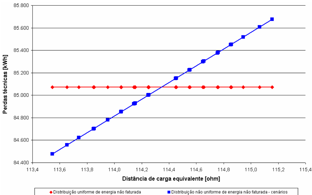
Figura 4.4 – Perdas técnicas obtidas através da metodologia de Meffe e perdas técnicas calculadas para o caso base de cada cenário proposto, em função da distância de carga equivalente. Detalhes no APÊNDICE V.
