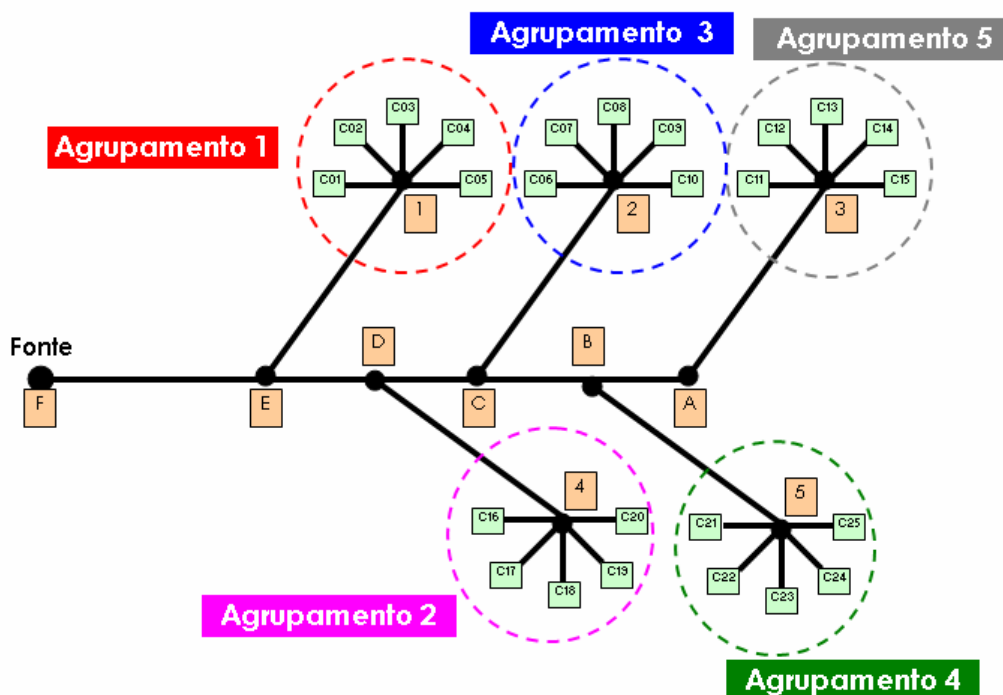
Figura 4.1 - Topologia de testes utilizada.
