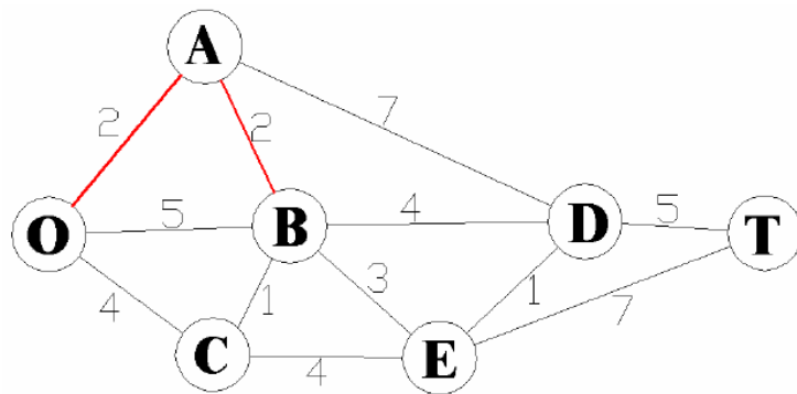
Figura A.3 - Rede após a segunda etapa: nó "B" conectado ao nó "A".
