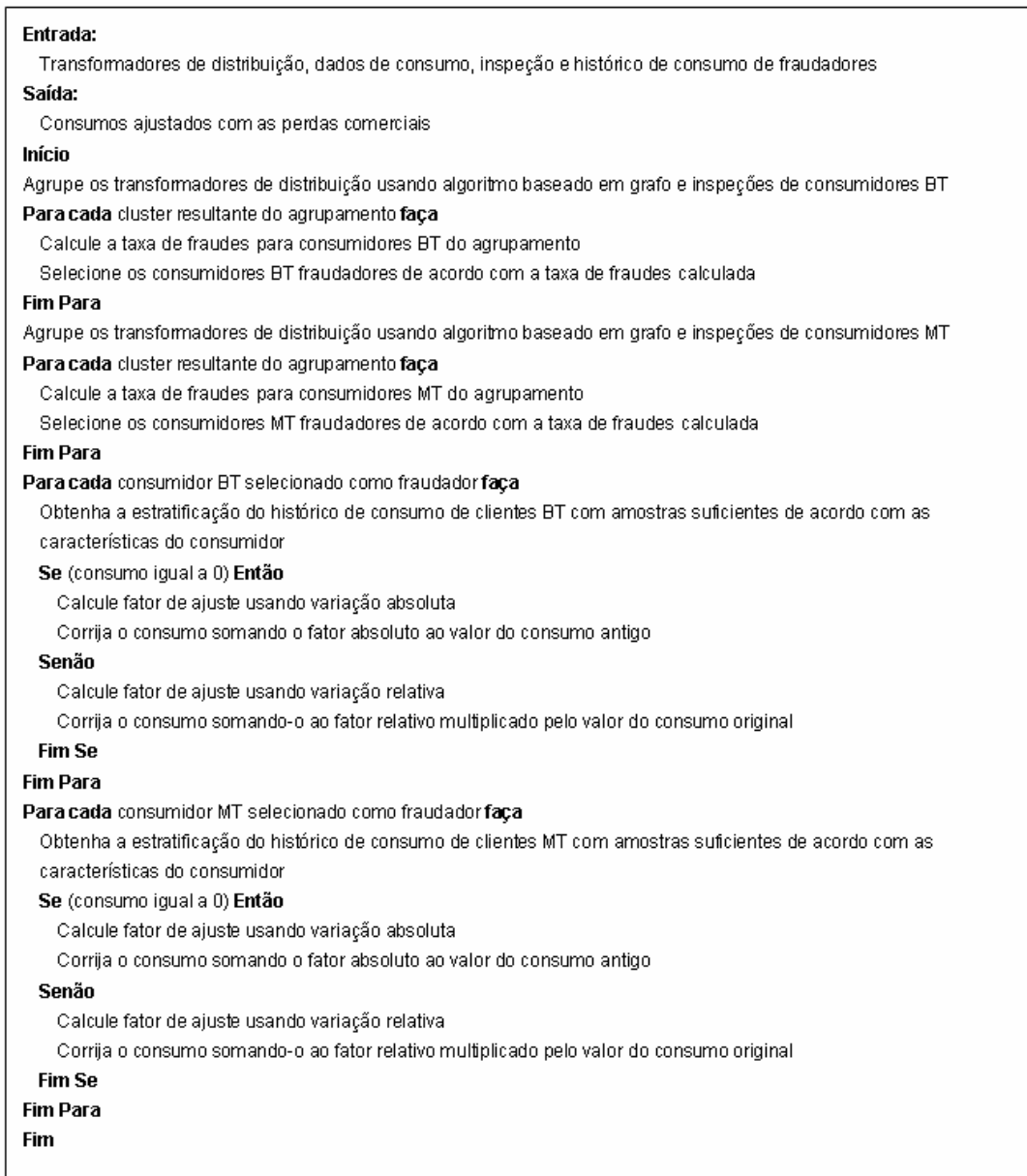
Figura 3.3 - Metodologia para estimativa das perdas não técnicas e ajuste dos consumos
