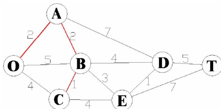
Figura A.4 - Rede após a terceira etapa: nó "C" conectado ao nó "B".
