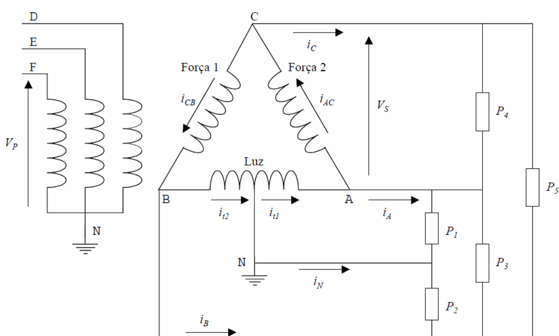
Figura 2.9 - Representação de uma unidade transformadora com três transformadores monofásicos na ligação delta fechada. Retirado de Meffe (2001)
