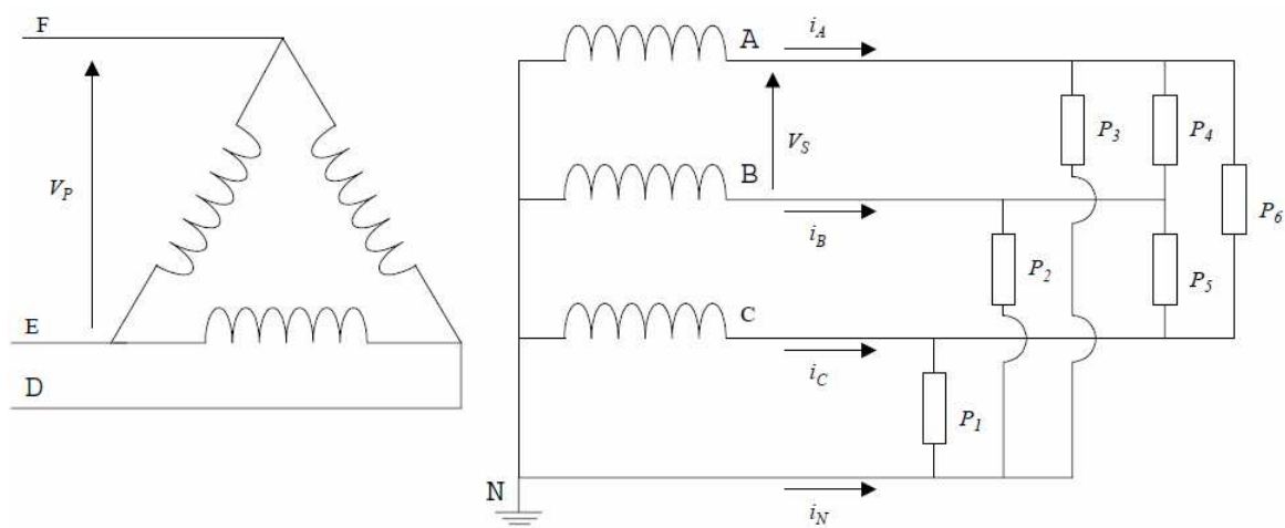
Figura 2.10 - Representação de uma unidade transformadora com um transformador trifásico na ligação delta-estrela. Retirado de Meffe (2001)
