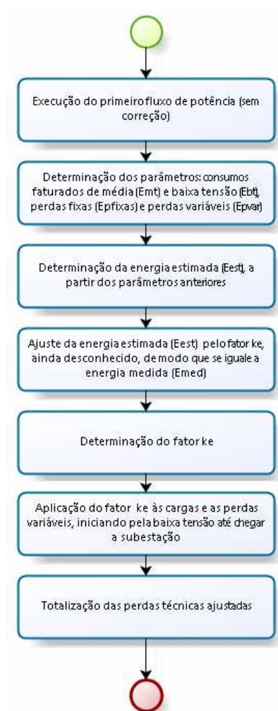
Figura 2.11 - Etapas da metodologia desenvolvida por Meffe.
