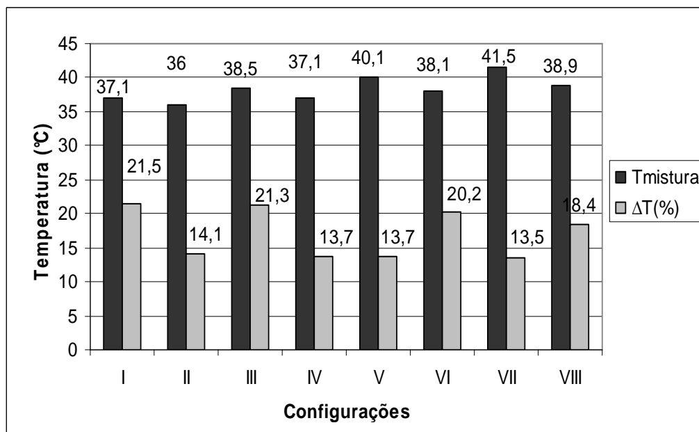
Figura 4.11. Comportamento assumido pela temperatura da água depois de misturada para as configurações estudadas a variação percentual entre a temperatura da água do fundo do reservatório ( T_f ) com a do topo ou em cima ( T_c ) no final do ensaio.
