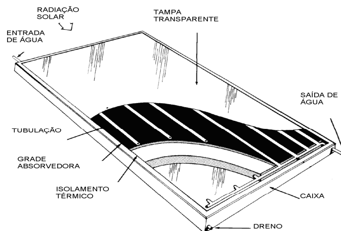
Figura 2.5. Coletor solar com seus principais componentes.
