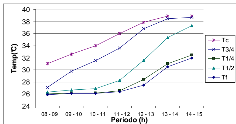
Figura 4.2. Comportamento assumido pela temperatura da água em vários pontos do reservatório térmico – Configuração I.
