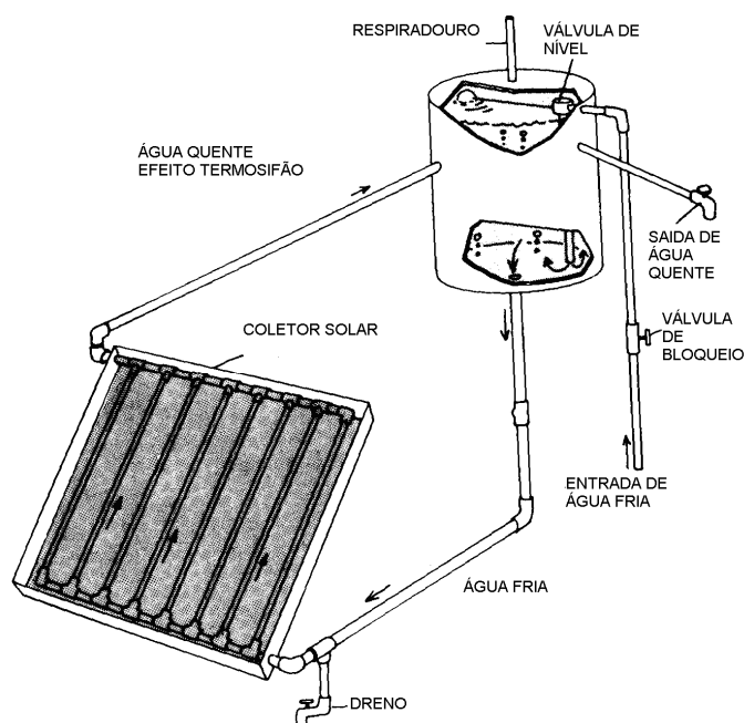
Figura 2.8. Esquema básico de um sistema de aquecimento solar convencional por termosifão ou convecção natural. (DICKINSON, CHEREMISINOFF, 1980).
