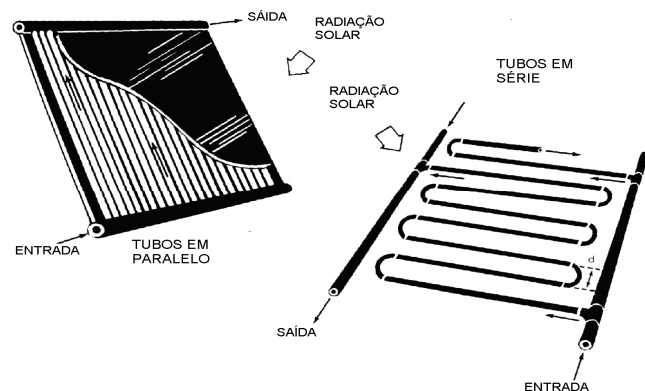
Figura 2.7. Esquemas típicos de ligação dos tubos absorvedores de coletores planos (DICKINSON, CHEREMISINOFF, 1980).
