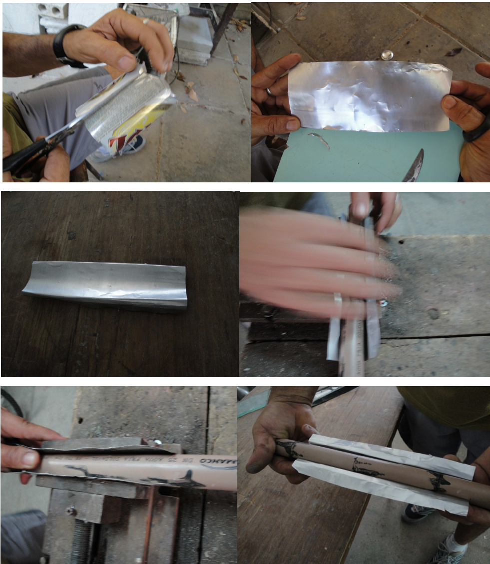
Figura 3.3. Etapas da construção das aletas com latas de alumínio.
