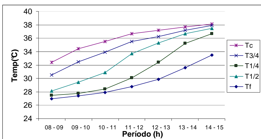
Figura 4.7. Comportamento assumido pela temperatura da água em vários pontos do reservatório térmico – Configuração IV.
