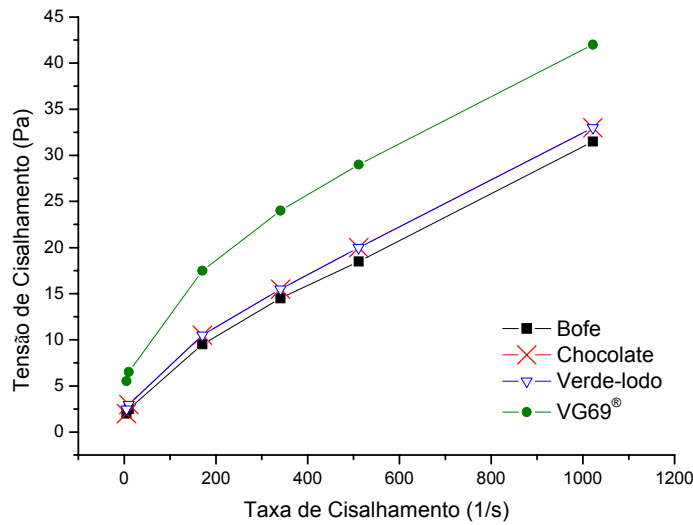
Figura 25: Curvas de fluxo dos fluidos (base parafina) das argilas Bofe, Chocolate UBM, Verde-lodo, organofilizadas com tensoativo não-iônico, e da VG69®
