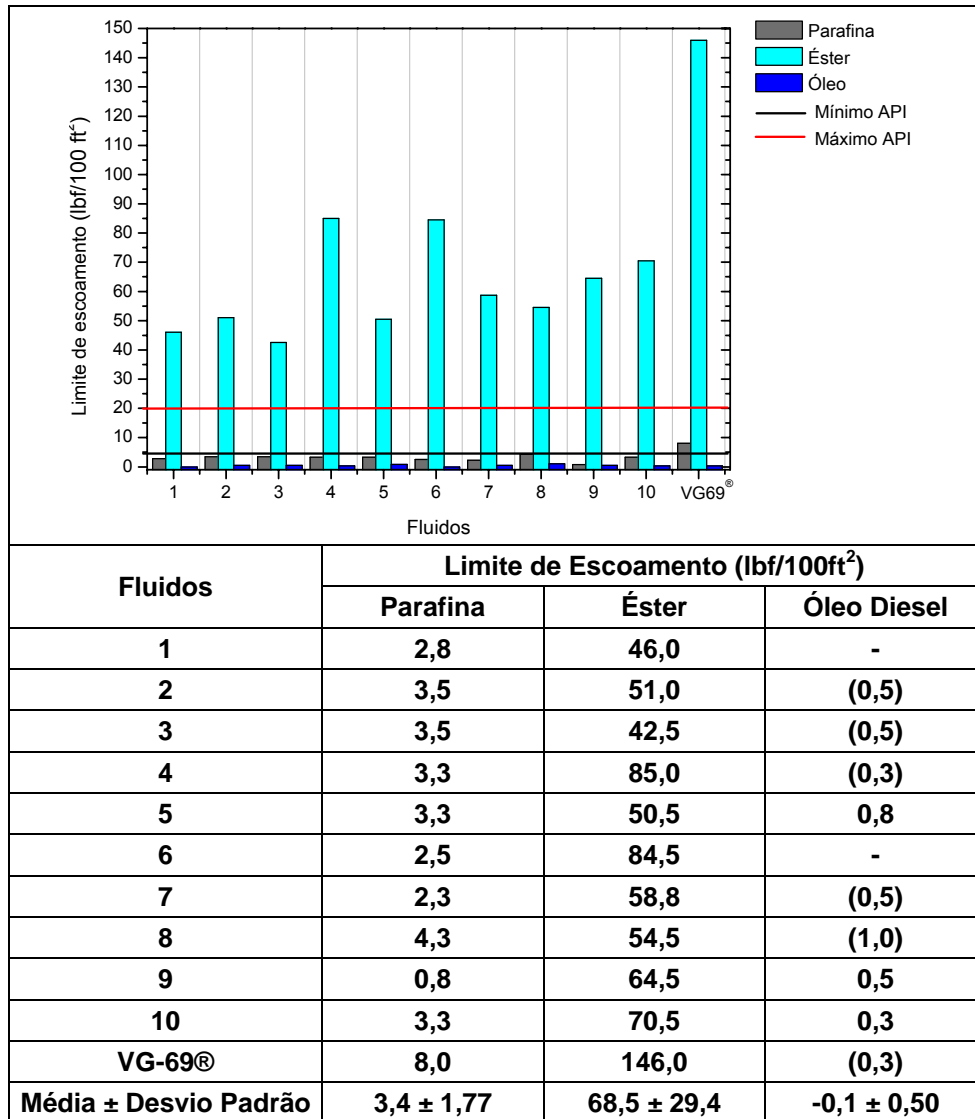
Figura 38: Limite de escoamento dos fluidos formulados com as composições de argilas e com a argila VG69 ® . Fluido 1: B (100%); Fluido 2: C (100%); Fluido 3: V (100%); Fluido 4: BC (50% + 50%); Fluido 5: BV (50% + 50%); Fluido 6: CV (50% + 50%); Fluido 7: BCV (33,3% + 33,3% + 33,3%); Fluido 8: BCV (66% + 16% + 16%); Fluido 9: BCV (16% + 66% + 16%); Fluido 10: BCV (16% + 16% + 66%)
