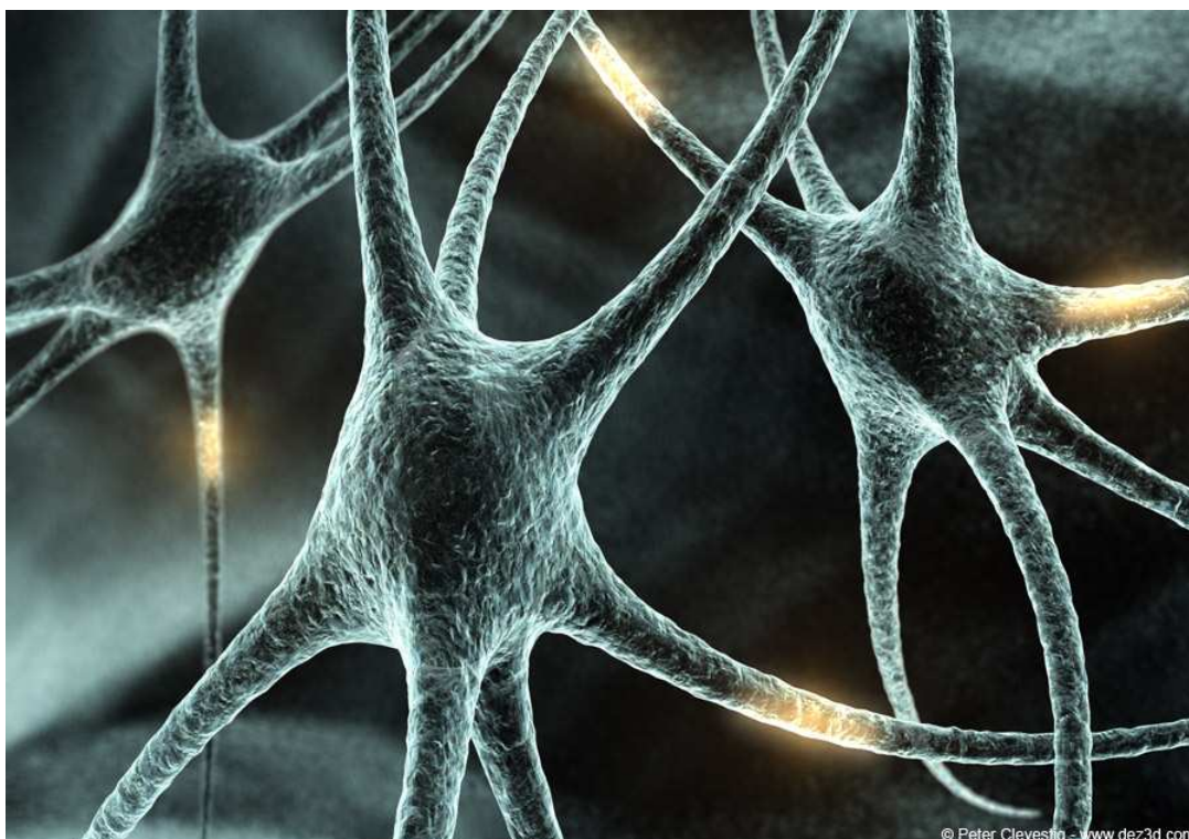
Figura n. 01 – Redes Neurais
