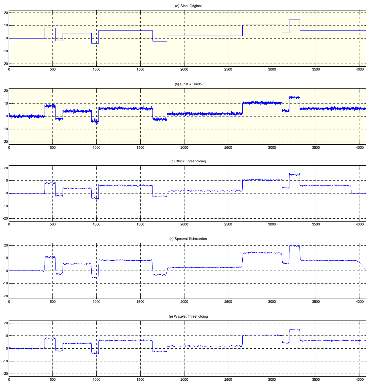
Figura 4.12 (a), (b): Blocks original e ruidosa. (c), (d), (e): Blocks tratada com cada uma das técnicas indicadas. O eixo vertical representa a magnitude e o horizontal o número de amostras pontuais.
