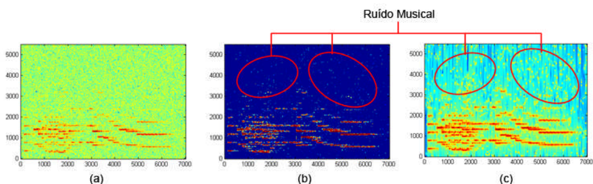
Figura 2.8 Espectrograma do sinal ruidoso (a), fatores de atenuação do ruído não regularizados (b) e o sinal filtrado exibindo os coeficientes frequenciais isolados que correspondem ao ruído musical (c) [8].
