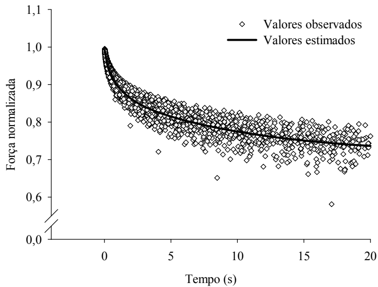
Figura 1.3. Valores observados e estimados pelo modelo generalizado de Maxwell da força requerida para se manter uma deformação específica de 0,005 m nos frutos de tomateiro não submetidos à compressão (testemunha), na temperatura de 15 °C (A).
