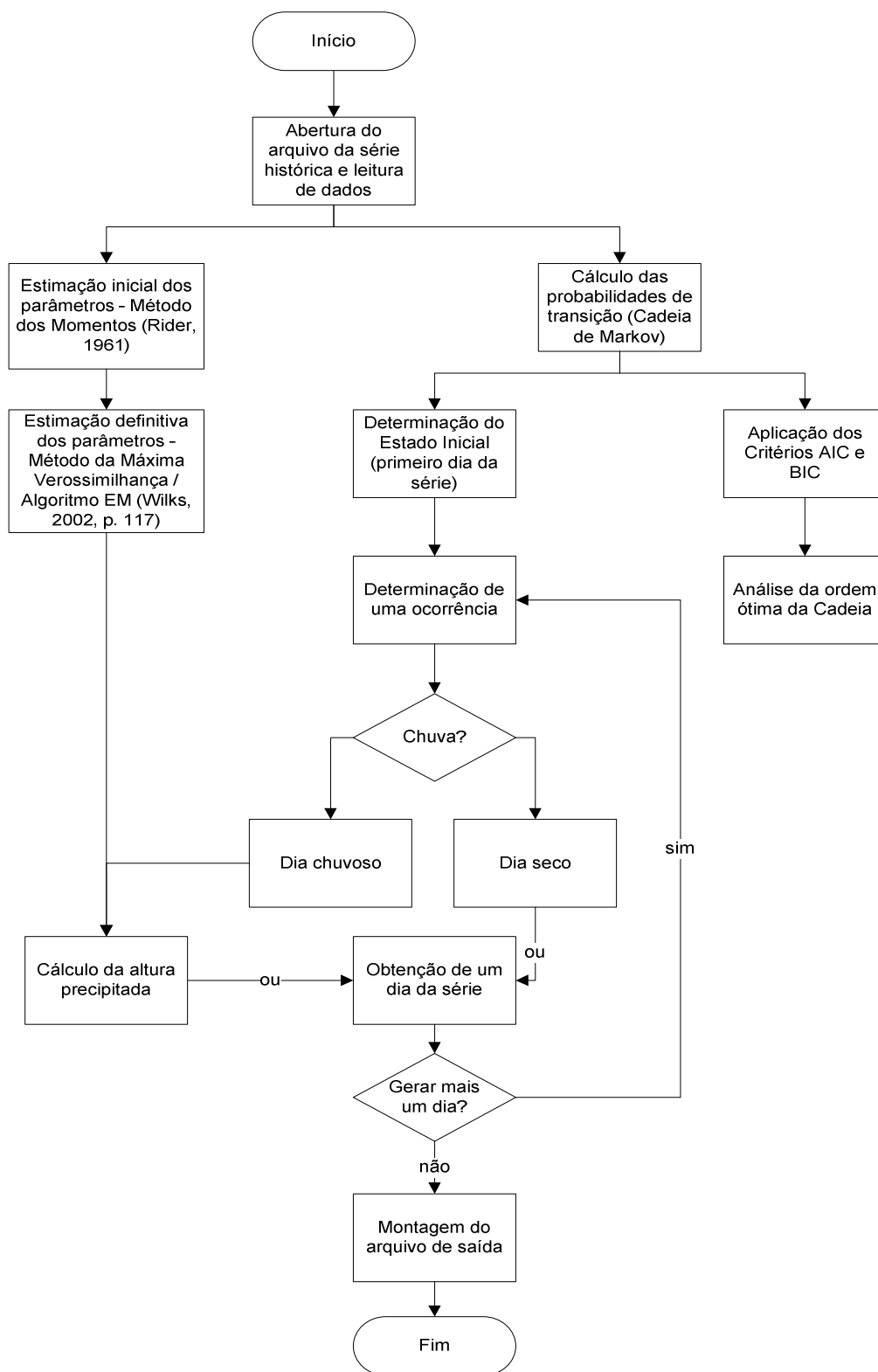
FIGURA 8 – ALGORITMO DE GERAÇÃO DE SÉRIES SINTÉTICAS
