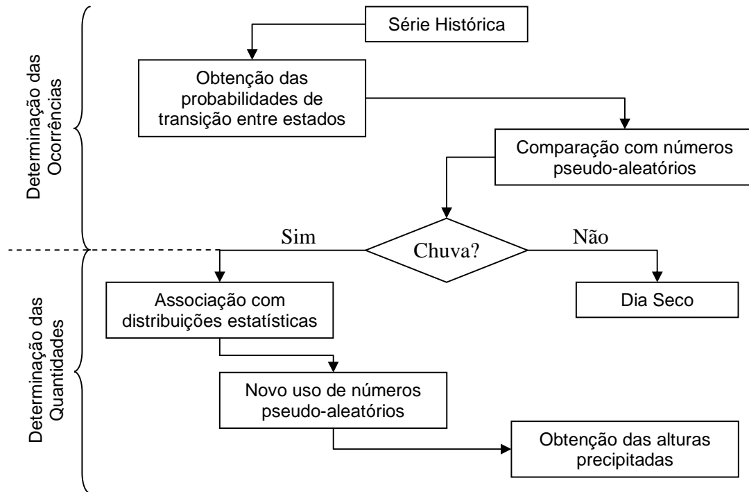
FIGURA 2 - ESTRUTURA GENÉRICA DE UM MODELO PARAMÉTRICO
