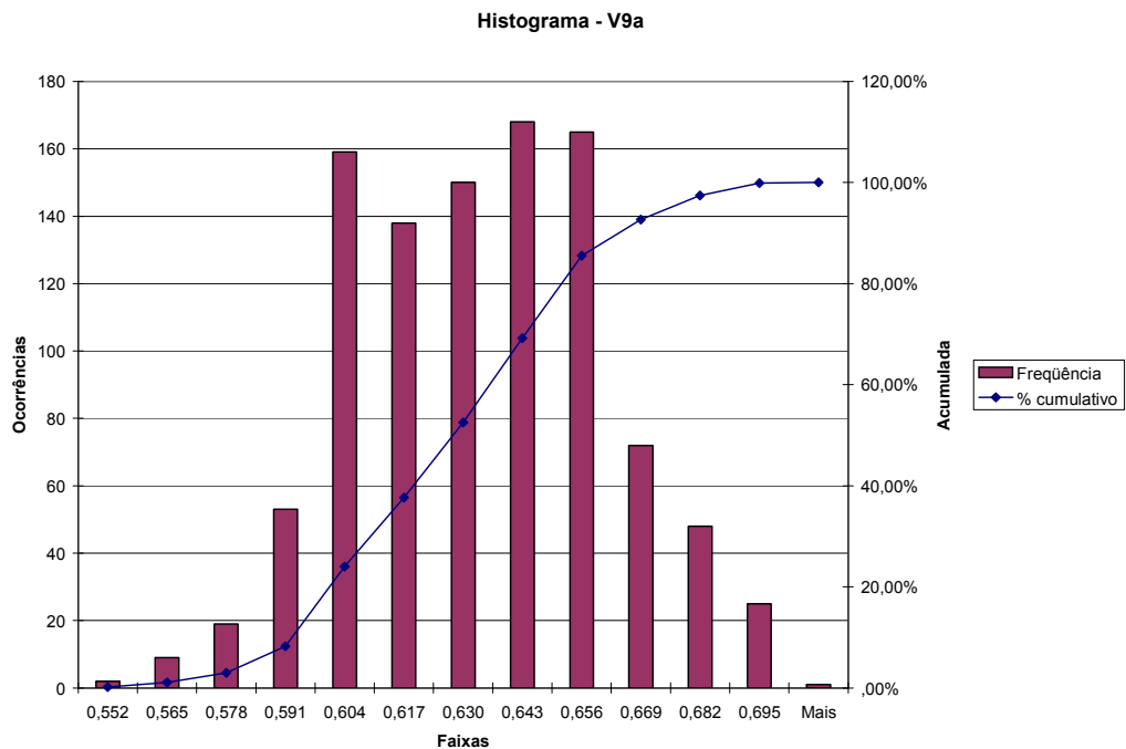
Figura A.64 – Distorção para o 9º harmônico de tensão na fase A – TPC
