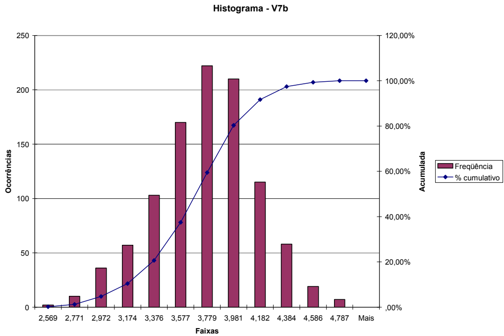
Figura A.62 – Distorção para o 7º harmônico de tensão na fase B – TPC
