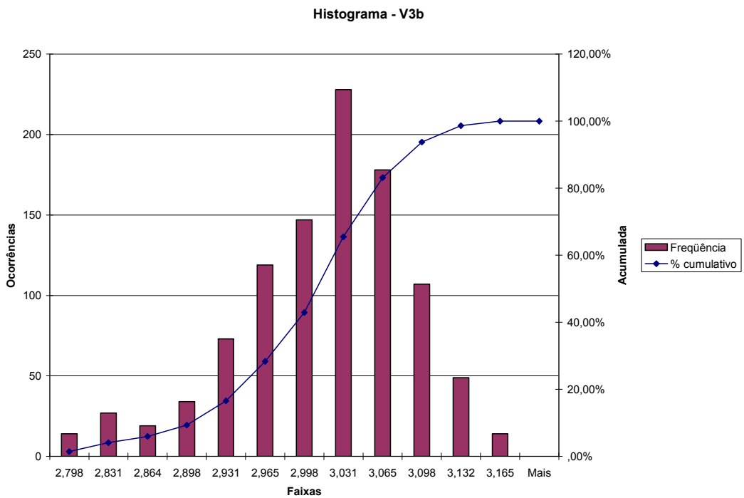
Figura A.59 – Distorção para o 3º harmônico de tensão na fase B – TPC
