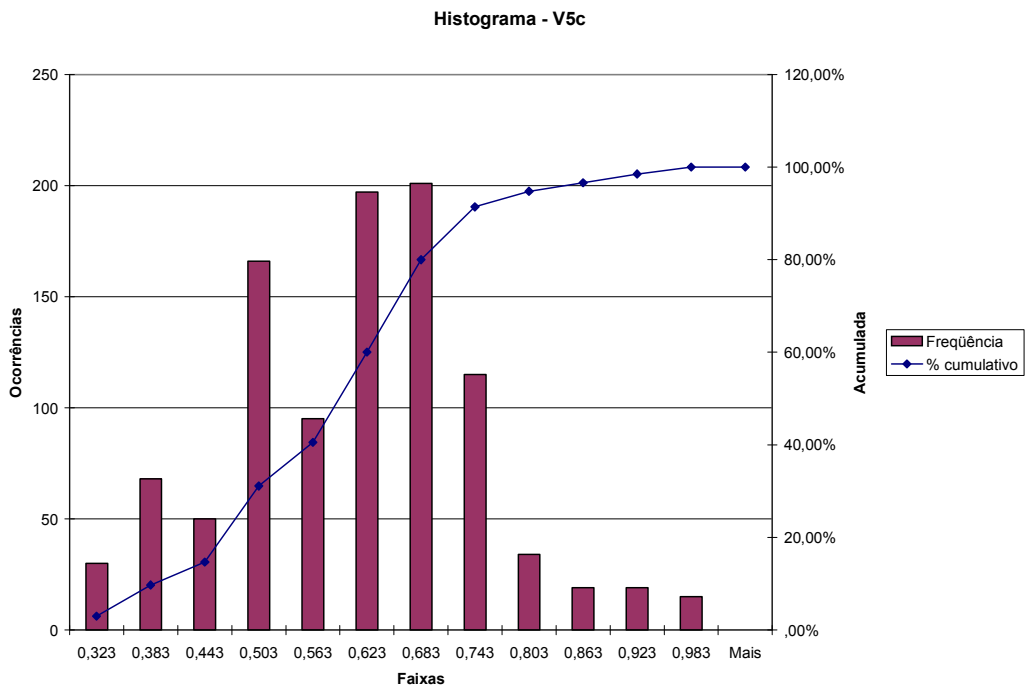
Figura A.51 – Distorção para o 5º harmônico de tensão na fase C – TPI (cabo blindado)
