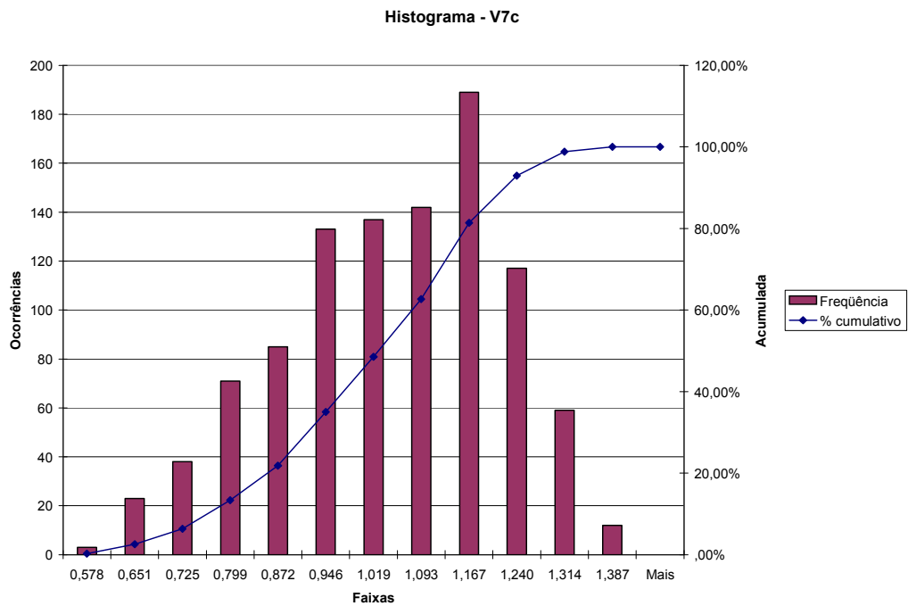
Figura A.63 – Distorção para o 7º harmônico de tensão na fase C – TPC
