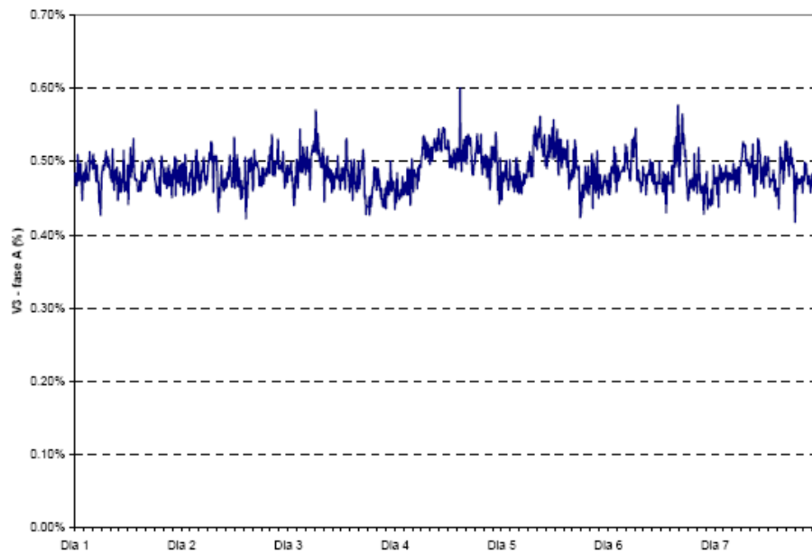
Figura 3.26 – Exemplo de gráfico tipo linha com valores de V_3 medidos na fase A
