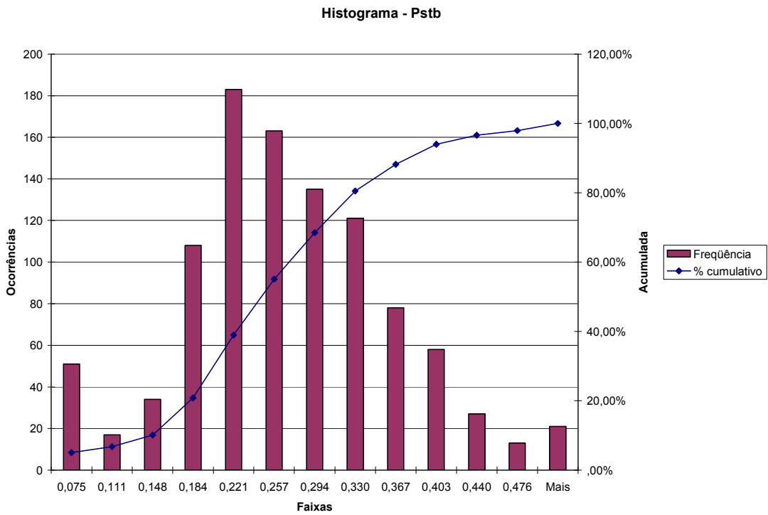
Figura A.26 – Histograma para P_{st} na fase B – TPC
