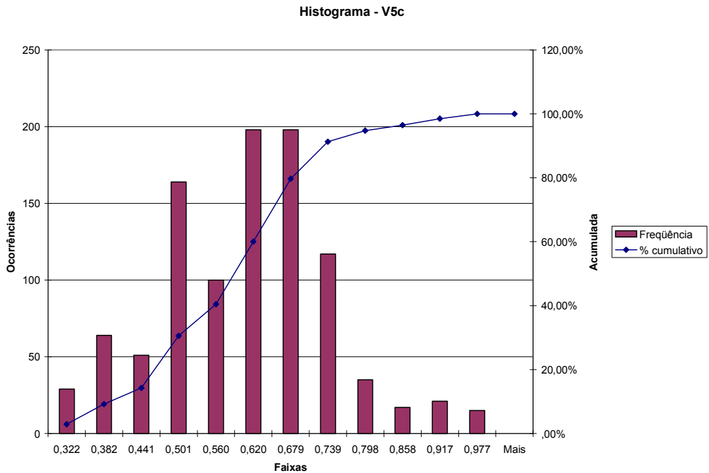
Figura A.54 – Distorção para o 5º harmônico de tensão na fase C – TPI (cabo comum)
