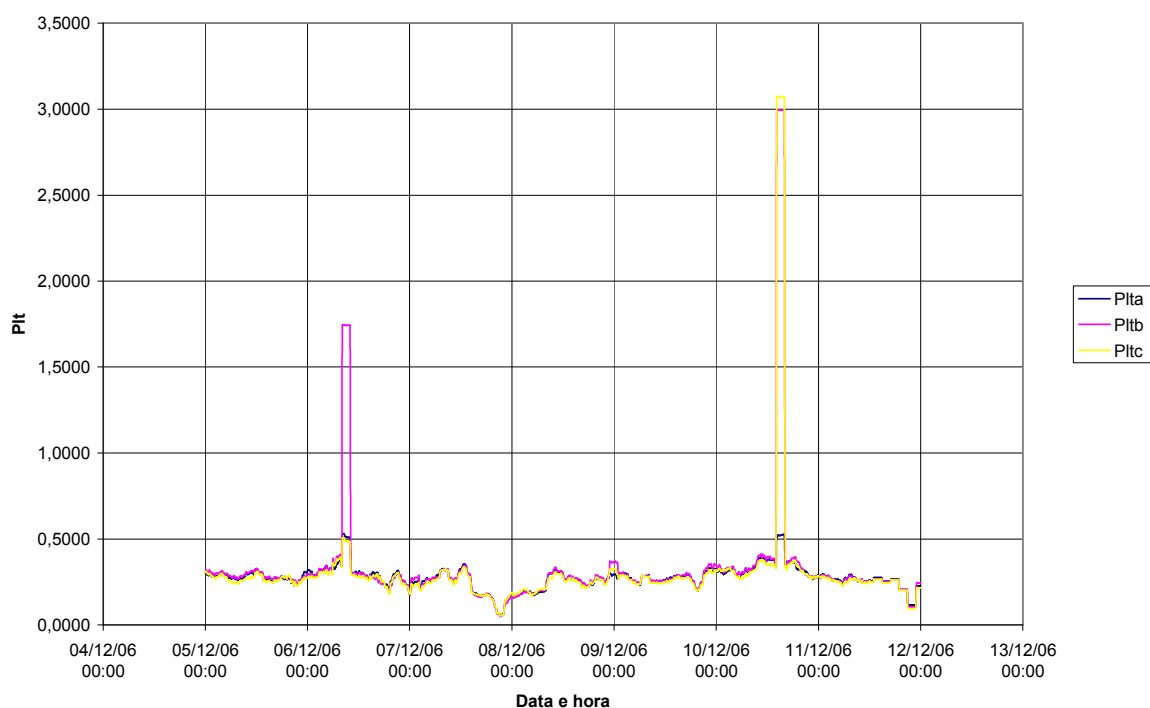
Figura A.12 – Plt por fase – TPC.
