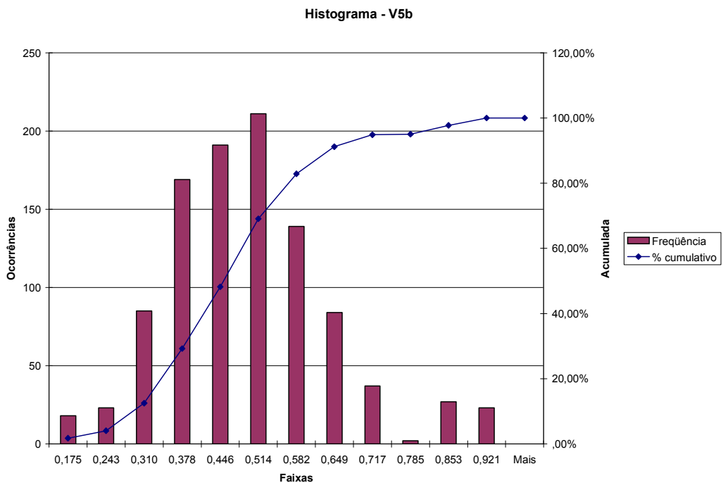
Figura A.50 – Distorção para o 5º harmônico de tensão na fase B – TPI (cabo blindado)
