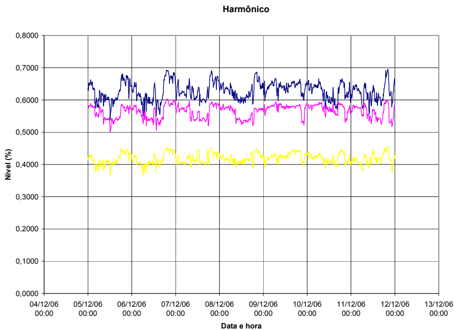
Figura A.39 – Distorção para o 9º harmônico de tensão por fase – TPC
