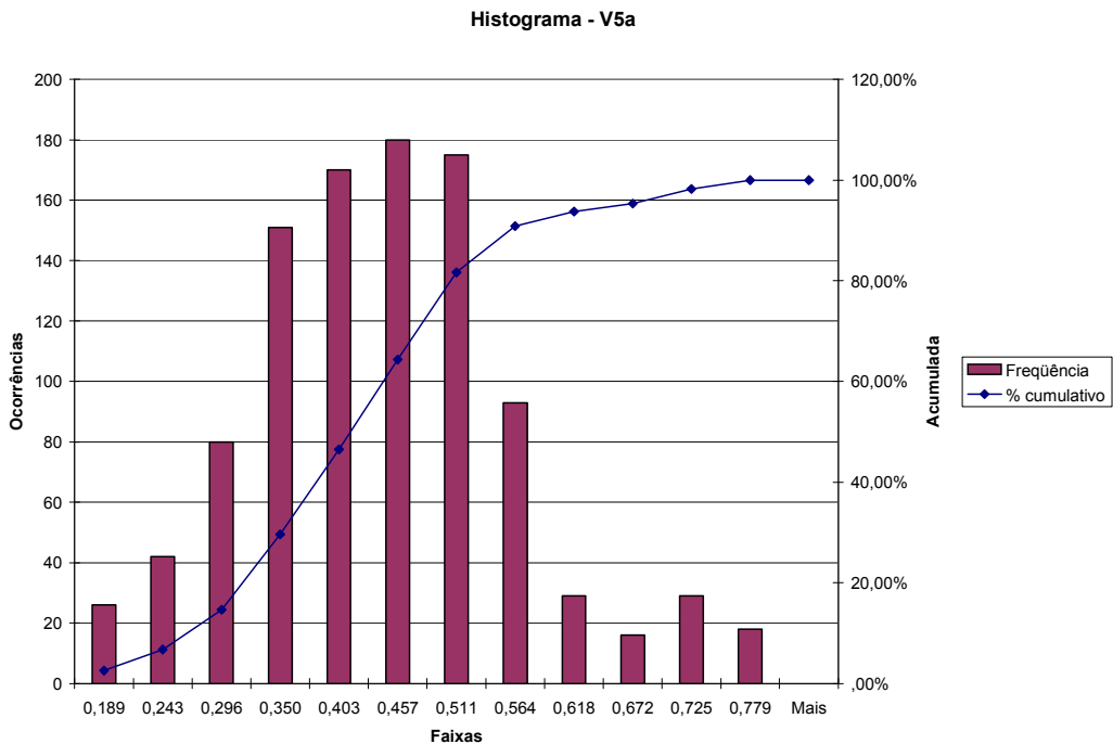
Figura A.52 – Distorção para o 5º harmônico de tensão na fase A – TPI (cabo comum)
