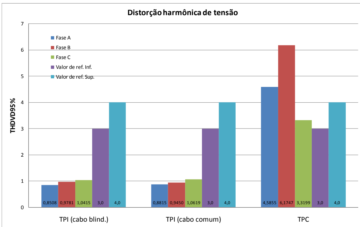
Figura 4.16 – Distorção harmônica total de tensão na fase B – TPC
