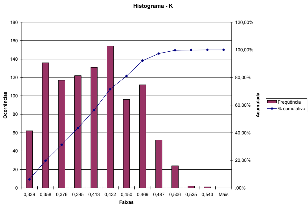
Figura A.4 – Histograma para o desequilíbrio de tensão – TPI (cabo blindado)
