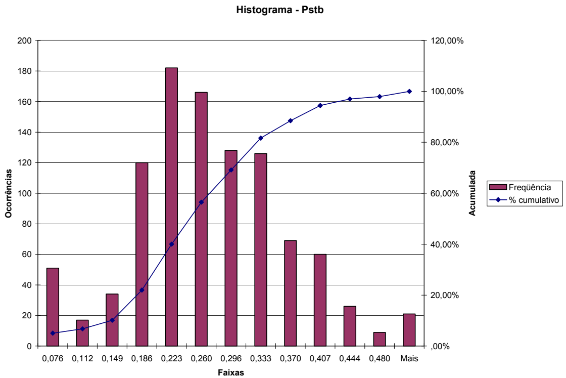
Figura A.14 – Histograma para P_{st} na fase B – TPI (cabo blindado)
