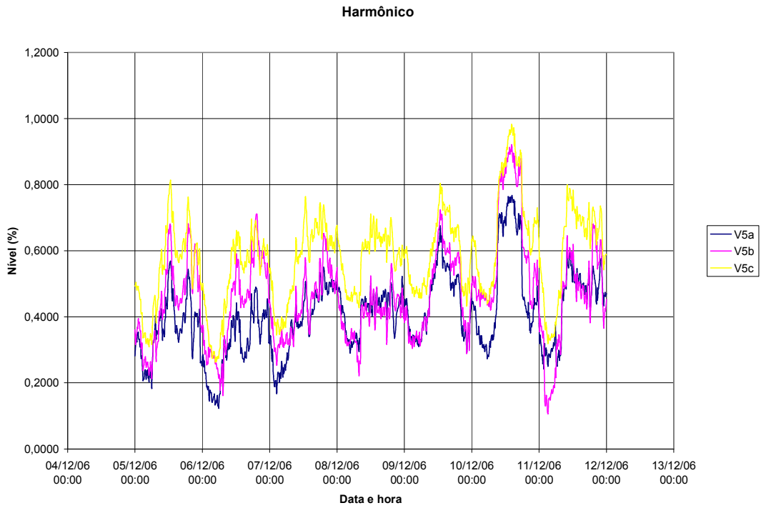
Figura A.34 – Distorção para o 5º harmônico de tensão por fase – TPI (cabo blindado)
