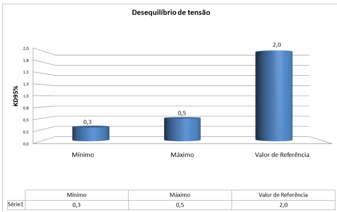
Figura 4.14 – Resultado da medição de desequilíbrio de tensão na SE PAL 10
