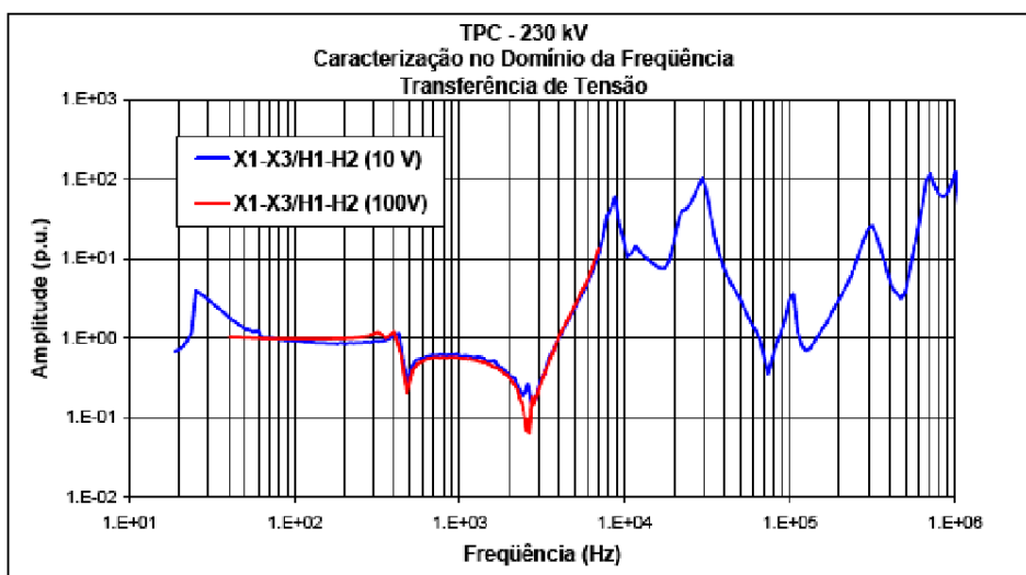
Figura 3.11 – Característica em frequência de um TPC
