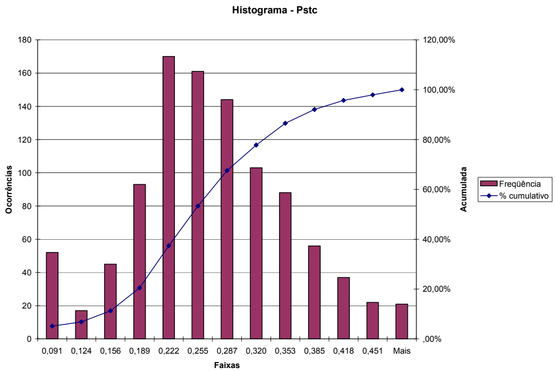
Figura A.21 – Histograma para P_{st} na fase C – TPI (cabo comum)
