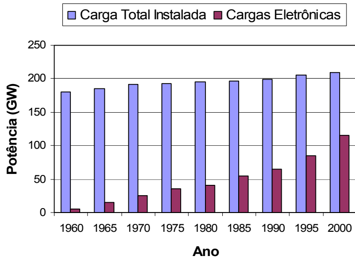
Figura 2.1 – Crescimento das cargas eletrônicas nos EUA
