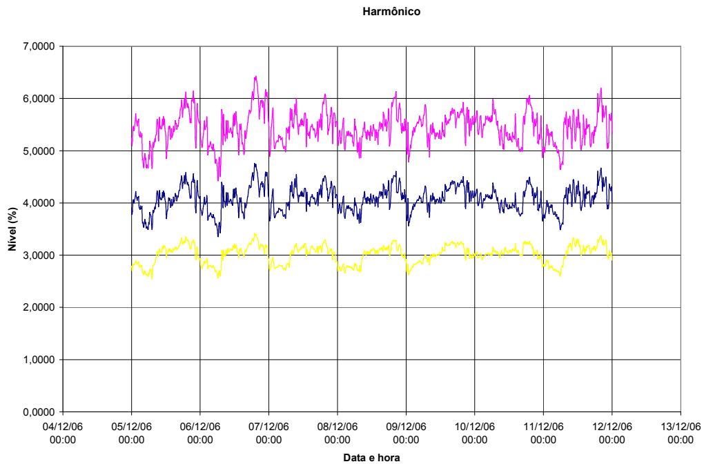
Figura A.33 – Distorção harmônica total de tensão por fase – TPC
