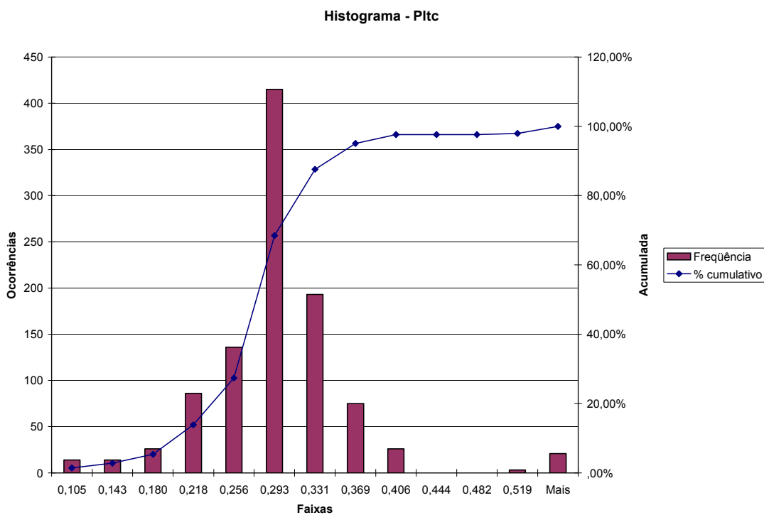
Figura A.24 – Histograma para Plt na fase C – TPI (cabo comum)
