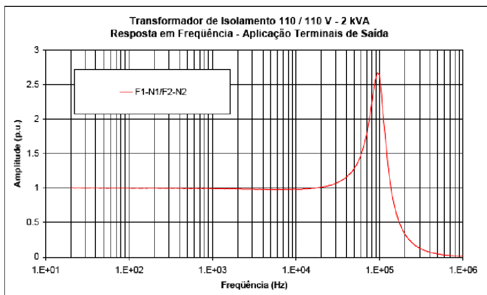
Figura 3.13 – Curva de resposta em frequência de um transformador de isolamento
