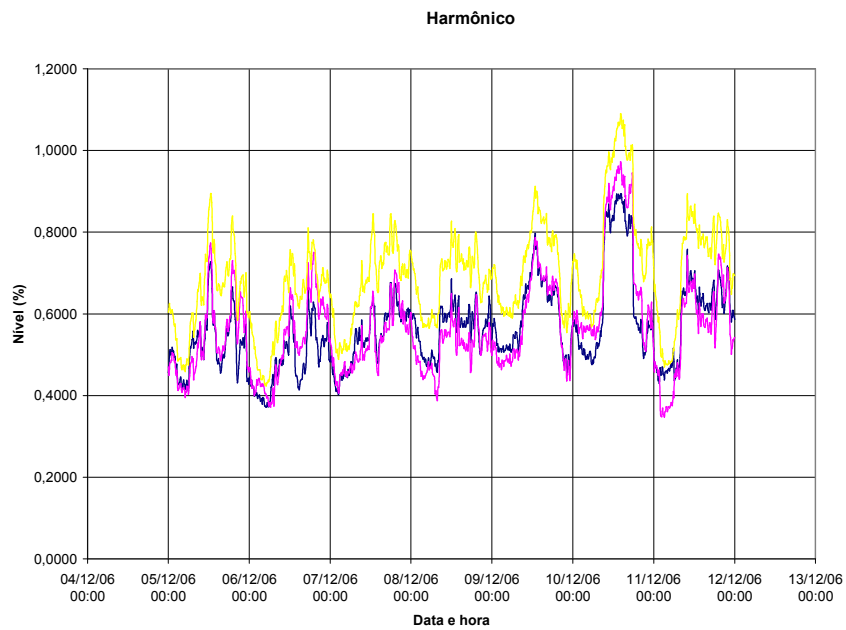
Figura A.32 – Distorção harmônica total de tensão por fase – TPI (cabo comum)
