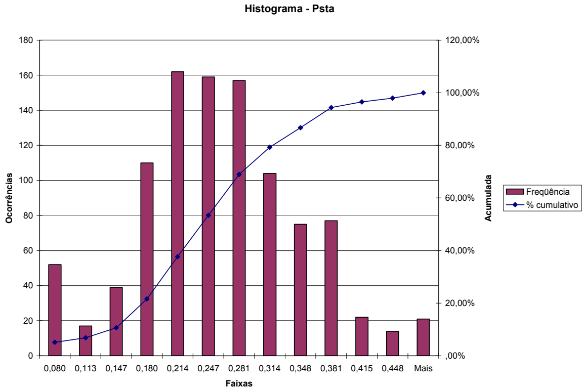
Figura A.13 – Histograma para P_{st} na fase A – TPI (cabo blindado)
