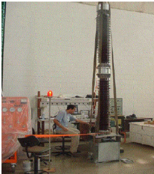
Figura 3.3 – Transformador de Potencial Capacitivo
