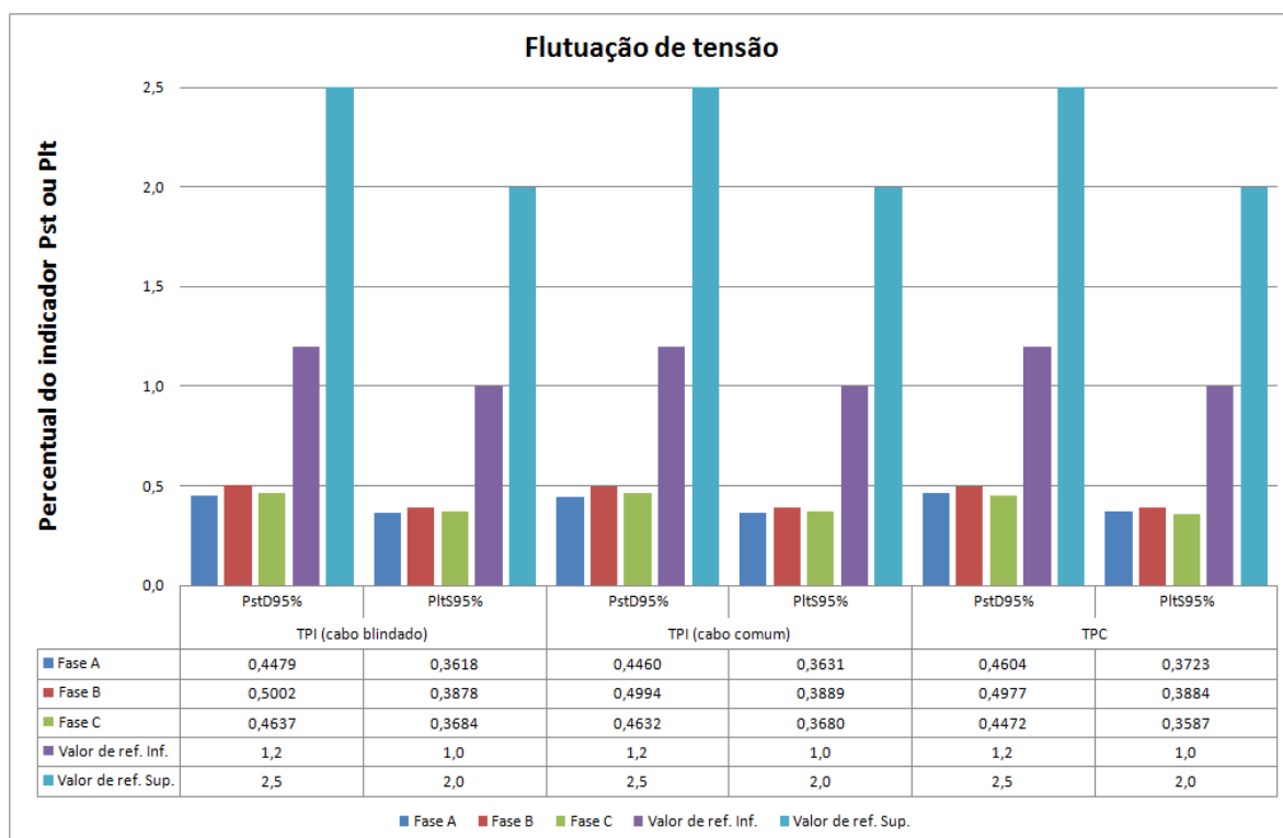
Figura 4.15 – Resultado da medição de flutuação de tensão na SE PAL 10
