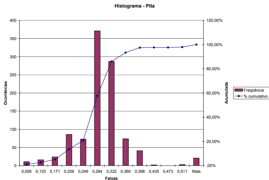
Figura 4.11 – Histograma para Plt na fase A – TPC
