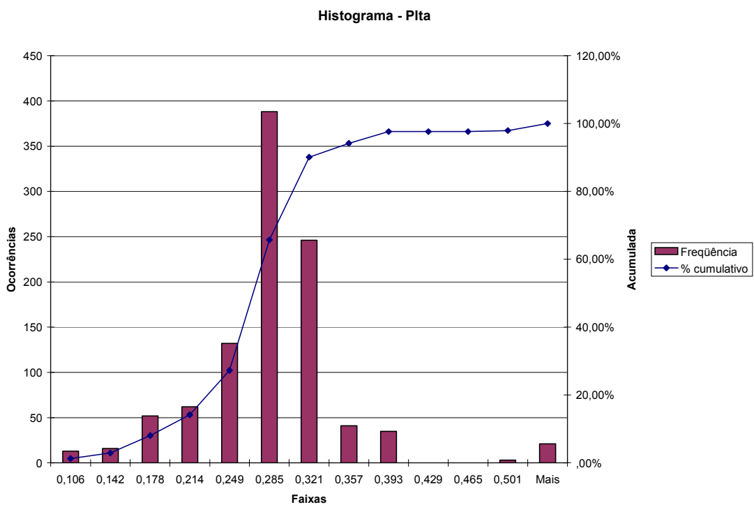
Figura A.22 – Histograma para P_{lt} na fase A – TPI (cabo comum)
