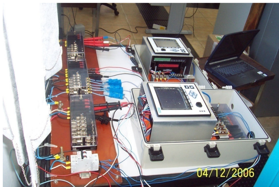
Figura 4.5 – Medidores instalados na SE PAL 10 para a medição realizada
