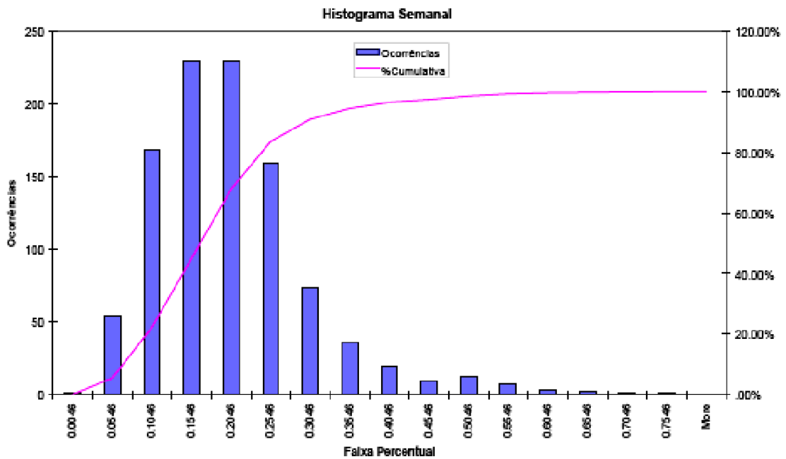
Figura 3.16 – Exemplo de histograma do indicador K durante os sete dias de medição
