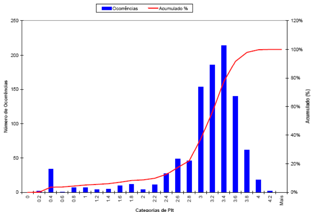
Figura 3.23 – Exemplo de histogramas com valores de Plt medidos na fase A de uma medição hipotética ao longo de uma semana
