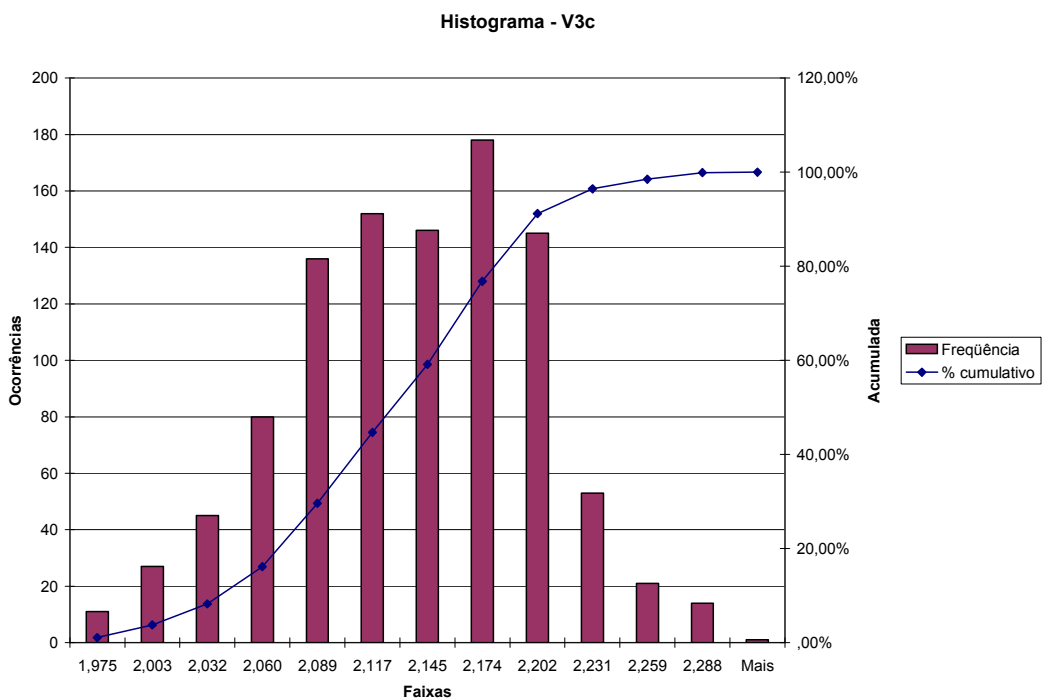
Figura A.60 – Distorção para o 3º harmônico de tensão na fase C – TPC
