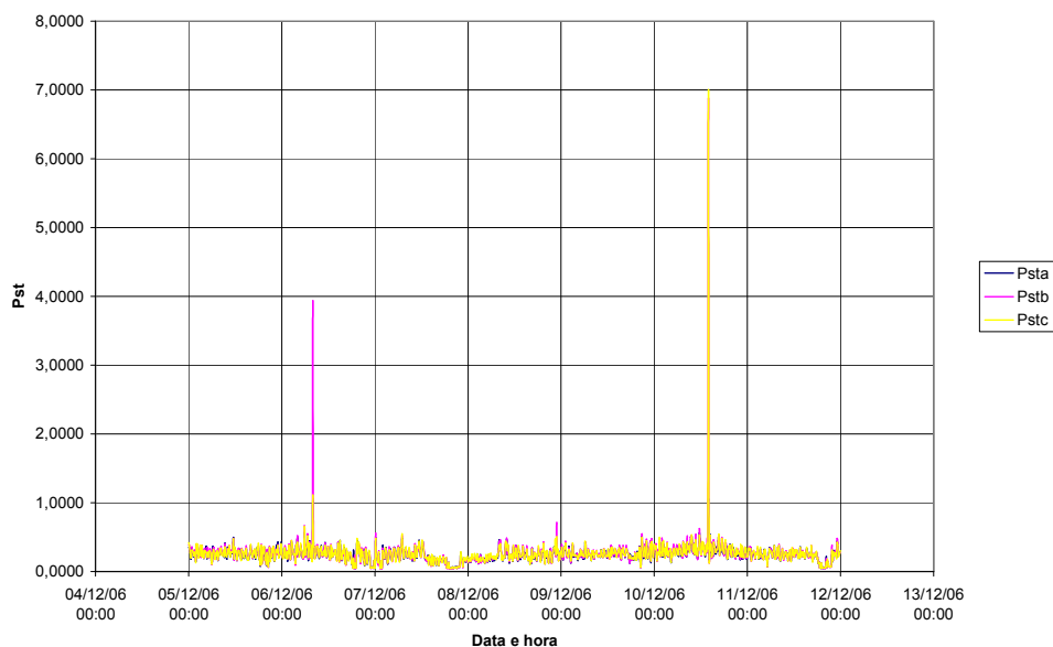
Figura A.7 – Pst por fase – TPI (cabo blindado)
