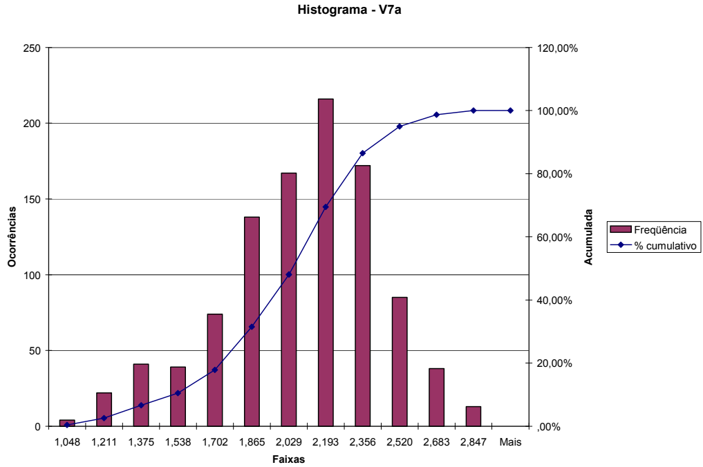
Figura A.61 –Distorção para o 7º harmônico de tensão na fase A – TPC
