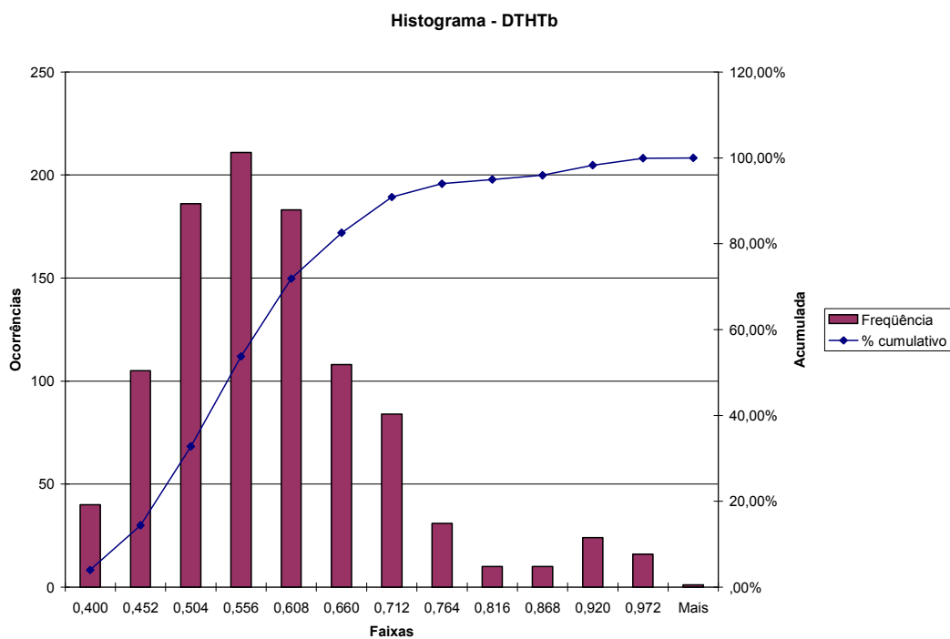
Figura A.44 – Distorção harmônica total de tensão na fase B – TPI (cabo comum)
