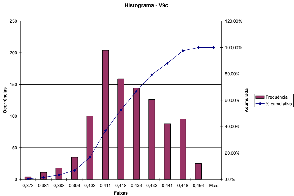
Figura A.66 – Distorção para o 9º harmônico de tensão na fase C – TPC
