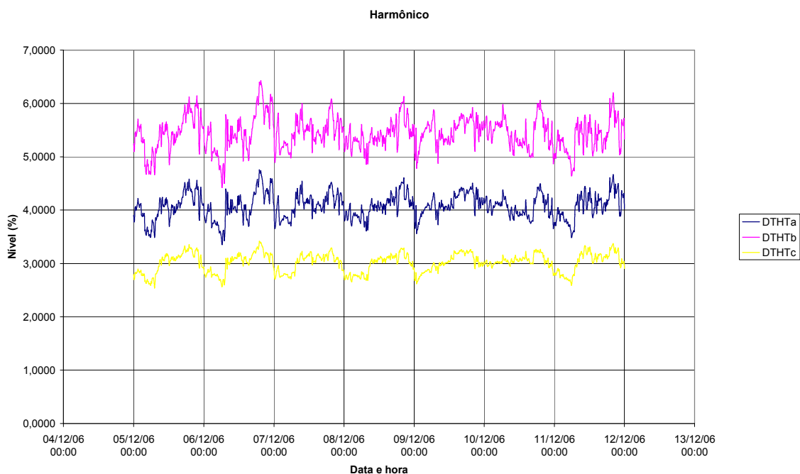
Figura 4.12 – Distorção harmônica total de tensão por fase – TPC
