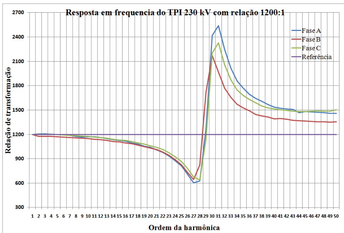
Figura 4.1 – Curvas de resposta em frequência do TPI com relação 1200:1 e cabo com blindagem até o medidor
