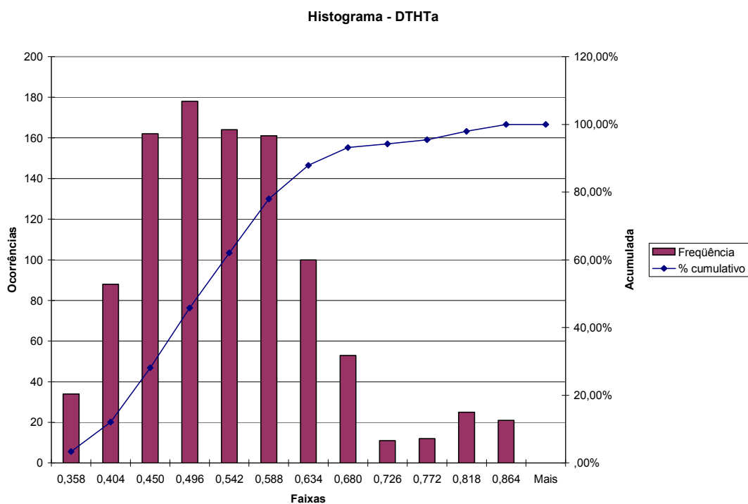
Figura A.40 – Distorção harmônica total de tensão na fase A – TPI (cabo blindado)
