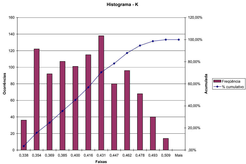
Figura A.5 – Histograma para o desequilíbrio de tensão – TPI (cabo comum)
