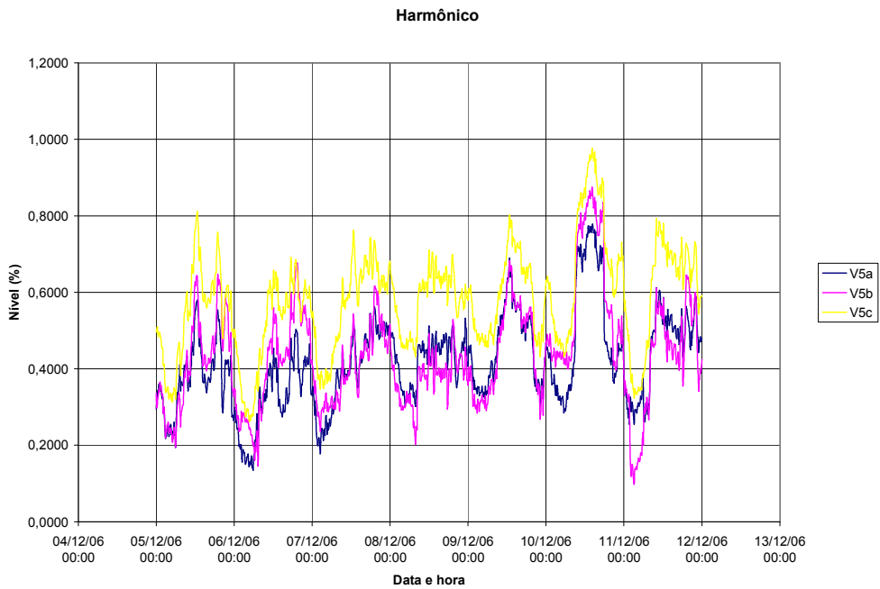
Figura A.35 – Distorção para o 5º harmônico de tensão por fase – TPI (cabo comum)
