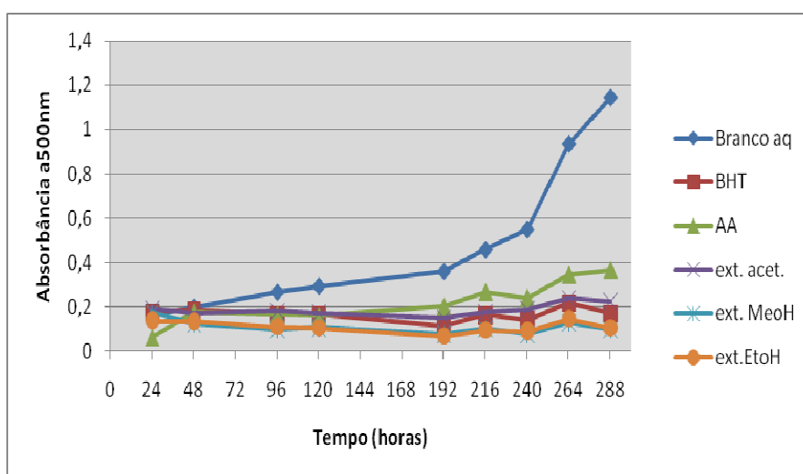
FIGURA 1. Atividade antioxidante de extratos de resíduo agroindustrial de acerola, BHT e ácido ascórbico (125ppm) pelo método tiocianato férrico.
