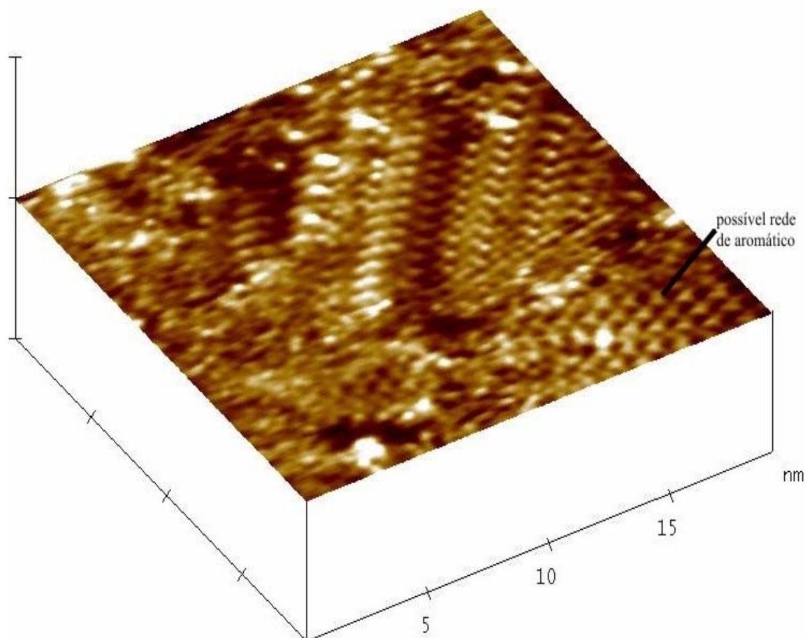
Figura 25 - Imagem de STM (AC) da organização do coroneno sobre a superfície estudada.
