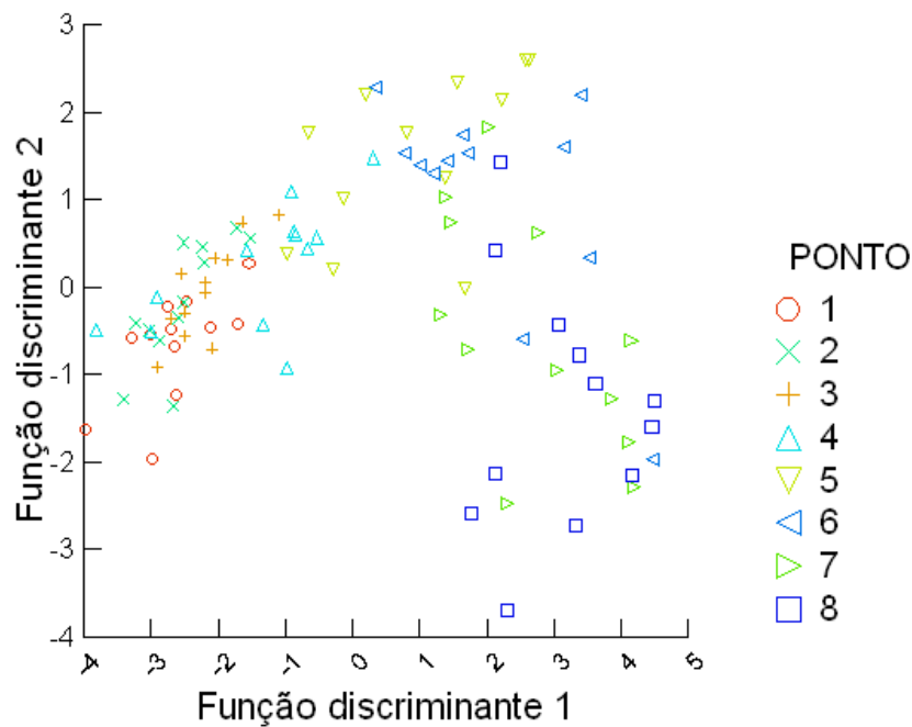
Figura 34 – Análise discriminante classificando os pontos de coleta com base nos macroinvertebrados bentônicos da Vila do Abraão, Ilha Grande, RJ, coletado com o Surber .
