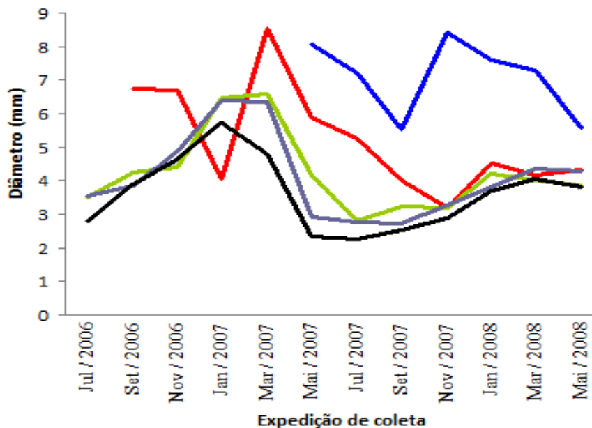
Figura 15 – Variação do diâmetro dos indivíduos de M. tuberculatus (Müller, 1774) da Vila do Abraão, Ilha Grande, RJ; em cada um dos oito pontos de coleta estudados. P4 – azul, P5 – vermelho, P6 – verde, P7 – roxo e P8 – preto.
