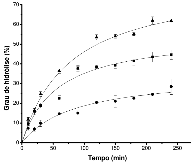
Figura 2 – Grau de hidrólise dos hidrolisados protéicos de peixe (■ HPP com R^2 = 0.97708 ), (HPP 100 , R^2 = 0.95775 ) (▲ HPP 600 R^2 = 0.98462 ).
