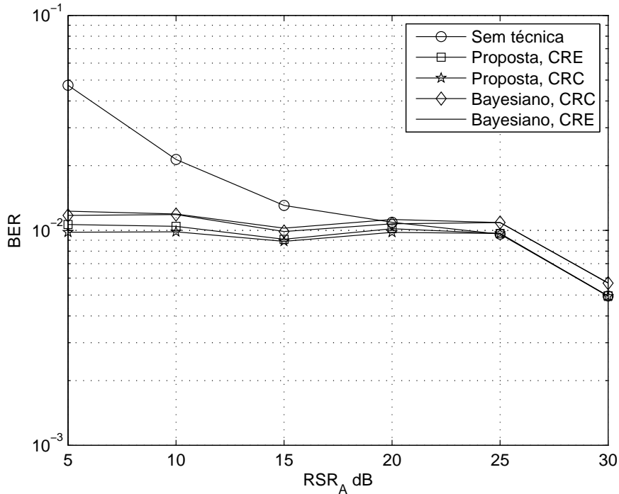
FIG. 4.6: Taxa de erro de bit da Estratégia I em função da RSR_A nas condições: PEM = 10^{-2} e RSR_R = 10 dB.
