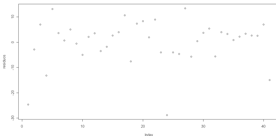
Figura 5. Gráfico do comportamento resíduos obtidos do modelo.
