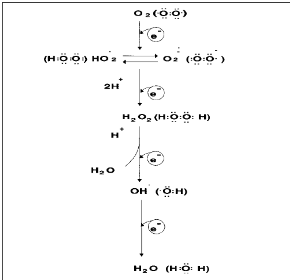
Figura 8: Redução tetraivalente do oxigênio molecular ( \text{O}_2 ) na mitocôndria até a formação de água ( \text{H}_2\text{O} ). Várias espécies reativas de \text{O}_2 são formadas no processo (FERREIRA; MATSUBARA, 1997).
