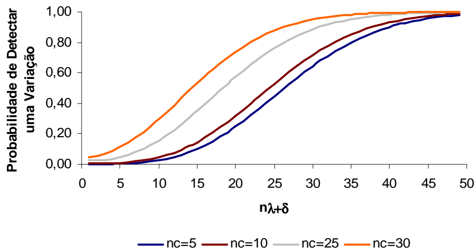
Figura 5.1 Probabilidade de Rejeição do Gráfico de Controle para Processos Poisson.
