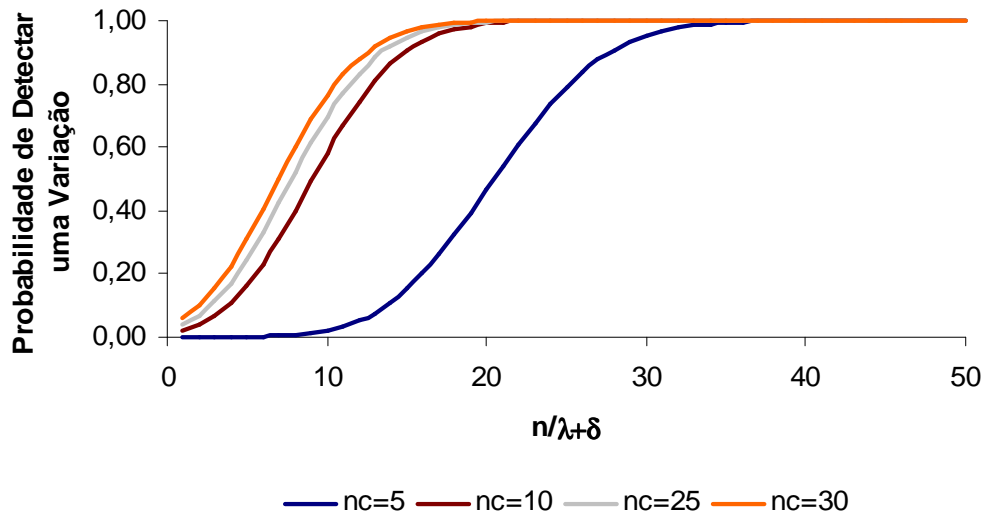
Figura 5.2 Probabilidade de Rejeição do Gráfico de Controle para Processos Exponenciais.
