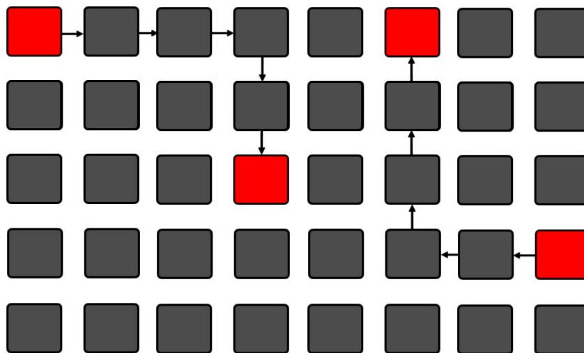
Figura 3.8. Algoritmo XY
