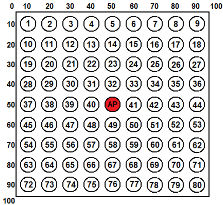
Figura 4.5. Área de simulação da rede plana com 80 nós sensores e AP no centro
