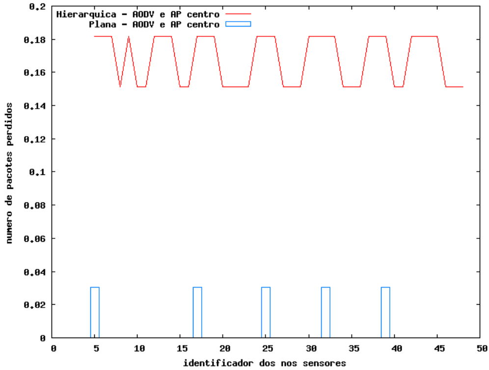
Figura 5.47. Número de pacotes perdidos da rede plana e da rede hierárquica com 48 nós sensores, protocolo de roteamento AODV e AP no centro – Rede plana foi superior
