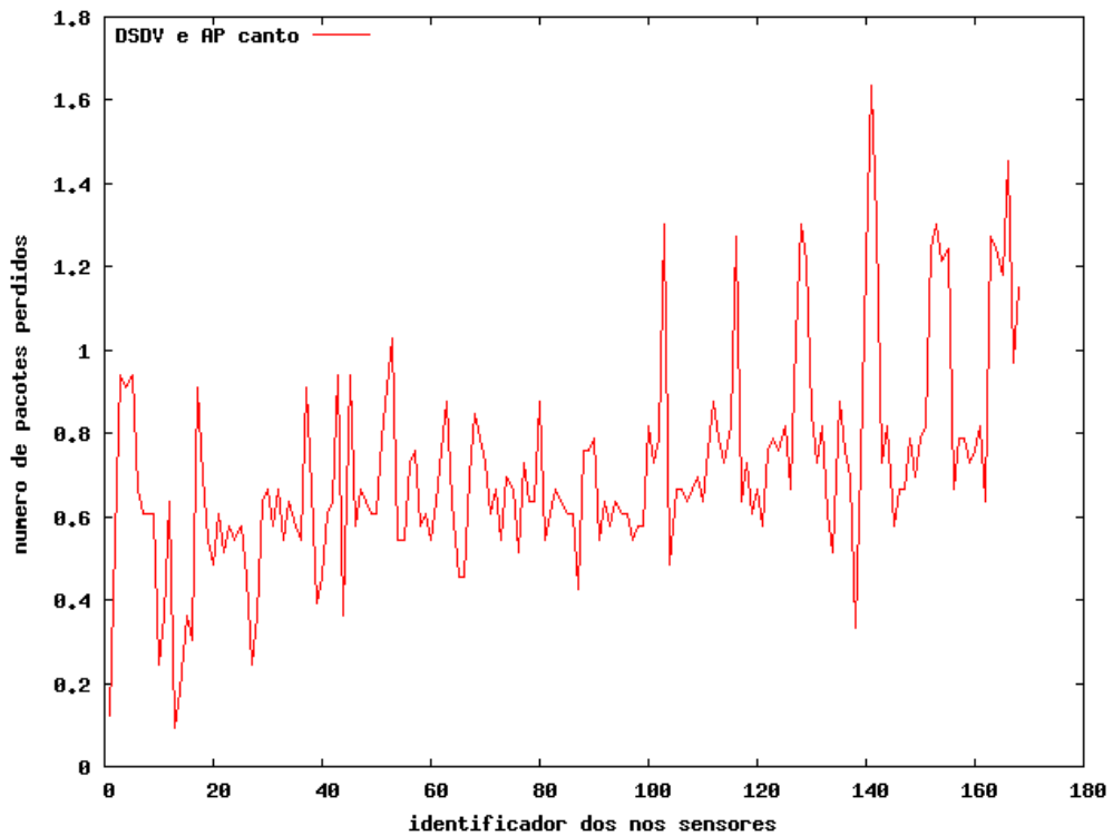
Figura 5.24. Número de pacotes perdidos na área com 168 nós sensores, protocolo de roteamento DSDV e AP no canto
