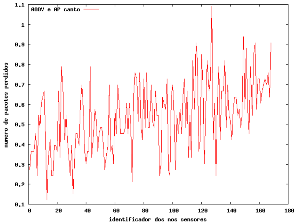
Figura 5.22. Número de pacotes perdidos na área com 168 nós sensores, protocolo de roteamento AODV e AP no canto – Nós sensores mais distantes do AP tiveram maior perda de pacotes
