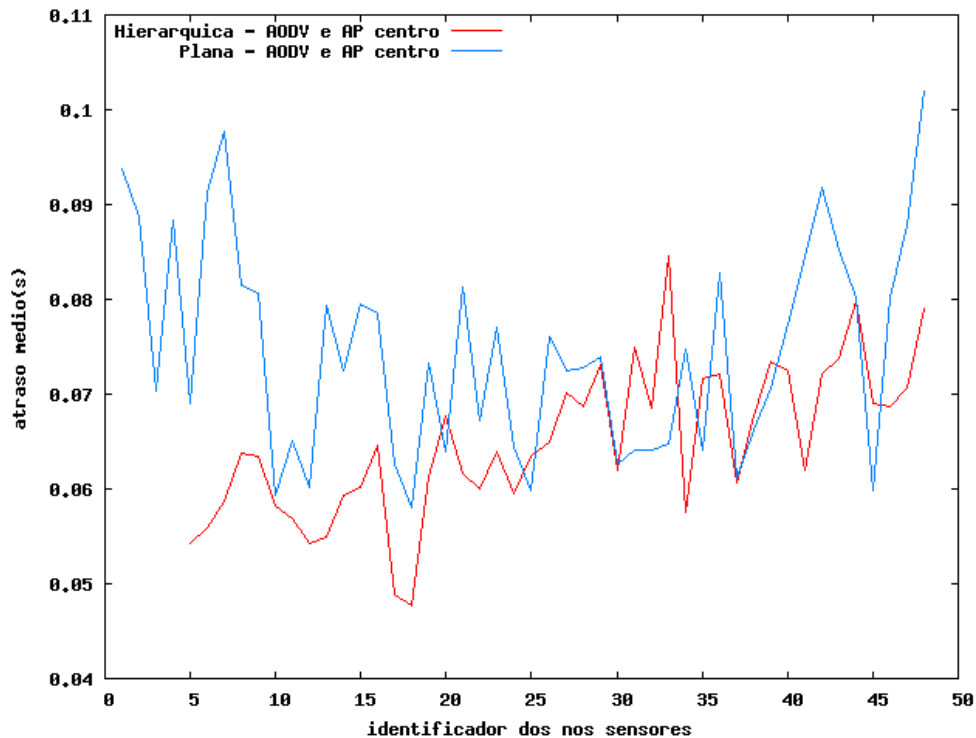
Figura 5.35. Atraso médio da rede plana e da rede hierárquica com 48 nós sensores, protocolo de roteamento AODV e AP no centro
