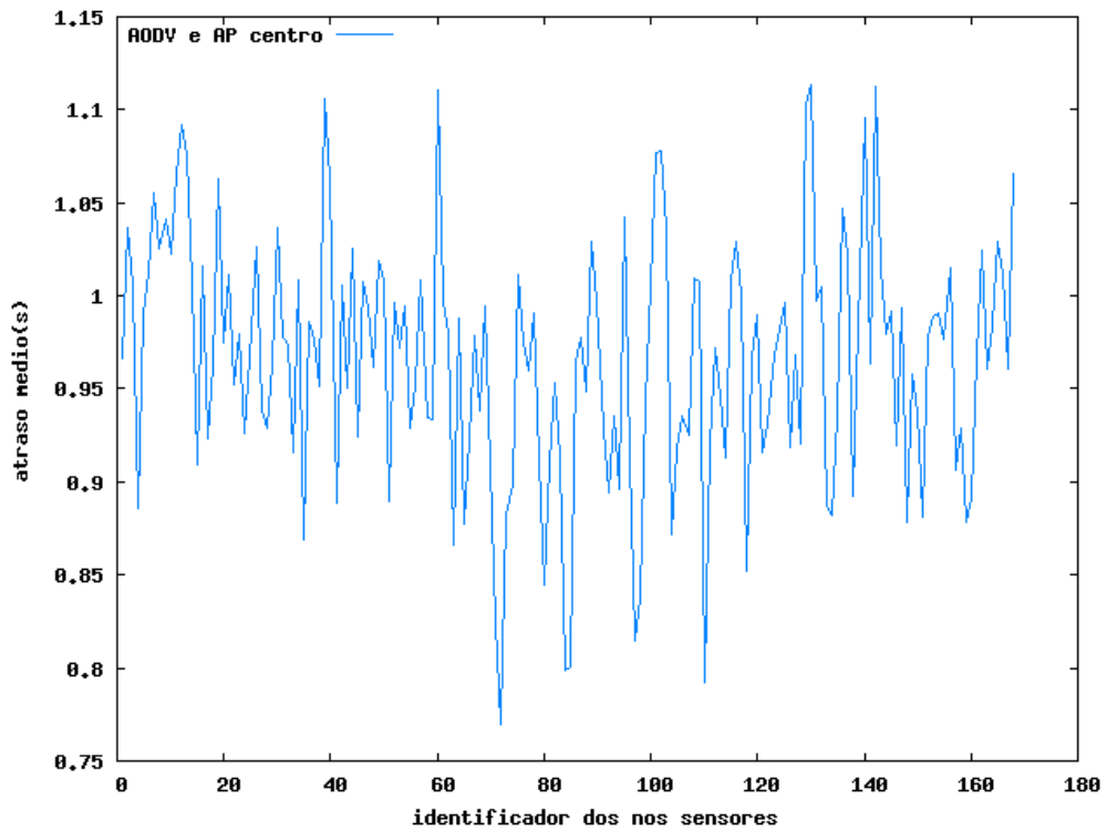
Figura 5.7. Atraso médio da rede plana com 168 nós sensores, protocolo de roteamento AODV e AP no centro
