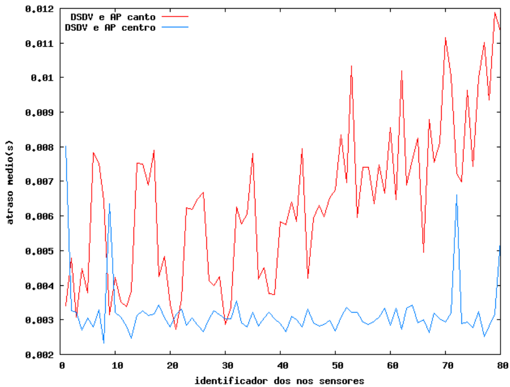
Figura 5.5. Atraso médio da rede plana com 80 nós sensores, protocolo de roteamento DSDV e AP no canto e no centro
