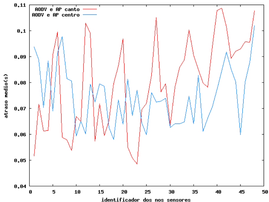
Figura 5.1. Atraso médio da rede plana com 48 nós sensores, protocolo de roteamento AODV e AP no canto e no centro
