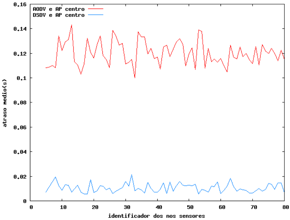
Figura 5.27. Atraso médio da rede hierárquica com 76 nós sensores comuns, 4 cluster-heads, protocolos de roteamento AODV e DSDV e AP no centro
