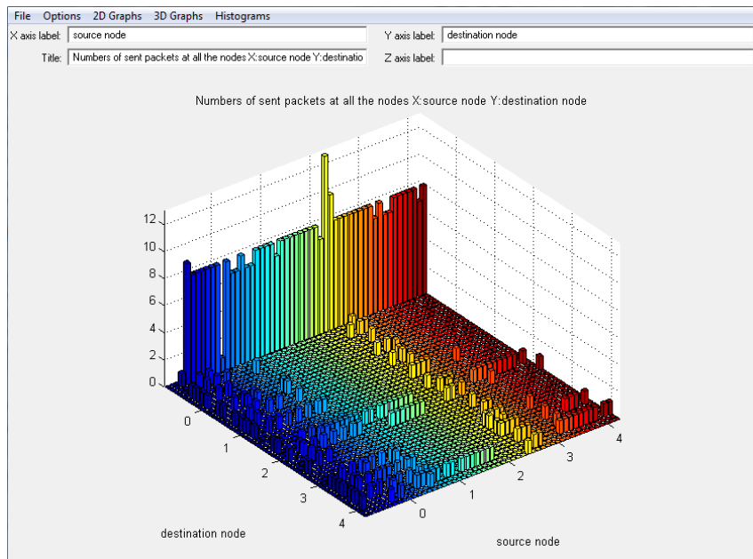
Figura 3.3. Ferramenta de geração de gráficos TraceGraph
