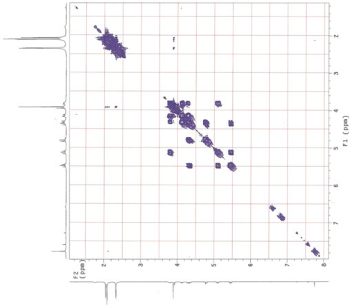
Figura 27- Espectro de COSY ^1\text{H} \times ^1\text{H} (300 MHz, \text{CDCl}_3 ) de \text{S}_5
