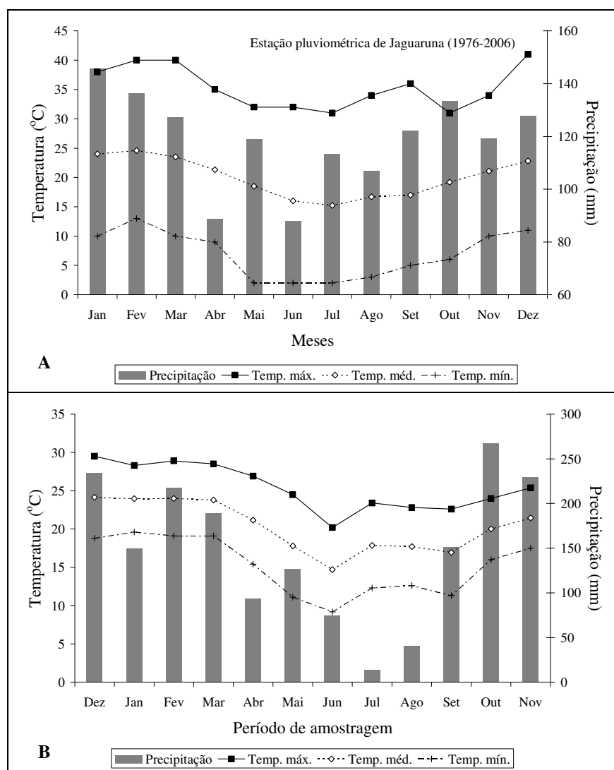
Figura 2. (A) Índices médios mensais de precipitação (mm) obtidos através da série histórica (1976 – 2006) registrada pela Estação Pluviométrica de Jaguaruna (UTM/SAD69 694374 E, 6828598 N); (B) Dados de precipitação pluviométrica (mm) e temperaturas máximas, médias e mínimas (°C) para o período de estudo registrado pela Estação Meteorológica de Urussanga, Urussanga, Santa Catarina.
